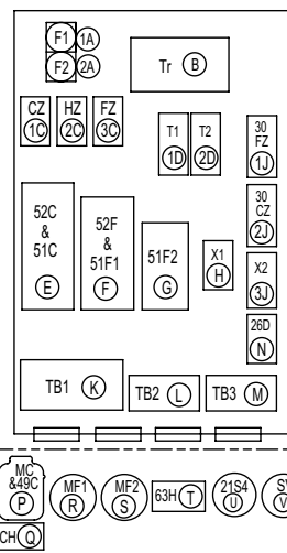
Рис 1. ПАНЕЛЬ УПРАВЛЕНИЯ: РАСПОЛОЖЕНИЕ ЭЛЕМЕНТОВ
