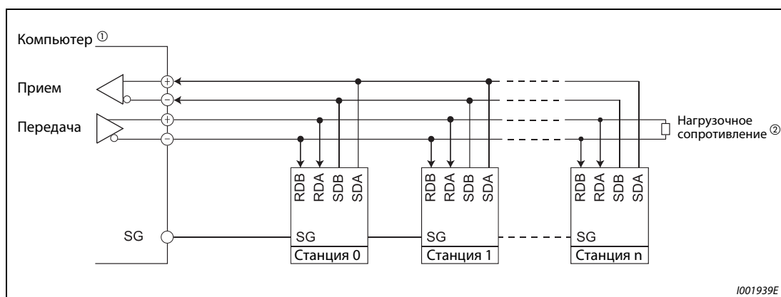
Рис. 6-114: Соединение с несколькими преобразователями частоты
