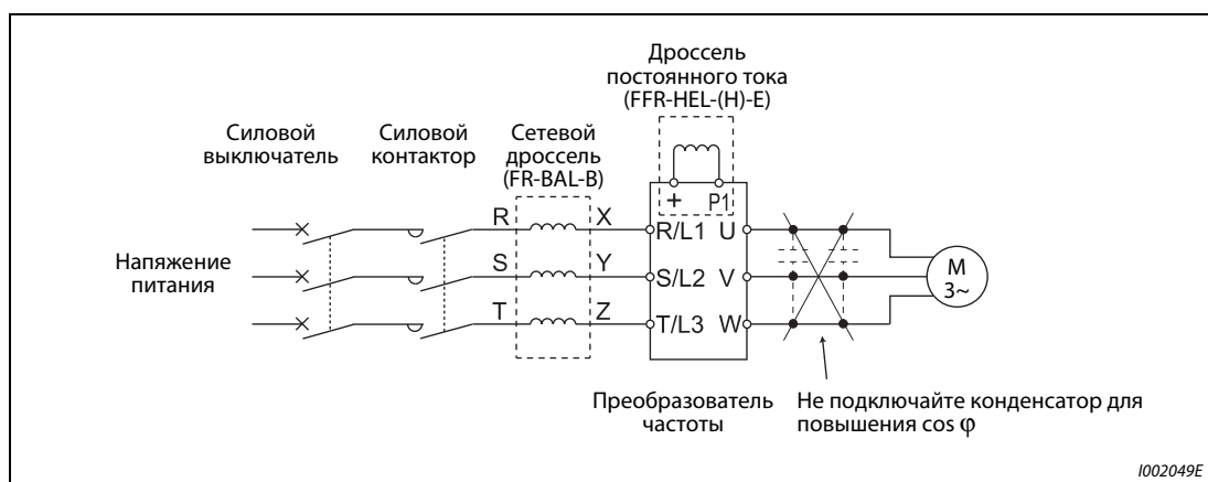
Рис. 3-34: Подавление высокочастотных гармоник в напряжении сети
