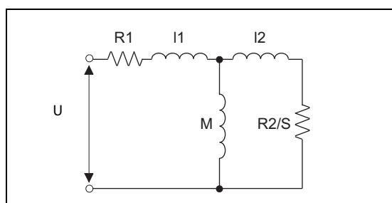
Рис. 6-40: Схема замещения электродвигателя
