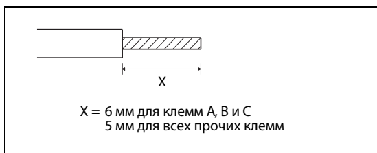
Рис. 3-7: Подготовка кабеля
