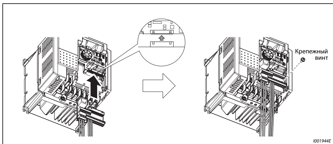
Рис. 8-8: Установка клеммного блока
