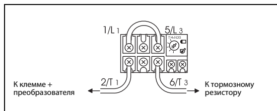
Рис. 3-22: Подключение Термореле
