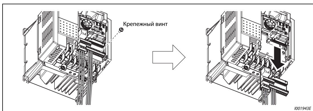
Рис. 8-7: Снятие клеммного блока
