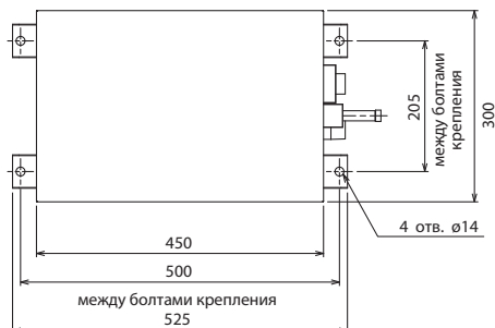
Вид сверху
