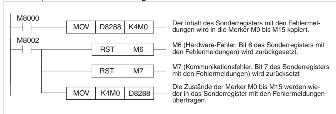
Abb. 11-17: Beispiel zum Zurücksetzen der Fehlermeldungen des FX3U-4AD-PTW-ADP, das als 3. analoges Adaptermodul (1. Modul bei FX3G) installiert ist.
