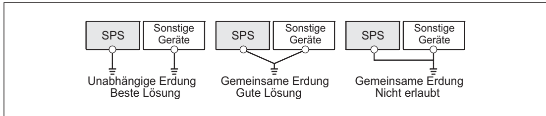
Abb. 11-9: Erdung der SPS
