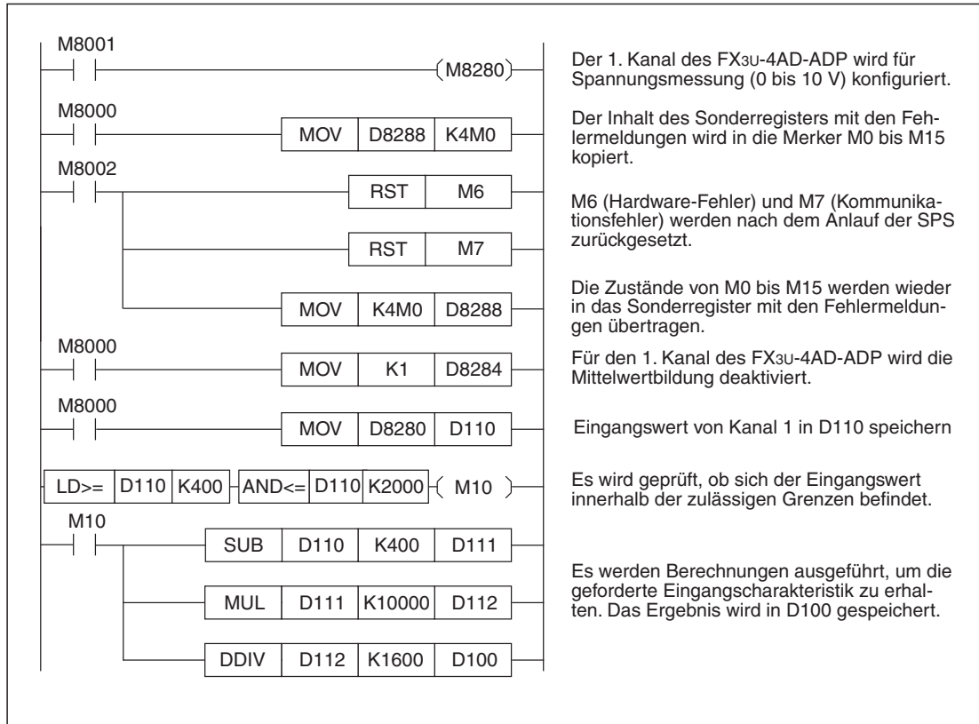
Abb. 4-25: Programmbeispiel zur Änderung der Charakteristik eines Spannungseingangs
