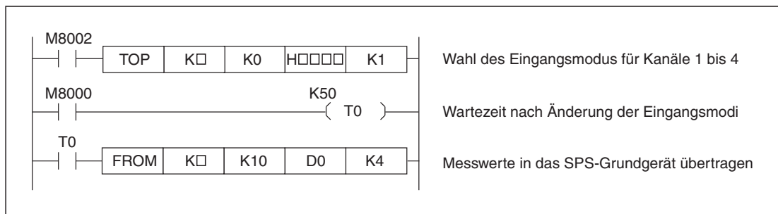
Abb. 5-28: Minimal-Programm zum Einstellen eines Analogeingangsmoduls FX3U-4AD/FX3UC-4AD und zum Lesen der Messwerte
