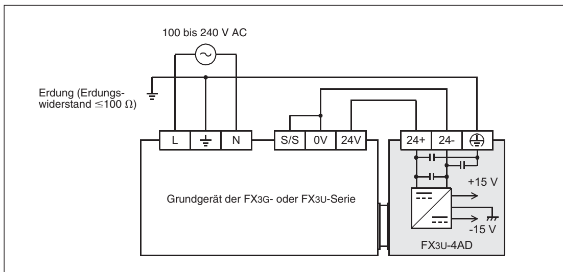
Abb. 5-14: Versorgung durch ein SPS-Grundgerät, das für plusschaltende Geber konfiguriert ist (Der Anschluss „S/S“ ist mit dem Anschluss „0V“ verbunden.)
