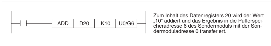
Abb. A-3: Anwendung des direkten Pufferspeicherzugriff bei einer Addition
