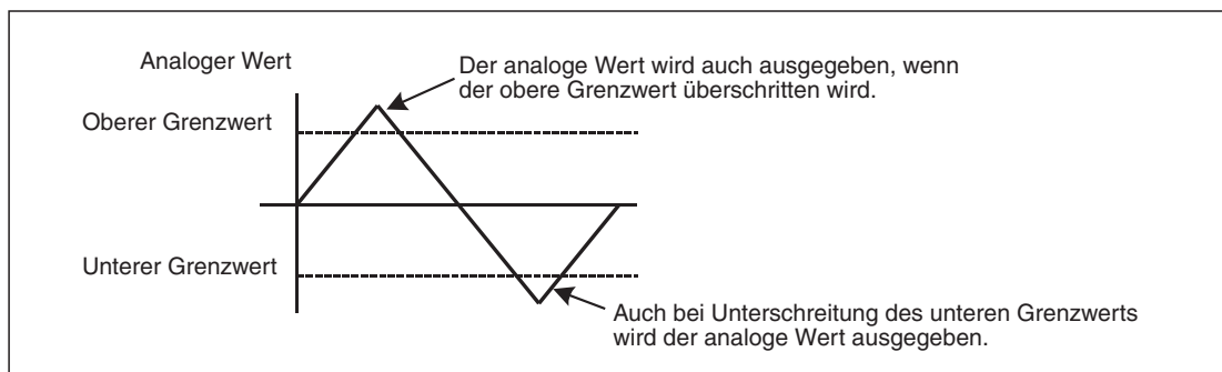
Abb. 8-20: Die Ausgabe des Analogwerts wird durch eine Grenzwertüberschreitung nicht beeinflusst.
