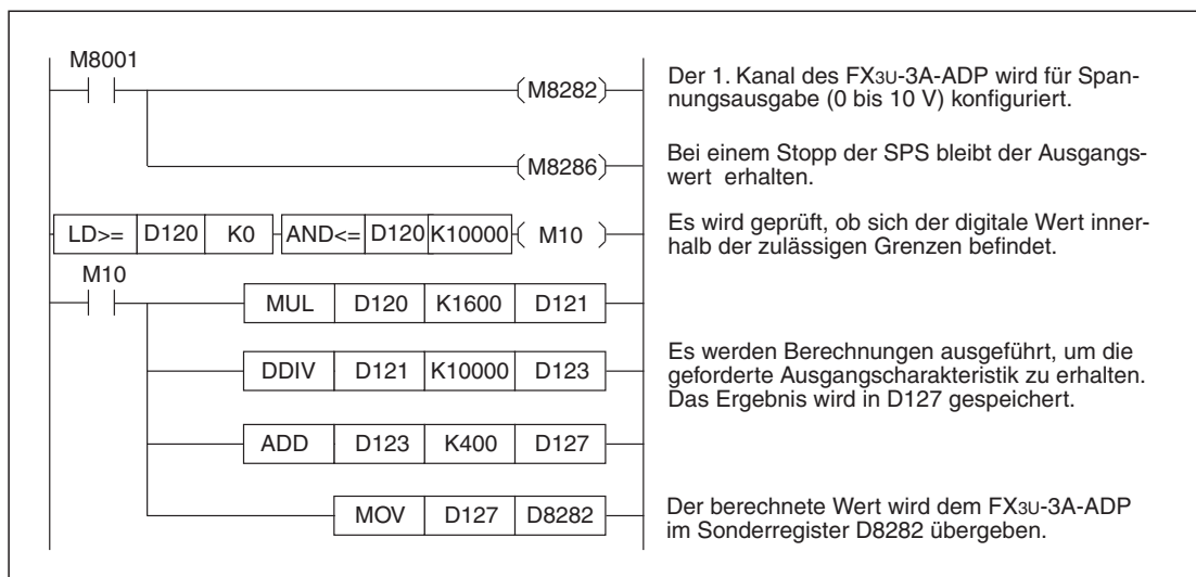
Abb. 9-33: Programmbeispiel zur Änderung der Charakteristik des Spannungsausgangs
