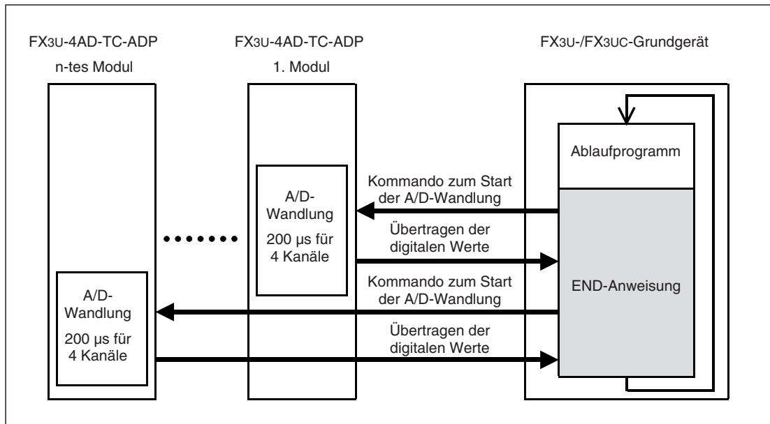
Abb. 13-2: Prinzip der Messwerterfassung bei FX3U- und FX3UC-Grundgeräten
