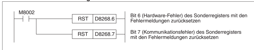
Abb. 12-20: Beispiel zum Zurücksetzen der Fehlermeldungen des FX3U-4AD-PNK-ADP, das als 1. analoges Adaptermodul installiert ist.
