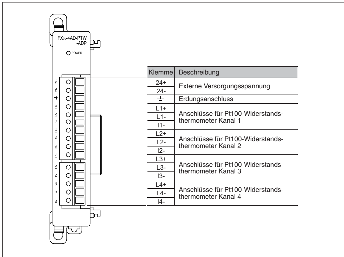
Abb. 11-5: Klemmenbelegung des FX3U-4AD-PTW-ADP
