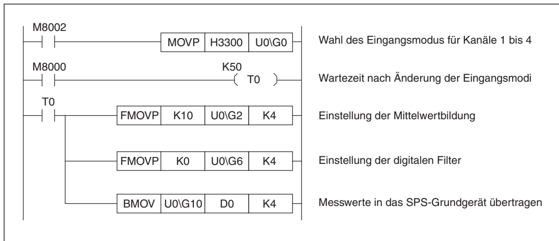
Abb. 5-31: Beispielprogramm mit direktem Speicherzugriff zur Konfiguration der Mittelwertbildung und der digitalen Filter
