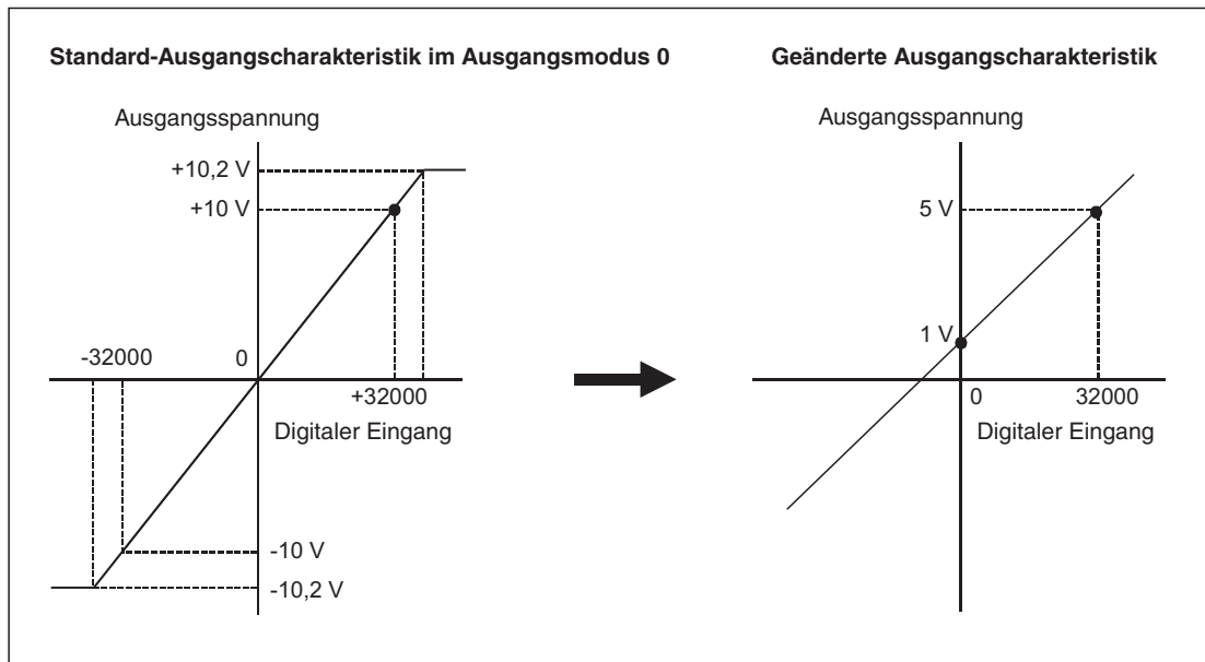
Abb. 8-34: Die Standard-Ausgangscharakteristik für den Ausgangsmodus 0 wird verändert.
