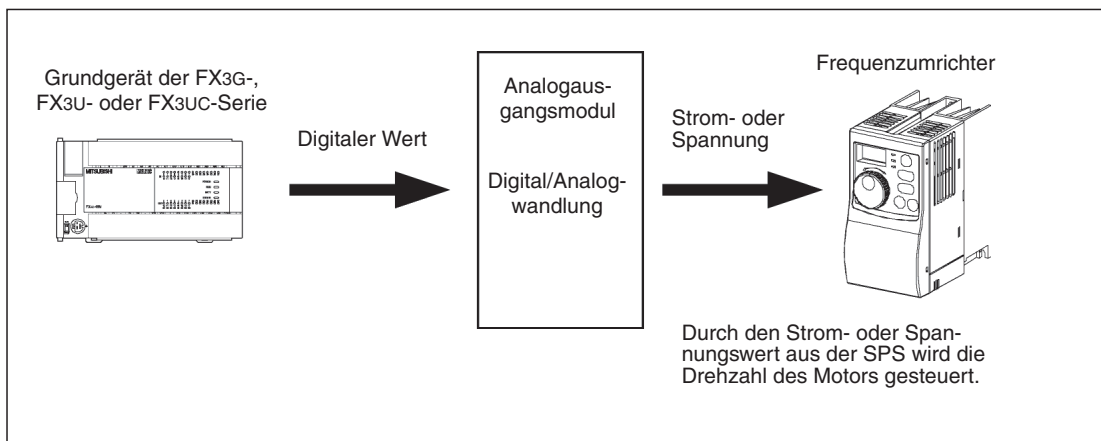
Abb. 1-2: Ausgabe eines analogen Werts: Durch den Strom- oder Spannungswert aus der SPS wird die Drehzahl eines Motors gesteuert.
