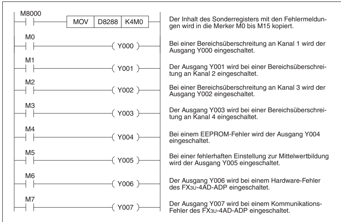
Abb. 4-19: Beispiel zur Auswertung von Fehlermeldungen eines FX3U-4AD-ADP, das als 3. analoges Adaptermodul (1. Modul bei FX3G) installiert ist.
