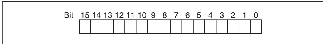
Abb. 5-19: Zuordnung der einzelnen Bit einer Pufferspeicheradresse
