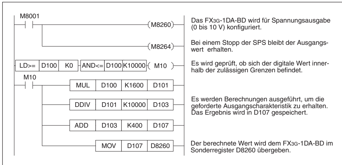
Abb. 6-14: Programmbeispiel zur Änderung der Charakteristik eines Spannungsausgangs
