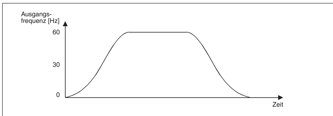
Abb. 8-25: Typische Anwendung eines Frequenzumrichters: Sanftes Beschleunigen und Verzögern des Antriebs
