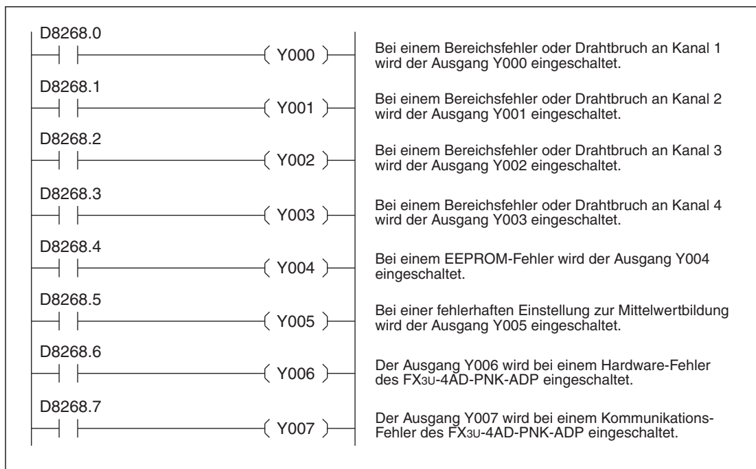
Abb. 12-22: Beispiel zur Auswertung von Fehlermeldungen eines FX3U-4AD-PNK-ADP, das als 1. analoges Adaptermodul installiert ist.
