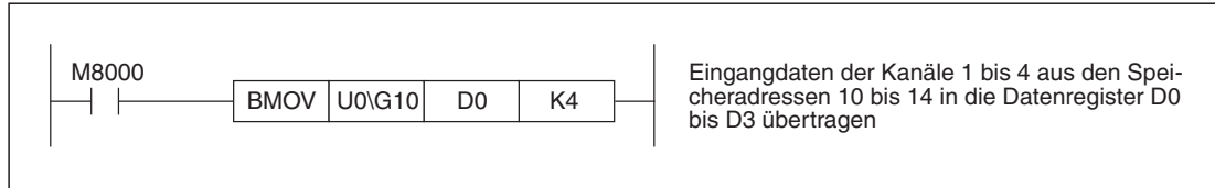
Abb. 5-27: Programmzeile zum Auslesen der Eingangsdaten der Kanäle 1 bis 4
