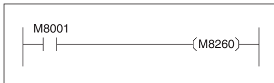
Abb. 3-7: Der 1. Kanal des FX3G-2AD-BD, das auf dem 1. Erweiterungssteckplatz installiert ist, wird für Spannungsmessung konfiguriert. Der Merker M8001 ist immer „0“.
