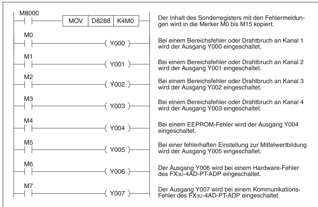
Abb. 10-19: Beispiel zur Auswertung von Fehlermeldungen eines FX3U-4AD-PT-ADP, das als 3. analoges Adaptermodul (1. Modul bei FX3G) installiert ist.
