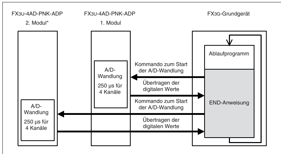
Abb. 12-1: Prinzip der Messwertverarbeitung bei FX3G-Grundgeräten (Maximal können zwei FX3U-4AD-PNK-ADP angeschlossen werden).
