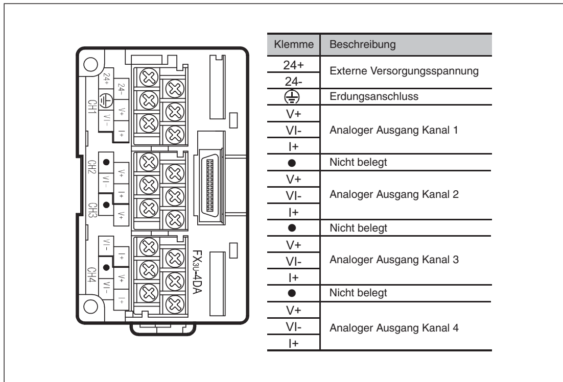
Abb. 8-7: Klemmenbelegung des FX3U-4DA
