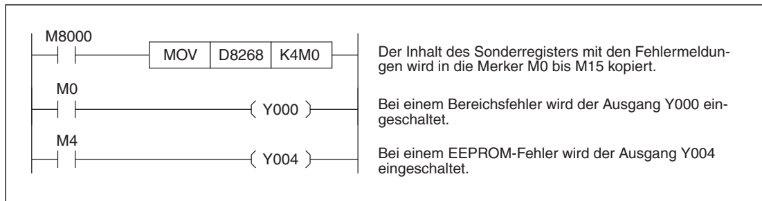
Abb. 6-10: Beispiel zur Auswertung der Fehlermeldungen eines FX3G-1DA-BD, das auf dem 1. Erweiterungssteckplatz installiert ist
