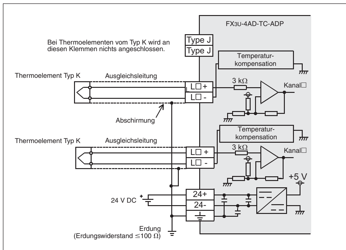
Abb. 13-10: Anschluss von Thermoelementen vom Typ K an ein Temperaturerfassungs-Adaptermodul FX3U-4AD-TC-ADP; die Klemmen „Type J“ werden nicht verdrahtet.
