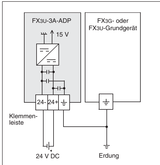
Abb. 9-7: Versorgung des FX3U-3A-ADP aus einer separaten Spannungsquelle
