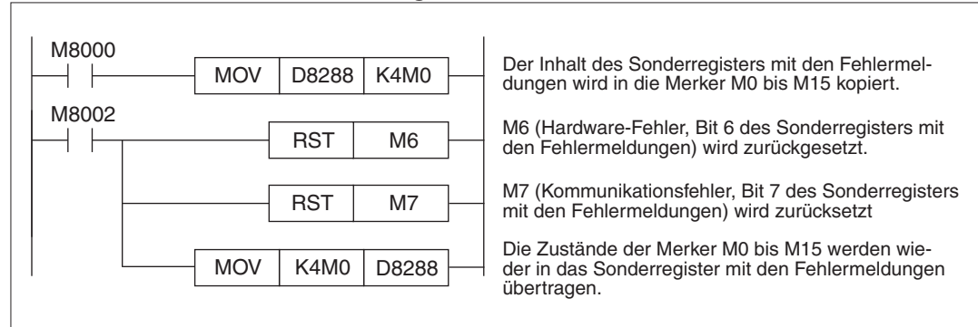
Abb. 9-22: Beispiel zum Zurücksetzen der Fehlermeldungen des FX3U-3A-ADP, das als 3. analoges Adaptermodul (1. Modul bei FX3G) installiert ist.
