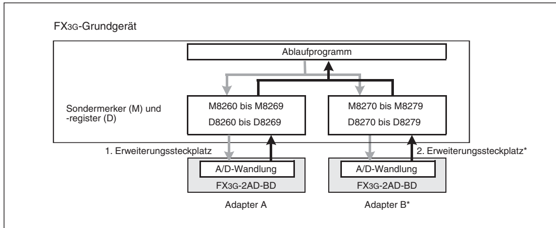
Abb. 3-6: Für jeden analogen Erweiterungsadapter sind 10 Sondermerker und 10 Sonderregister reserviert.
