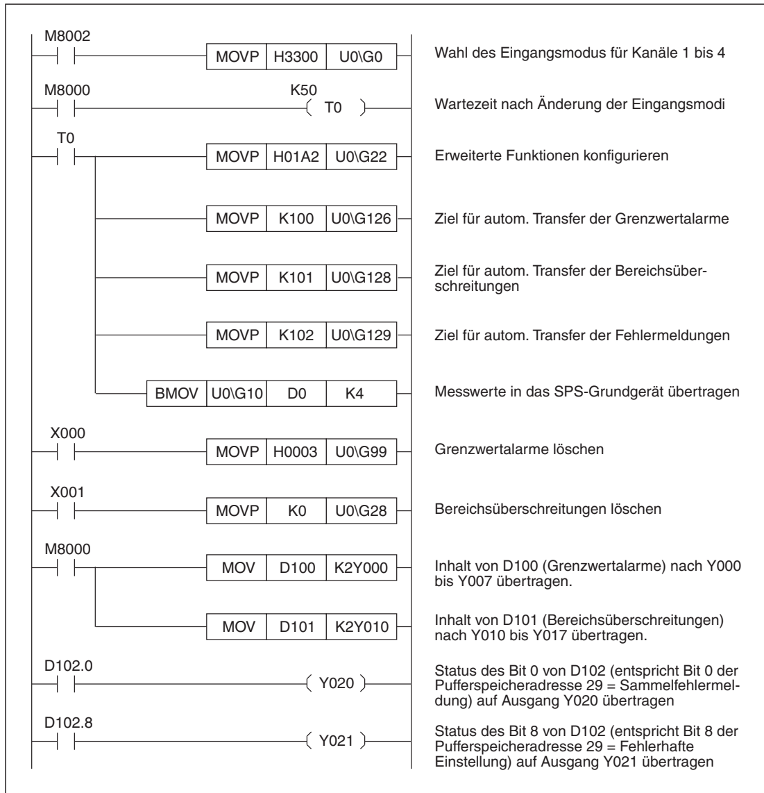
Abb. 5-33: Beispielprogramm mit direktem Speicherzugriff zur Konfiguration erweiterter Funktionen des FX3U-4AD/FX3UC-4AD
