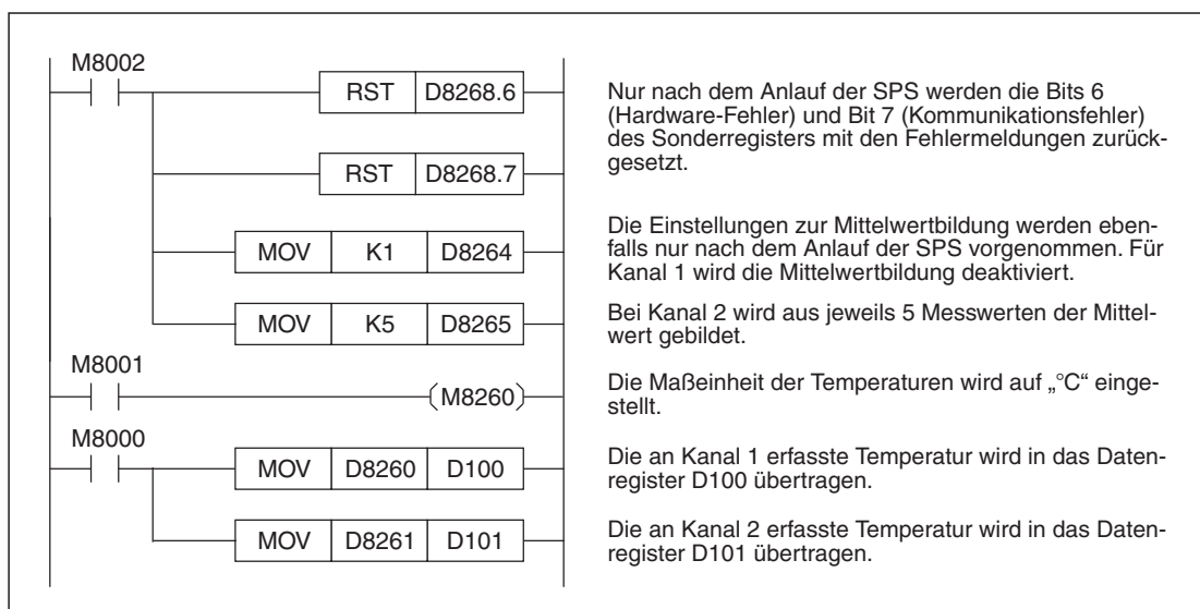
Abb. 10-23: Beispielprogramm zur Konfiguration von Kanal 1 und Kanal 2 eines FX3U-4AD-PT-ADP, das als 1. analoges Adaptermodul installiert ist.
