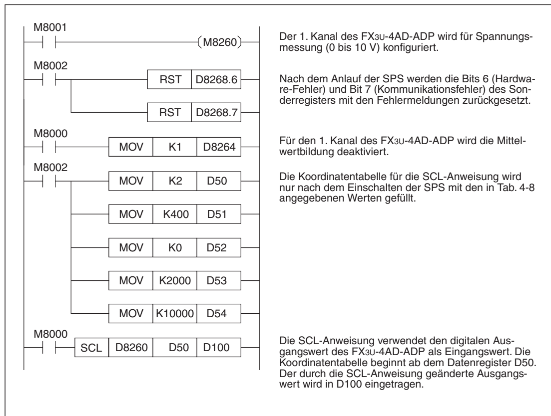
Abb. 4-26: Programmbeispiel zur Änderung der Charakteristik eines Spannungseingangs durch eine SCL-Anweisung
