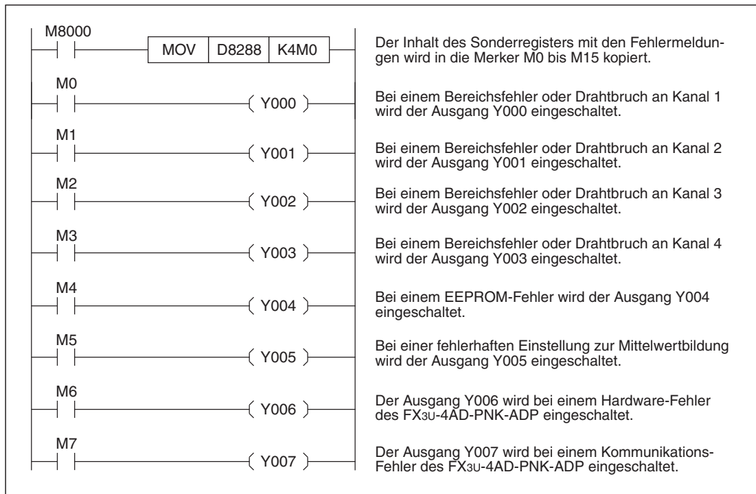
Abb. 12-21: Beispiel zur Auswertung von Fehlermeldungen eines FX3U-4AD-PNK-ADP, das als 3. analoges Adaptermodul (1. Modul bei FX3G) installiert ist.
