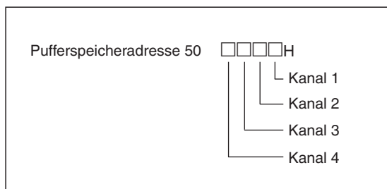
Abb. 8-23: Zuordnung der 4-Bit-Gruppen zu den einzelnen Kanälen
