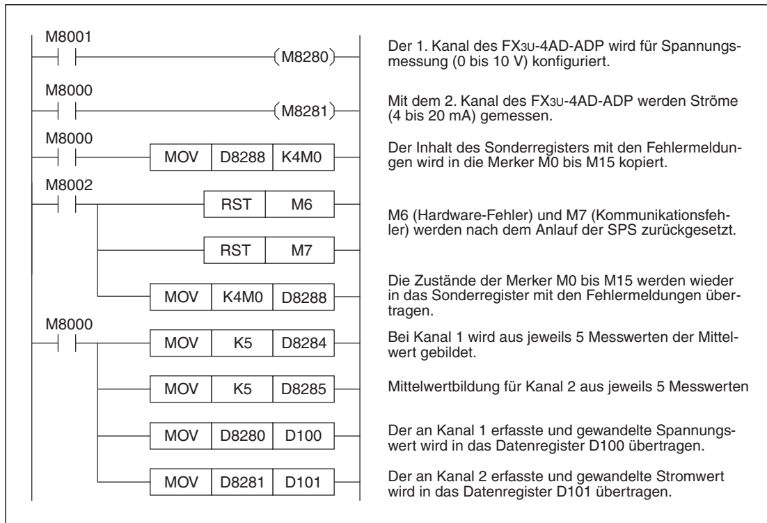
Abb. 4-22: Beispielprogramm zur Konfiguration von Kanal 1 und Kanal 2 eines FX3U-4AD-ADP
