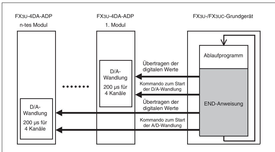
Abb. 7-2: Prinzip der Analogwertausgabe bei FX3U- und FX3UC-Grundgeräten
