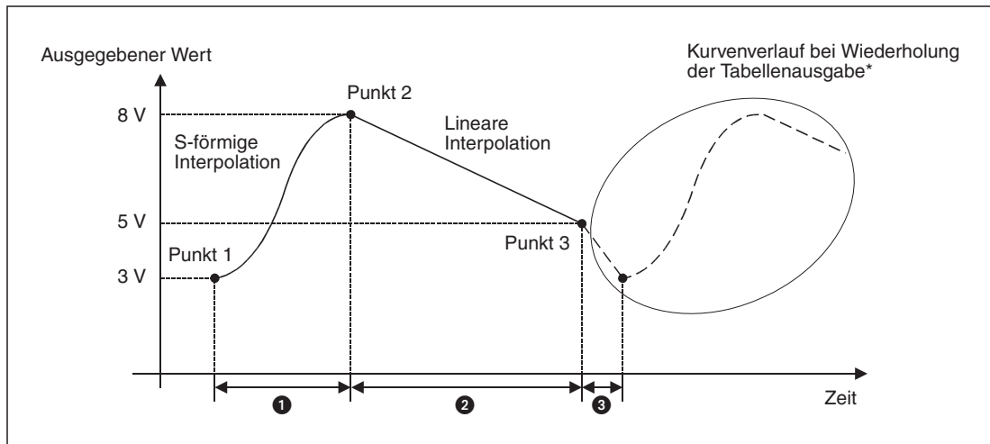
Abb. 8-29: Kurvenverlauf bei Ausgabe von Datensatz 1 im Ausgangsmodus 1
