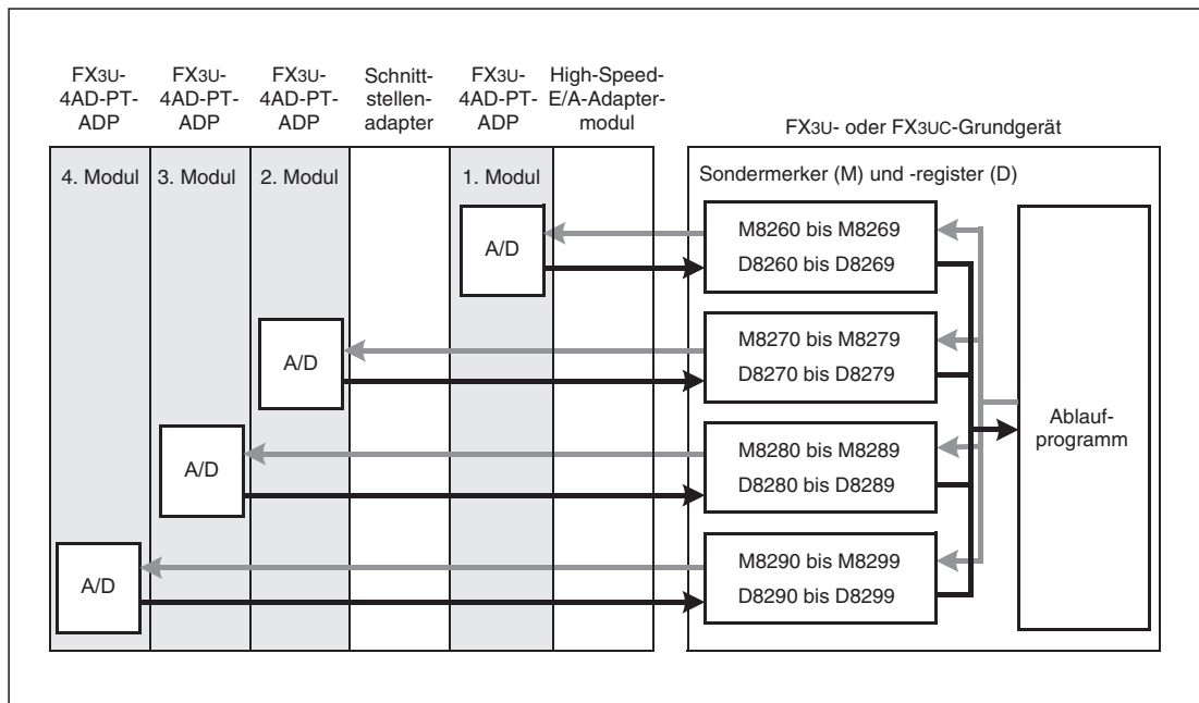
Abb. 10-12: Datenaustausch eines FX3U- oder FX3UC-Grundgeräts mit analogen Adaptermodulen
