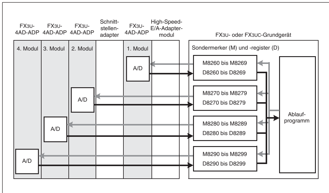
Abb. 4-12: Datenaustausch eines FX3U- oder FX3UC-Grundgeräts mit analogen Adaptermodulen
