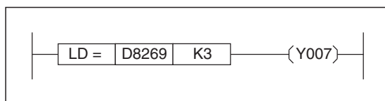
Abb. 6-11: Wenn auf dem 1. Erweiterungssteckplatz ein FX3G-1DA-BD installiert ist, wird der Ausgang Y007 eingeschaltet.
