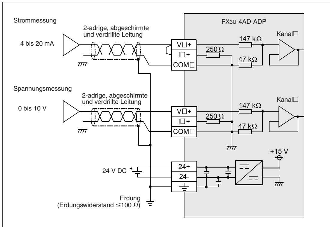
Abb. 4-10: Anschluss der analogen Signale an ein Analogeingangs-Adaptermodul FX3U-4AD-ADP
