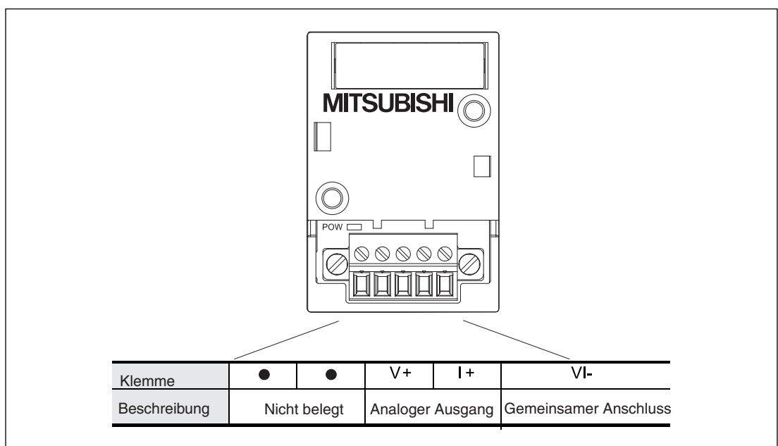
Abb. 6-4: Klemmenbelegung des FX3G-1DA-BD
