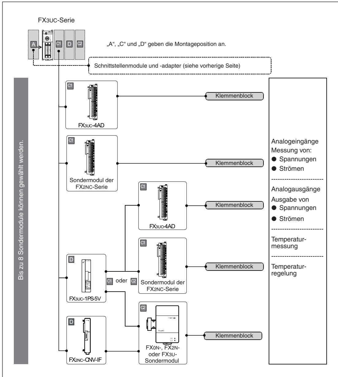
Abb. 1-17: Anschluss von Sondermodulen an ein Grundgerät der FX3UC-Serie
