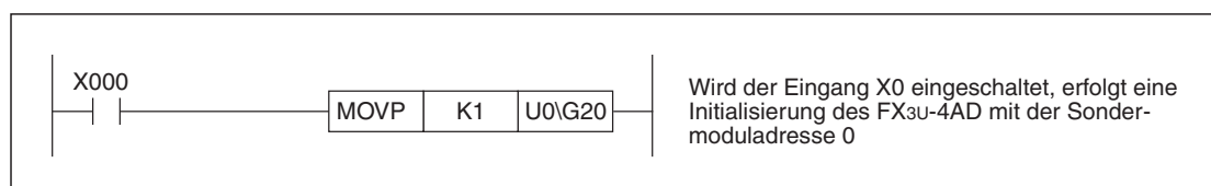
Abb. 5-23: Beispiel für eine Programmsequenz* für ein FX3U- oder FX3UC-Grundgerät zur Initialisierung eines FX3U-4AD/FX3UC-4AD
