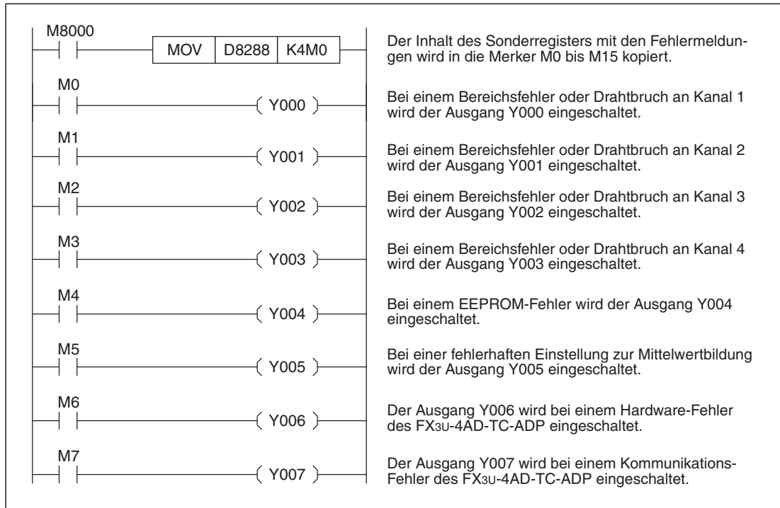
Abb. 13-22: Beispiel zur Auswertung von Fehlermeldungen eines FX3U-4AD-TC-ADP, das als 3. analoges Adaptermodul (1. Modul bei FX3G) installiert ist.
