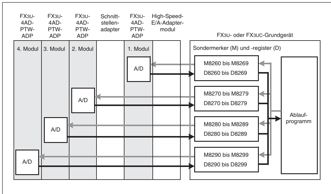
Abb. 11-12: Datenaustausch eines FX3U- oder FX3UC-Grundgeräts mit analogen Adaptermodulen
