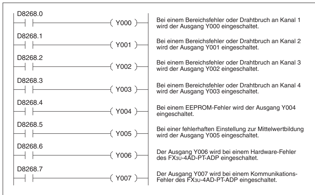
Abb. 10-20: Beispiel zur Auswertung von Fehlermeldungen eines FX3U-4AD-PT-ADP, das als 1. analoges Adaptermodul installiert ist.
