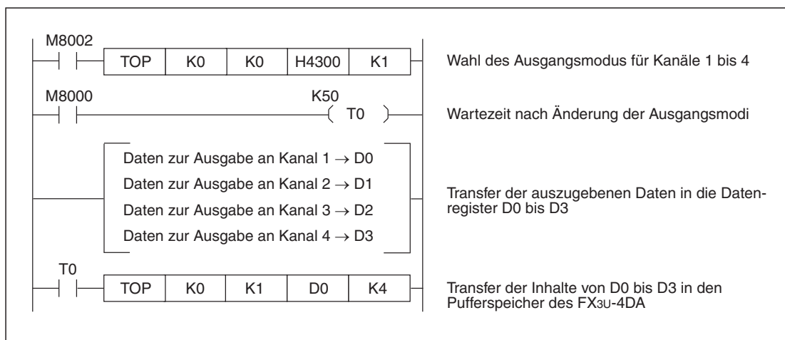
Abb. 8-36: Beispielprogramm zur Einstellung der Ausgangsmodi und der Ausgabe von analogen Werten
