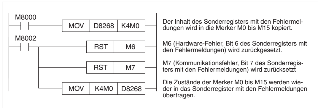
Abb. 3-11: Beispiel zum Zurücksetzen der Fehlermeldungen des FX3G-2AD-BD, das auf dem 1. Erweiterungssteckplatz installiert ist. Der Sondermerker M8002 wird nur im ersten Zyklus nach dem Einschalten der SPS gesetzt.
