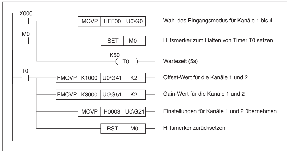
Abb. 5-26: Programmbeispiel zur Änderung der Eingangskarakteristik der Kanäle 1 und 2
