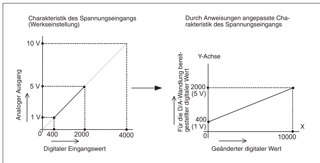
Abb. 7-22: In diesem Beispiel wird durch Anweisungen im Programm der Anfangspunkt und die Steigung einer Geraden verändert.
