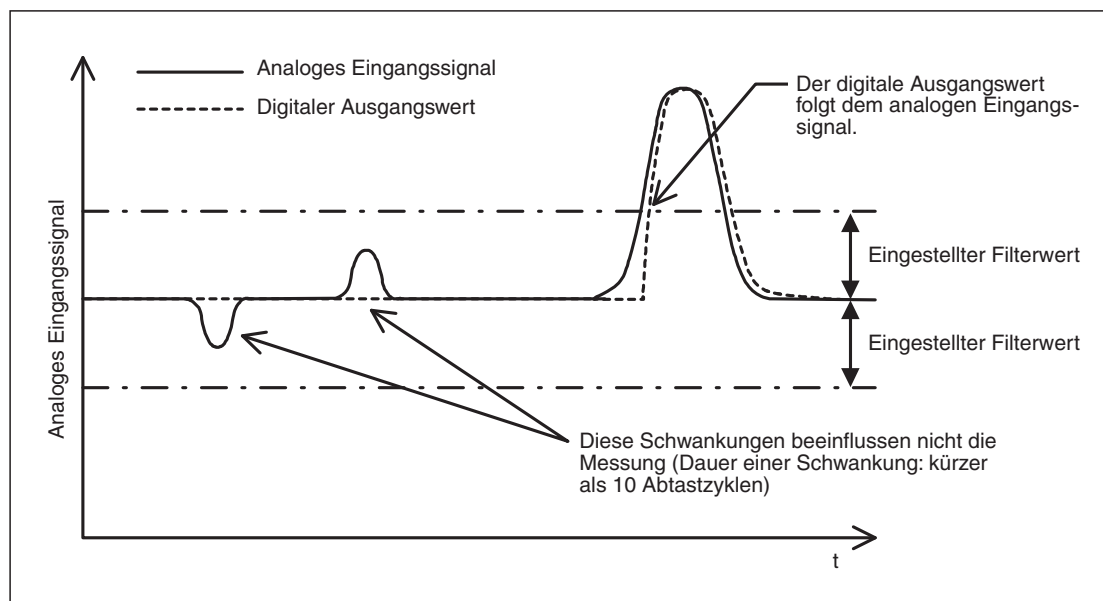
Abb. 5-22: Durch ein digitales Filter können kurzzeitige Störungen des Eingangssignals unterdrückt werden.
