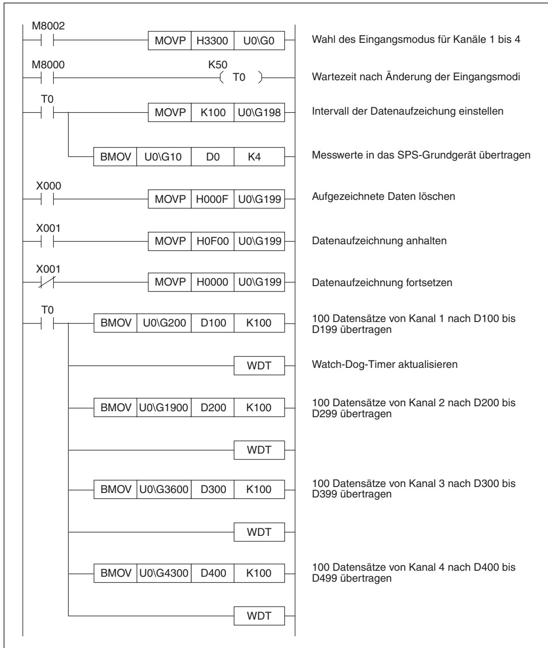
Abb. 5-35: Beispiel für ein Programm mit direktem Speicherzugriff zur Konfiguration der Datenaufzeichnung und zum Auslesen von aufgezeichneten Daten
