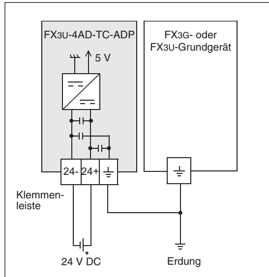
Abb. 13-7: Versorgung des FX3U-4AD-TC-ADP aus einer separaten Spannungsquelle
