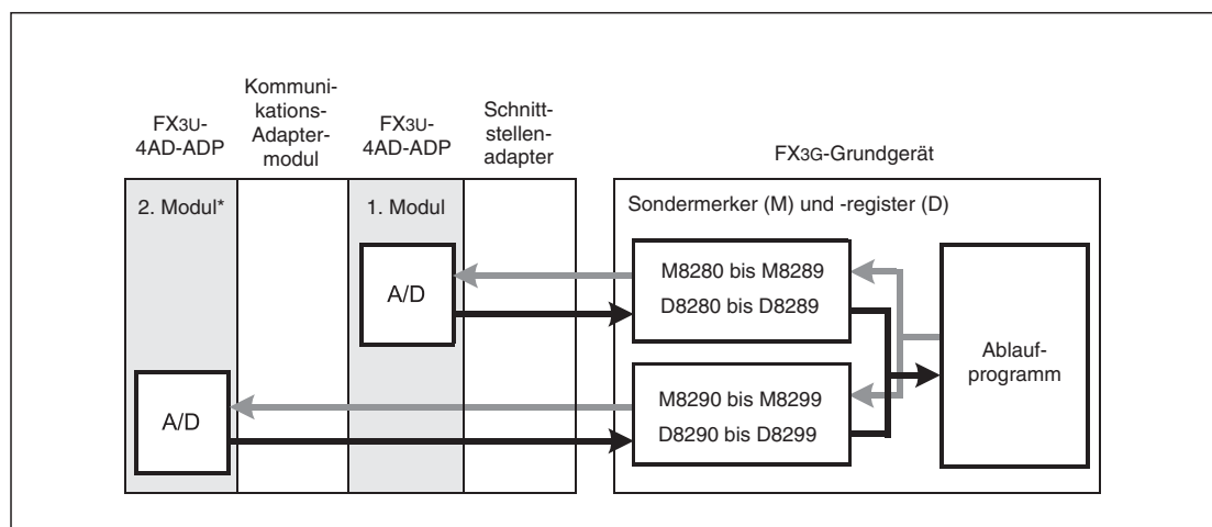
Abb. 4-11: Datenaustausch eines FX3G-Grundgeräts mit analogen Adaptermodulen
