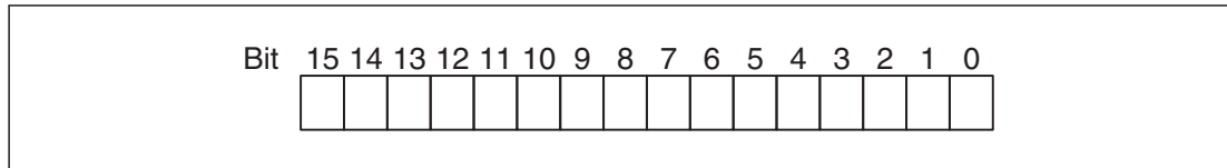
Abb. 8-12: Zuordnung der einzelnen Bit einer Pufferspeicheradresse
