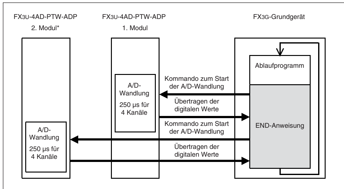
Abb. 11-1: Prinzip der Messwertverarbeitung bei FX3G-Grundgeräten (Maximal können zwei FX3U-4AD-PTW-ADP angeschlossen werden).
