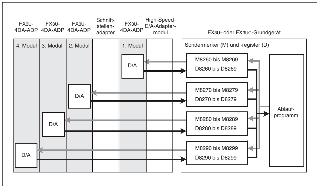
Abb. 7-12: Datenaustausch eines FX3U- oder FX3UC-Grundgeräts mit analogen Adaptermodulen
