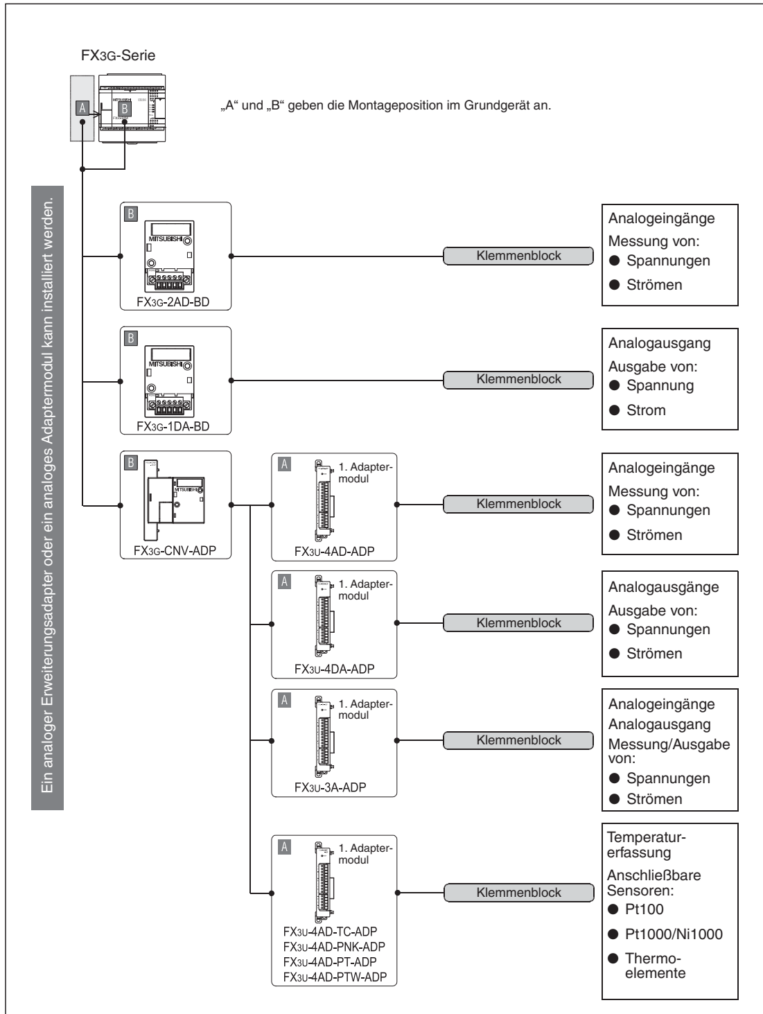
Abb. 1-11: Verwendbare Analogmodule für ein FX3G-Grundgerät mit 14 oder 24 Ein- und Ausgängen
