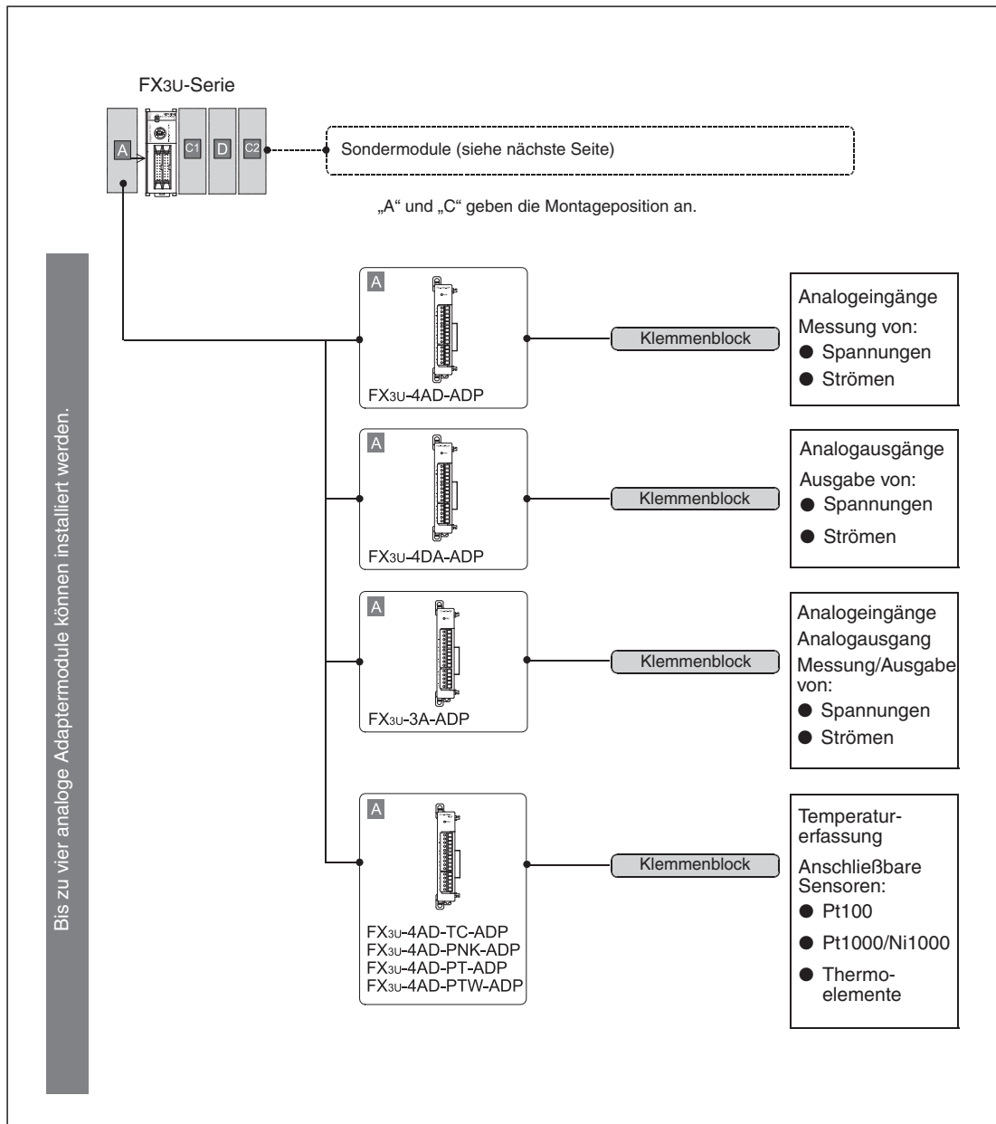
Abb. 1-16: Anschluss von analogen Adaptermodulen an ein Grundgerät der FX3UC-Serie
