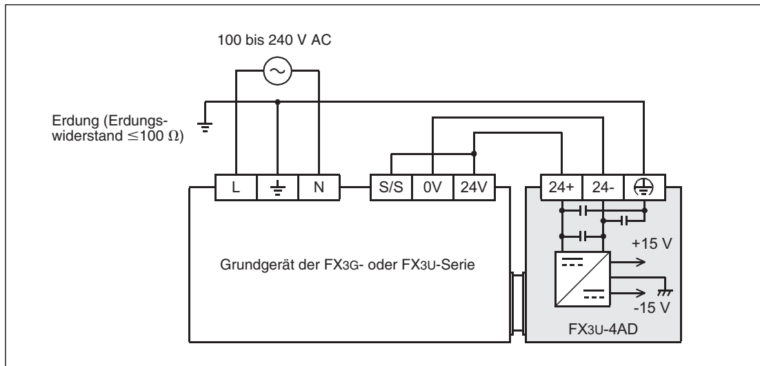
Abb. 5-13: Versorgung durch ein SPS-Grundgerät, das für minusschaltende Geber konfiguriert ist (Der Anschluss „S/S“ ist mit dem Anschluss „24V“ verbunden.)
