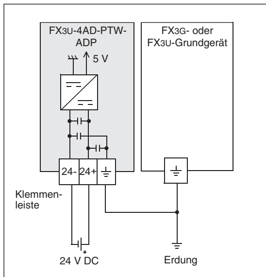
Abb. 11-6: Versorgung des FX3U-4AD-PTW-ADP aus einer separaten Spannungsquelle
