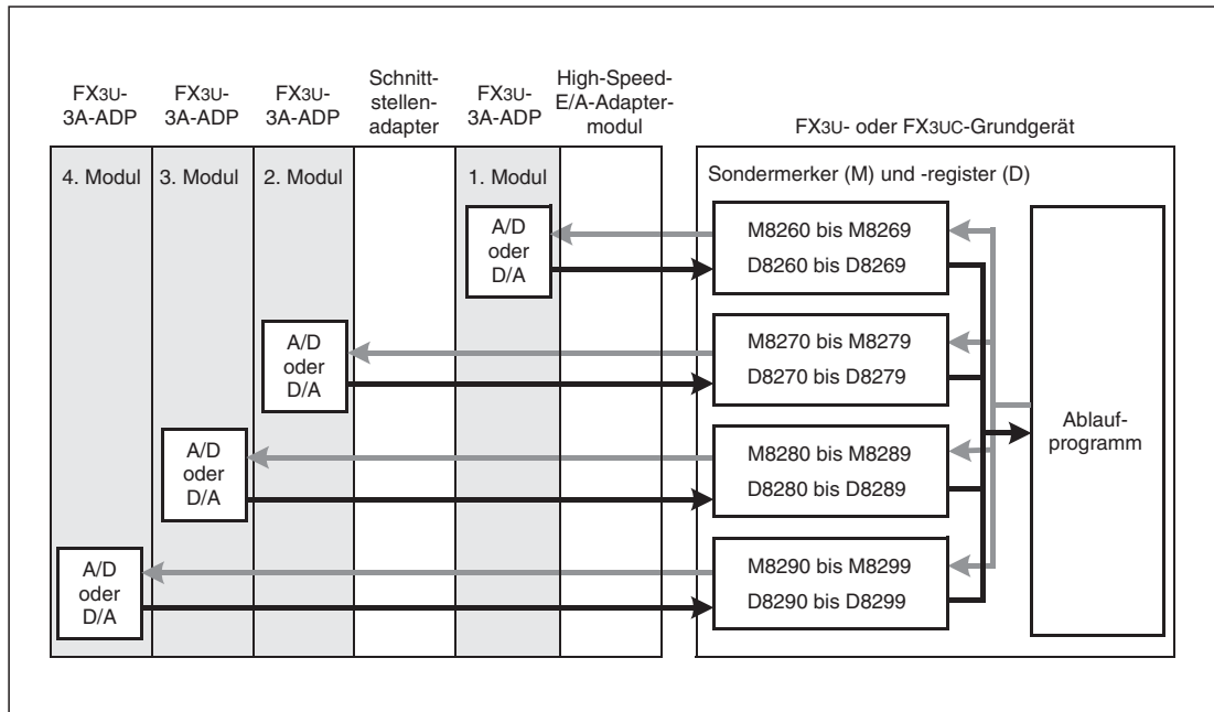
Abb. 9-13: Datenaustausch eines FX3U- oder FX3UC-Grundgeräts mit analogen Adaptermodulen
