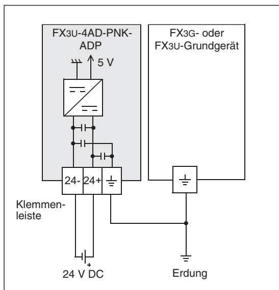
Abb. 12-6: Versorgung des FX3U-4AD-PNK-ADP aus einer separaten Spannungsquelle
