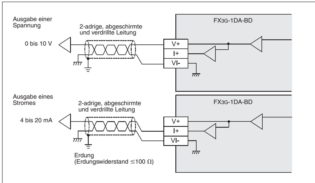
Abb. 6-5: Anschluss der analogen Signale an ein Analogausgangs-Erweiterungsadapter FX3G-1DA-BD
