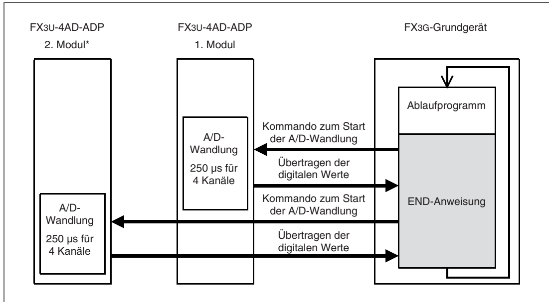
Abb. 4-1: Prinzip der Messwerterfassung bei FX3G-Grundgeräten (Maximal können zwei FX3U-4AD-ADP angeschlossen werden).
