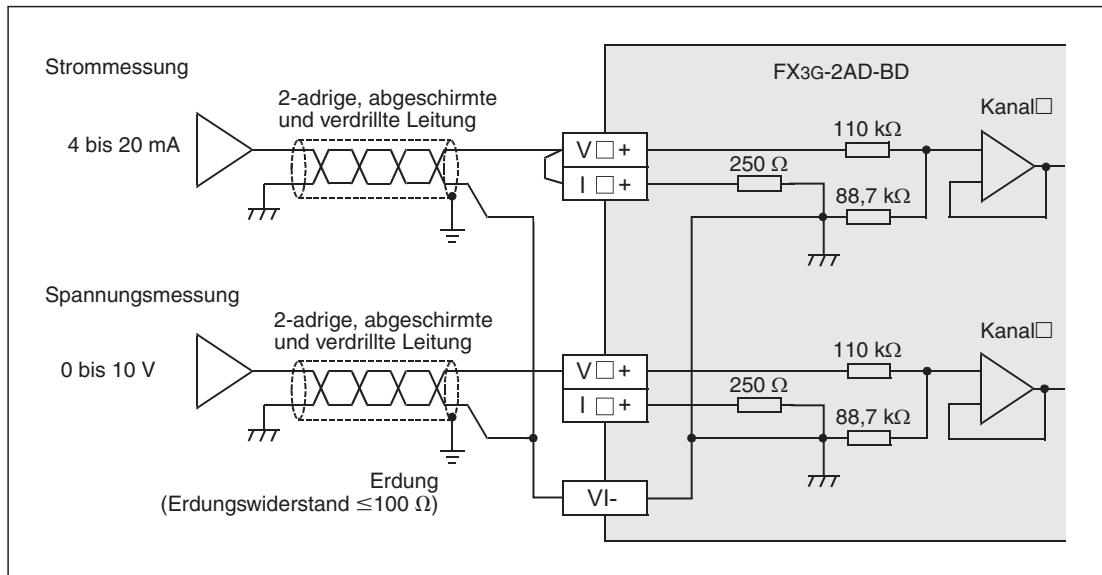
Abb. 3-5: Anschluss analoger Signale an einen Erweiterungsadapter FX3G-2AD-BD
