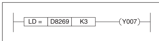
Abb. 3-12: Wenn auf dem 1. Erweiterungssteckplatz ein FX3G-2AD-BD installiert ist, wird der Ausgang Y007 eingeschaltet.
