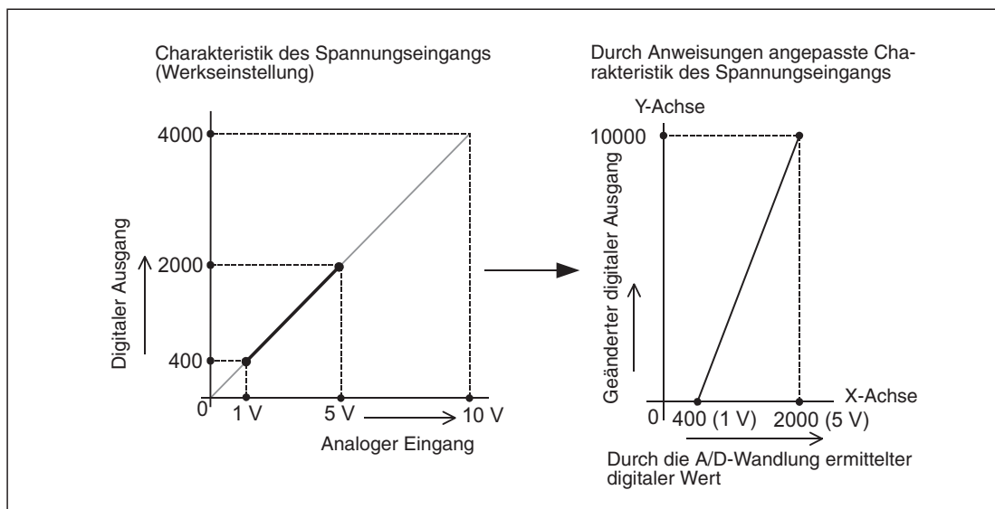
Abb. 4-24: In diesem Beispiel wird durch Anweisungen im Programm der Anfangspunkt und die Steigung einer Geraden verändert.
