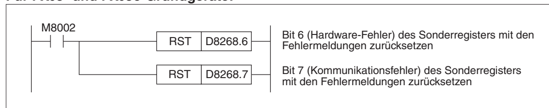
Abb. 9-23: Beispiel zum Zurücksetzen der Fehlermeldungen des FX3U-3A-ADP, das als 1. analoges Adaptermodul installiert ist.
