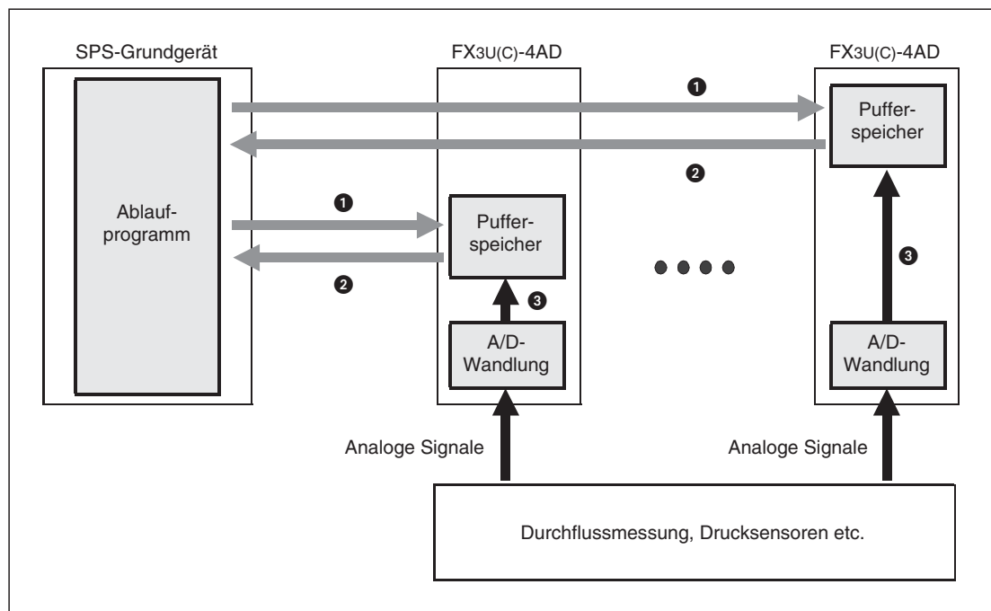
Abb. 5-20: Prinzip des Datenaustausches zwischen SPS-Grundgerät und Sondermodulen
