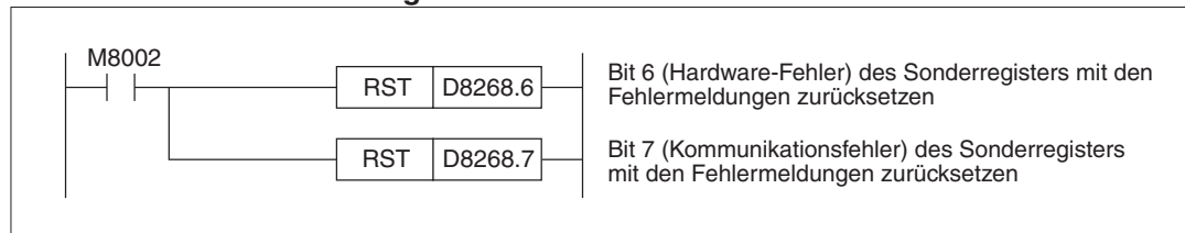
Abb. 11-18: Beispiel zum Zurücksetzen der Fehlermeldungen des FX3U-4AD-PTW-ADP, das als 1. analoges Adaptermodul installiert ist.
