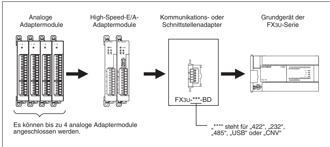
Abb. 1-6: Anschluss von Adaptermodulen an der linken Seite eines FX3U-Grundgeräts
