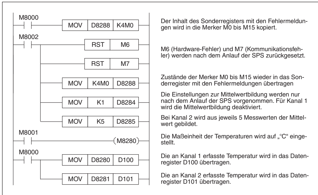
Abb. 11-22: Beispielprogramm zur Konfiguration von Kanal 1 und Kanal 2 eines FX3U-4AD-PTW-ADP
