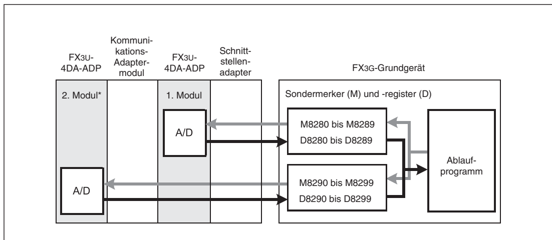
Abb. 7-11: Datenaustausch eines FX3G-Grundgeräts mit analogen Adaptermodulen
