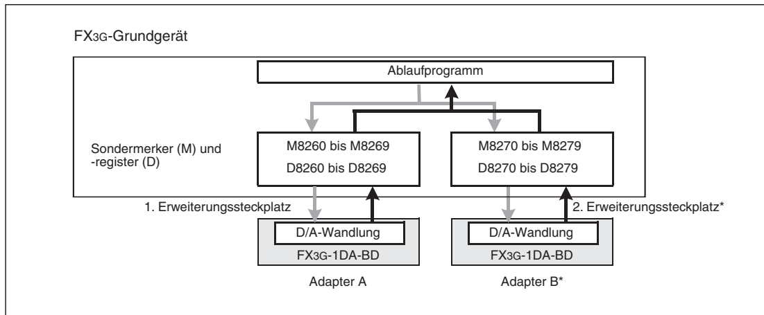
Abb. 6-6: Für jeden analogen Erweiterungsadapter sind 10 Sondermerker und 10 Sonderregister reserviert.
