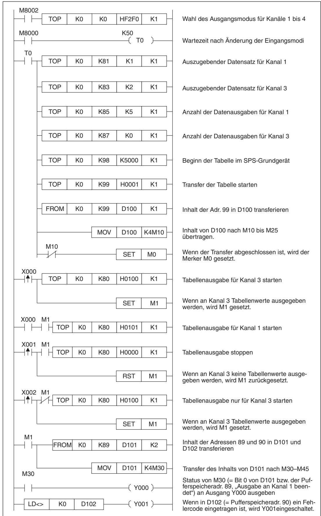
Abb. 8-40: Beispielprogramm zur Ausgabe von Werten aus einer Tabelle
