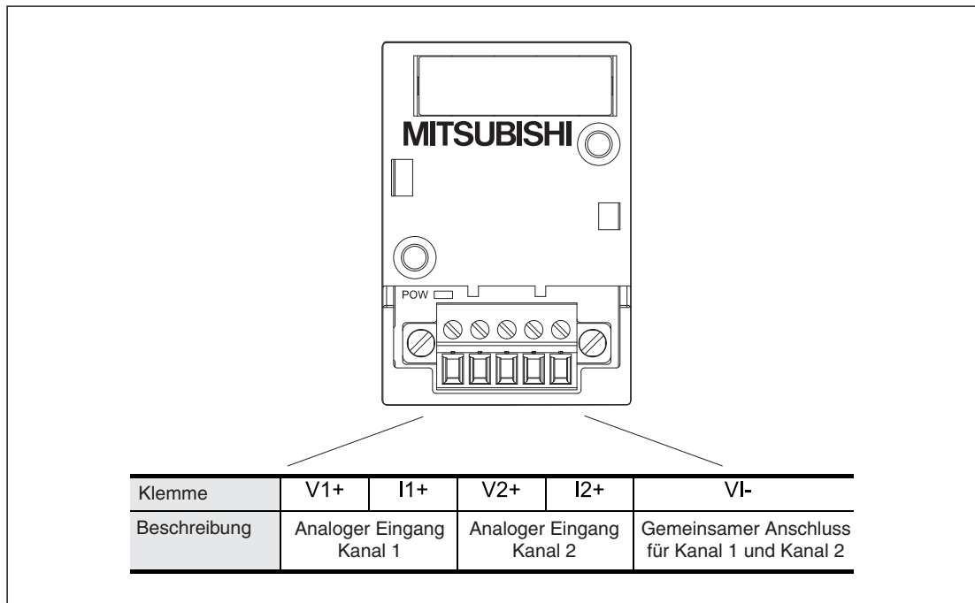
Abb. 3-4: Klemmenbelegung des FX3G-2AD-BD
