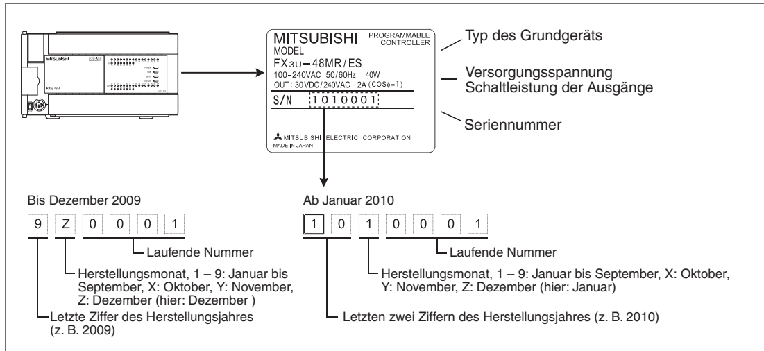
Abb. 1-18: Typenschild eines Grundgeräts der MELSEC FX3U-Serie
