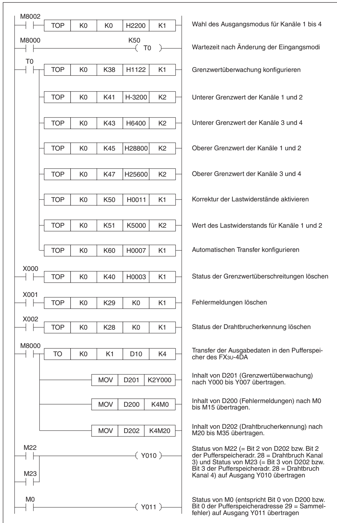
Abb. 8-38: Beispielprogramm zur Konfiguration erweiterter Funktionen des FX3U-4DA
