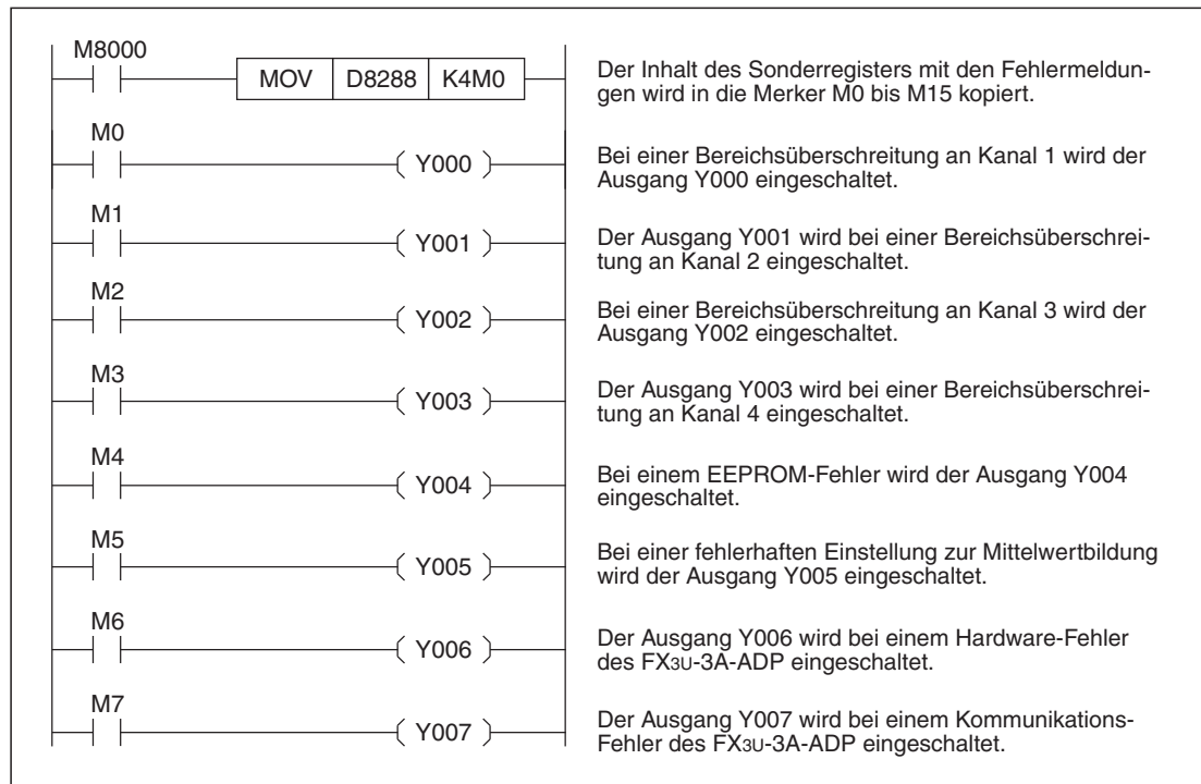
Abb. 9-24: Beispiel zur Auswertung von Fehlermeldungen eines FX3U-3A-ADP, das als 3. analoges Adaptermodul (1. Modul bei FX3G) installiert ist.
