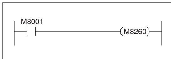
Abb. 6-7: Das FX3G-1DA-ADP, das auf dem 1. Erweiterungssteckplatz installiert ist, wird für die Ausgabe einer Spannung konfiguriert. Der Merker M8001 ist immer „0“.
