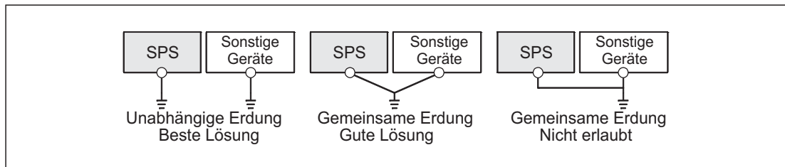
Abb. 9-8: Erdung der SPS
