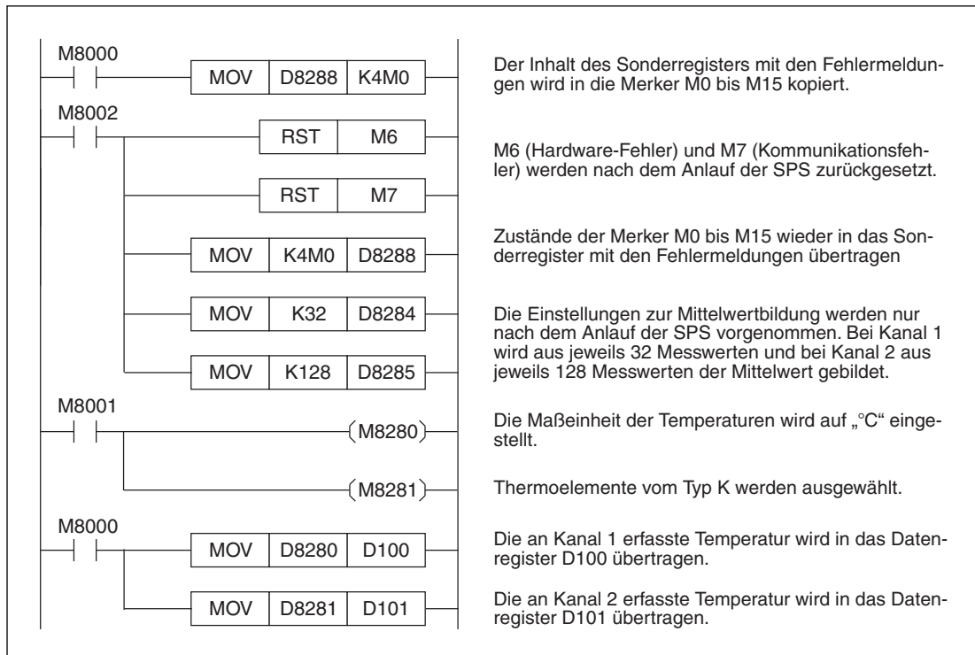
Abb. 13-24: Beispielprogramm zur Konfiguration von Kanal 1 und Kanal 2 eines FX3U-4AD-TC-ADP
