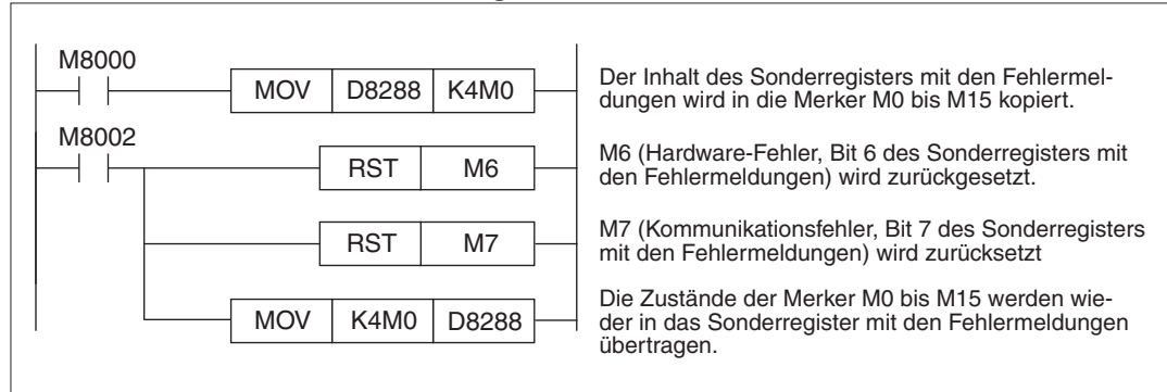
Abb. 4-17: Beispiel zum Zurücksetzen der Fehlermeldungen des FX3U-4AD-ADP, das als 3. analoges Adaptermodul (1. Modul bei FX3G) installiert ist.
