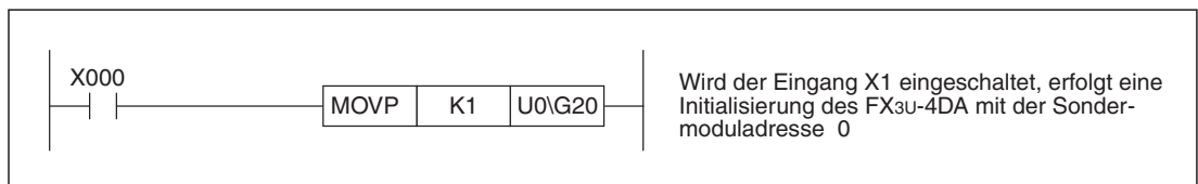
Abb. 8-17: Beispiel für eine Programmsequenz* für ein FX3U- oder FX3UC-Grundgerät zur Initialisierung eines FX3U-4DA
