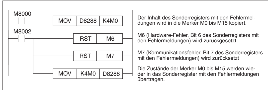
Abb. 10-17: Beispiel zum Zurücksetzen der Fehlermeldungen des FX3U-4AD-PT-ADP, das als 3. analoges Adaptermodul (1. Modul bei FX3G) installiert ist.
