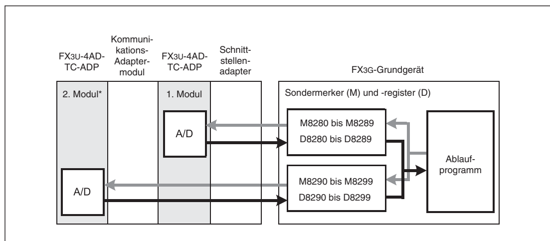
Abb. 13-12: Datenaustausch eines FX3G-Grundgeräts mit analogen Adaptermodulen
