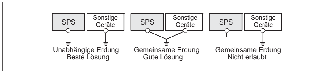
Abb. 10-9: Erdung der SPS
