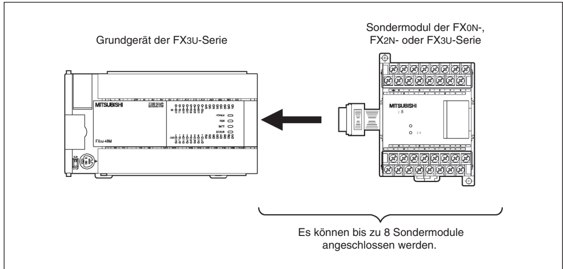
Abb. 1-9: Durch den Anschluss von Sondermodulen kann eine SPS der FX3U-Serie jeder Automatisierungsaufgabe angepasst werden.
