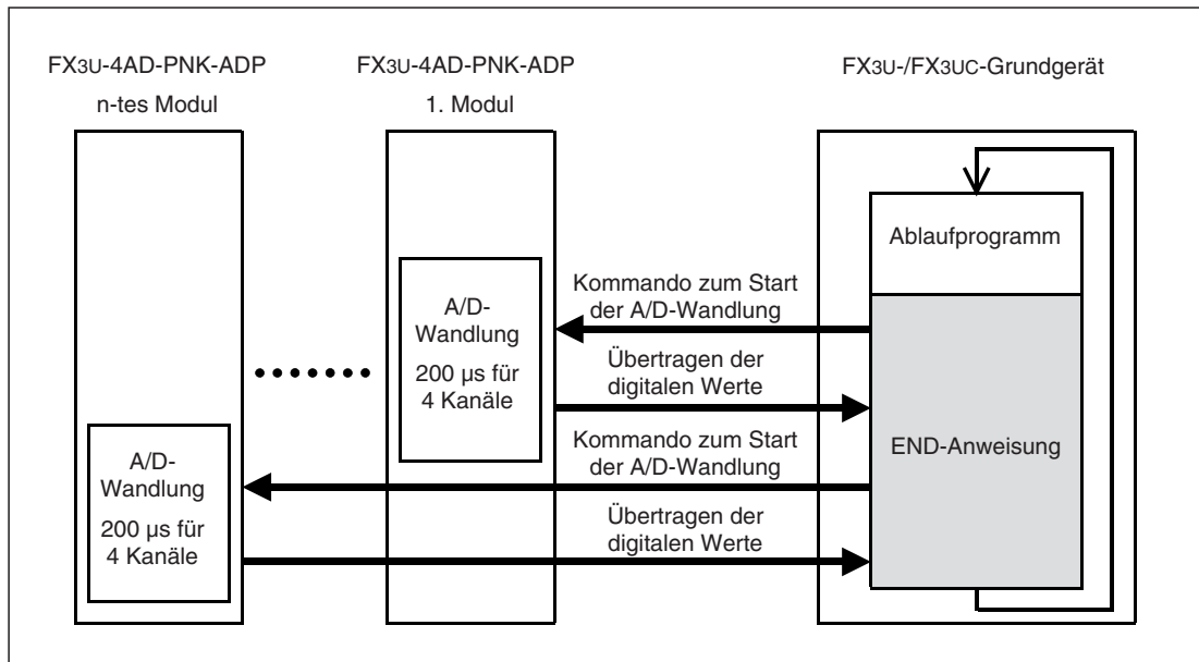
Abb. 12-2: Prinzip der Messwerterfassung bei FX3U- und FX3UC-Grundgeräten.
