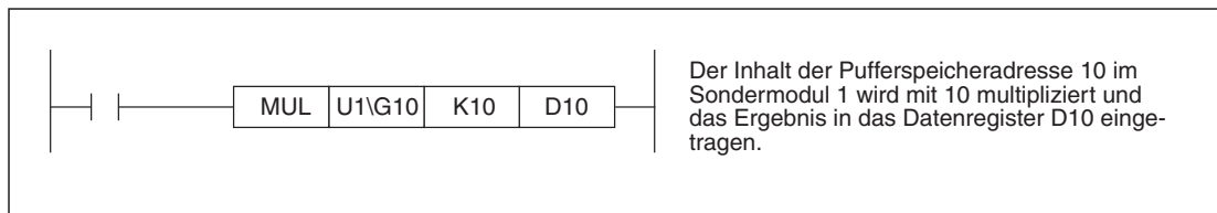
Abb. A-4: Anwendung des direkten Pufferspeicherzugriff bei einer Multiplikation
