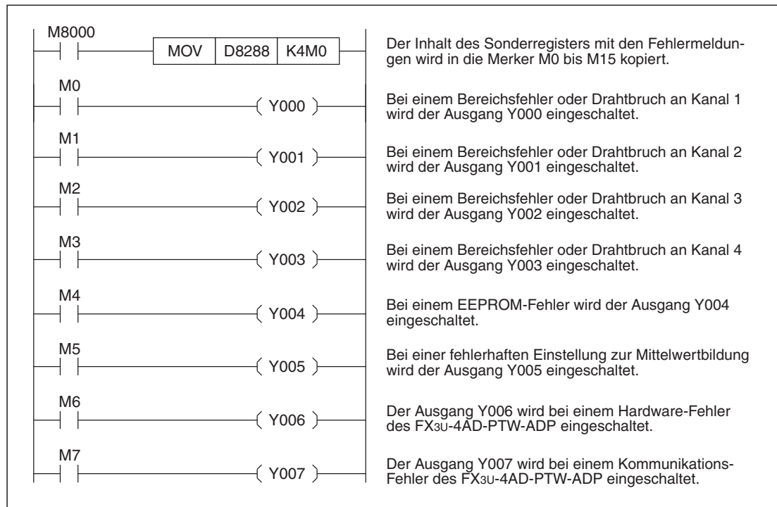
Abb. 11-19: Beispiel zur Auswertung von Fehlermeldungen eines FX3U-4AD-PTW-ADP, das als 3. analoges Adaptermodul (1. Modul bei FX3G) installiert ist.
