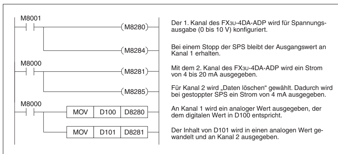
Abb. 7-21: Beispielprogramm für FX3G-, FX3U- oder FX3UC-Grundgeräte zur Konfiguration der Kanäle 1 und 2 eines FX3U-4DA-ADP, das als 3. bzw. 1. analoges Adaptermodul installiert ist.
