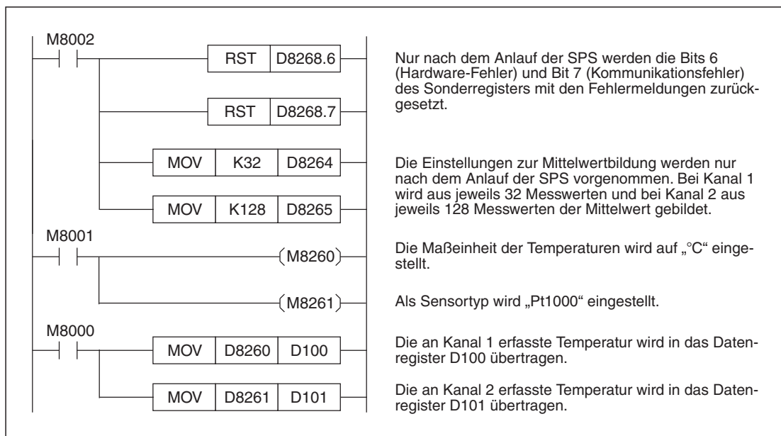
Abb. 12-25: Beispielprogramm zur Konfiguration von Kanal 1 und Kanal 2 eines FX3U-4AD-PNK-ADP, das als 1. analoges Adaptermodul installiert ist.
