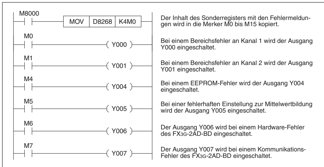
Abb. 3-13: Beispiel zur Auswertung von Fehlermeldungen eines FX3G-2AD-BD, das auf dem 1. Erweiterungssteckplatz installiert ist.
