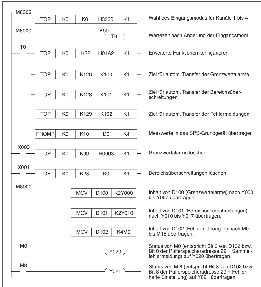
Abb. 5-32: Beispielprogramm zur Konfiguration erweiterter Funktionen des FX3U-4AD oder FX3UC-4AD
