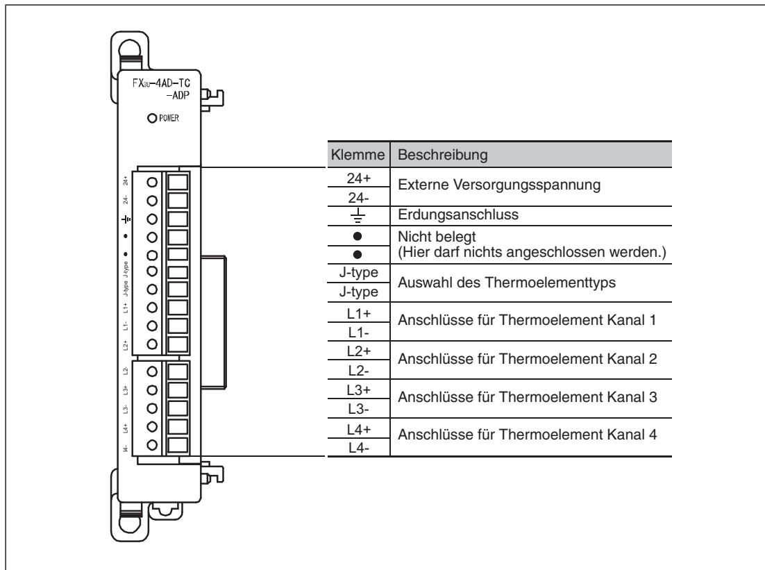
Abb. 13-5: Klemmenbelegung des FX3U-4AD-TC-ADP
