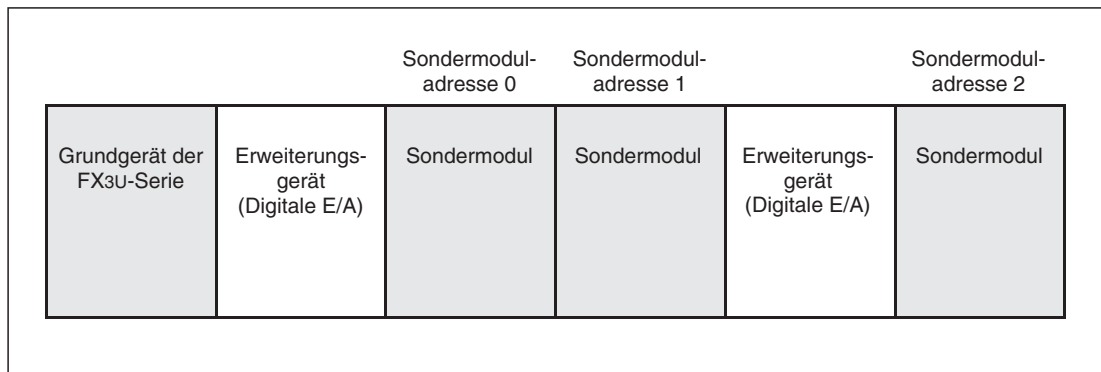
Abb. A-2: Beispiel für die Nummerierung von Sondermodulen
