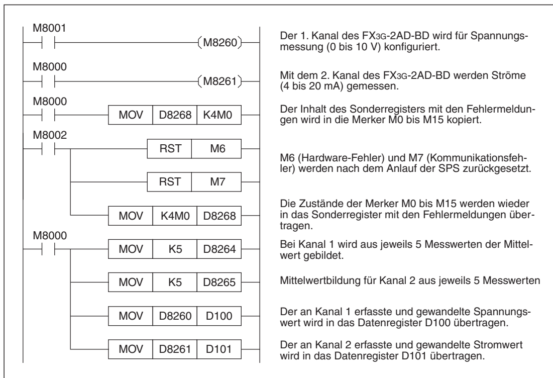
Abb. 3-14: Beispielprogramm zur Konfiguration von Kanal 1 und Kanal 2 eines FX3G-2AD-BD, das auf dem 1. Erweiterungssteckplatz installiert ist.
