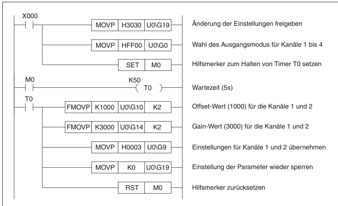
Abb. 8-35: Programmbeispiel für ein FX3U- oder FX3UC-Grundgerät zur Änderung der Ausgangscharakteristik der Kanäle 1 und 2
