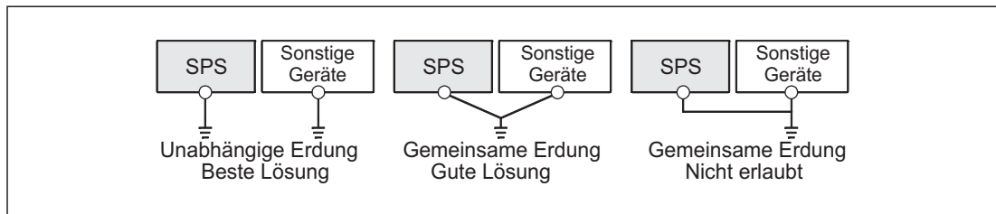
Abb. 12-9: Erdung der SPS
