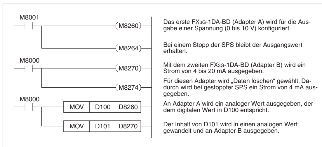
Abb. 6-12: Beispielprogramm zur Konfiguration von zwei analogen Erweiterungsadaptern FX3G-1DA-BD
