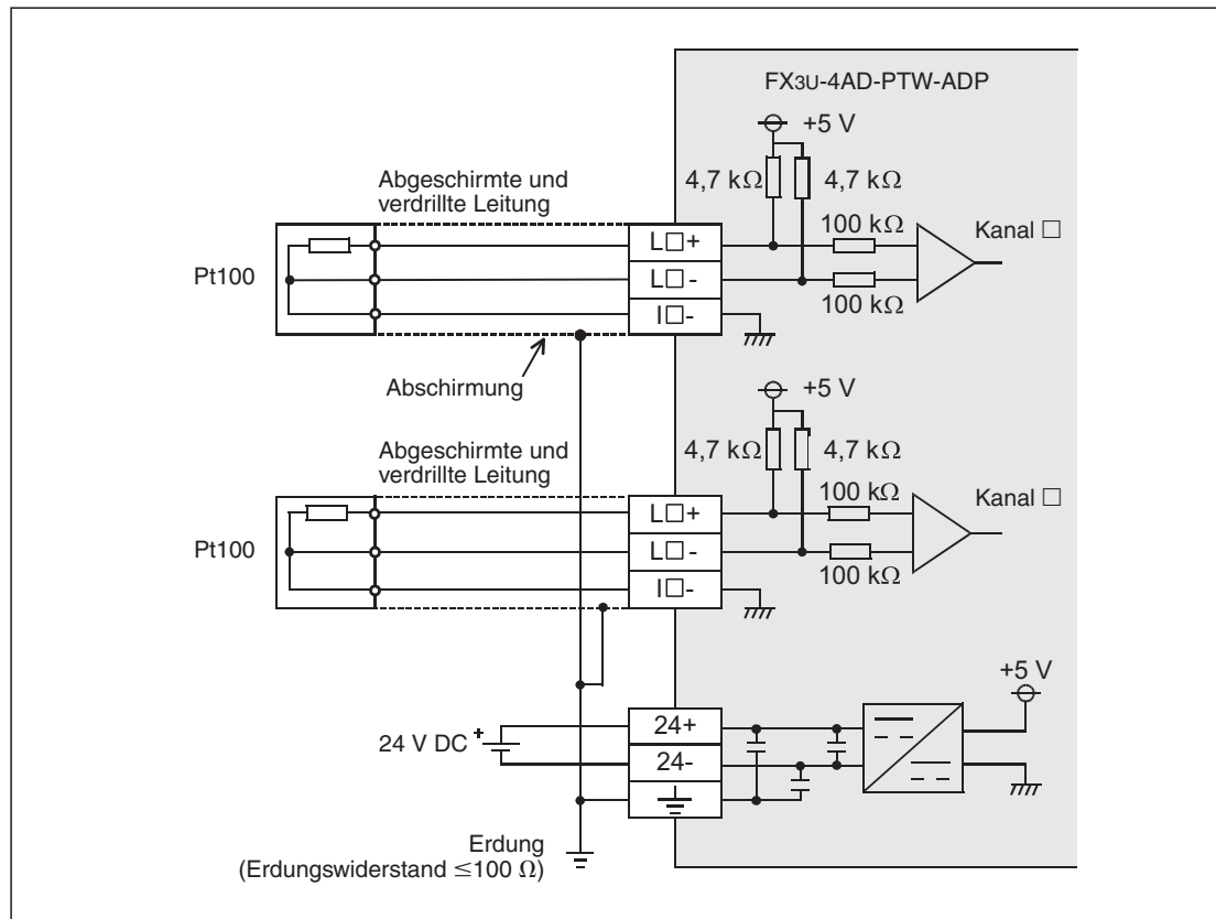
Abb. 11-10: Anschluss der Widerstandsthermometer an ein Temperaturerfassungs-Adaptermodul FX3U-4AD-PTW-ADP
