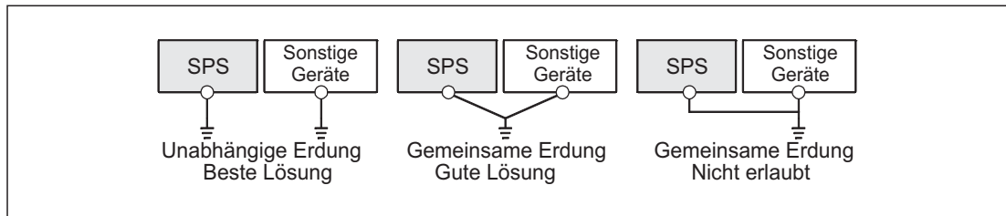
Abb. 5-16: Erdung der SPS
