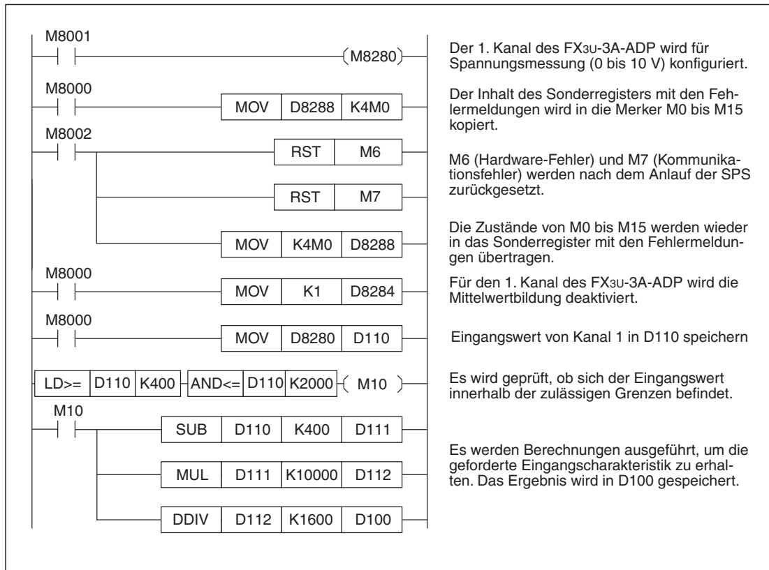
Abb. 9-30: Programmbeispiel zur Änderung der Charakteristik eines Spannungseingangs
