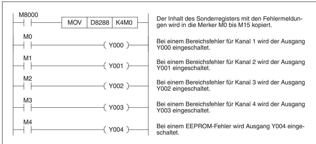
Abb. 7-19: Beispiel zur Auswertung der Fehlermeldungen eines FX3U-4DA-ADP, das als 3. analoges Adaptermodul (1. Modul bei FX3G) installiert ist.
