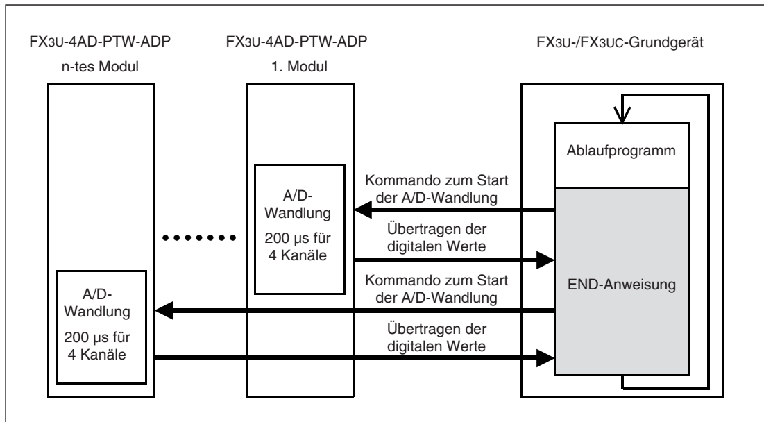
Abb. 11-2: Prinzip der Messwerterfassung bei FX3U- und FX3UC-Grundgeräten.
