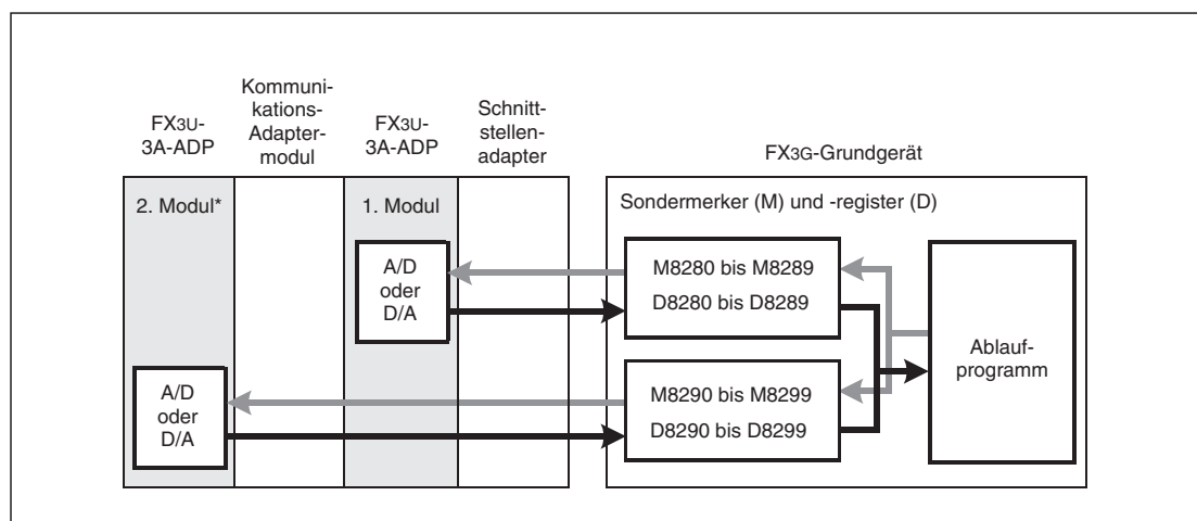
Abb. 9-12: Datenaustausch eines FX3G-Grundgeräts mit analogen Adaptermodulen
