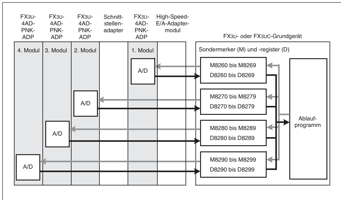
Abb. 12-12: Datenaustausch eines FX3U- oder FX3UC-Grundgeräts mit analogen Adaptermodulen
