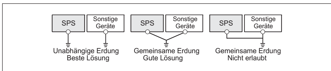
Abb. 8-10: Erdung der SPS
