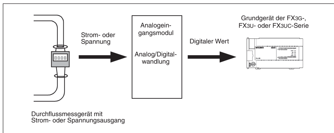
Abb. 1-1: Beispiel für eine Durchflussmessung mit einer SPS der MELSEC FX-Familie
