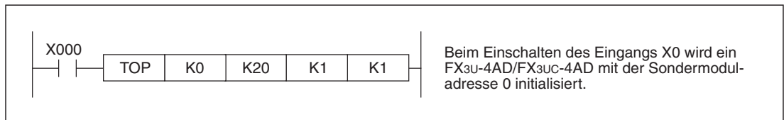
Abb. 8-18: Beispiel für FX3G-, FX3U- oder FX3UC-Grundgeräte zur Initialisierung eines FX3U-4DA.
