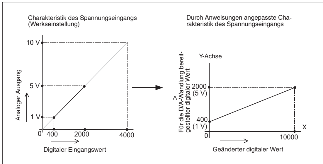
Abb. 9-32: In diesem Beispiel wird durch Anweisungen im Programm der Anfangspunkt und die Steigung einer Geraden verändert.
