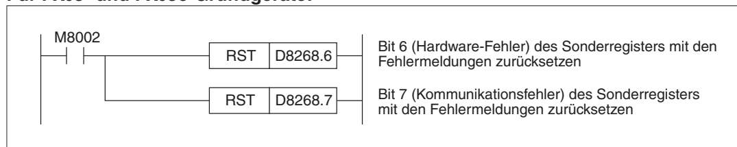
Abb. 10-18: Beispiel zum Zurücksetzen der Fehlermeldungen des FX3U-4AD-PT-ADP, das als 1. analoges Adaptermodul installiert ist.
