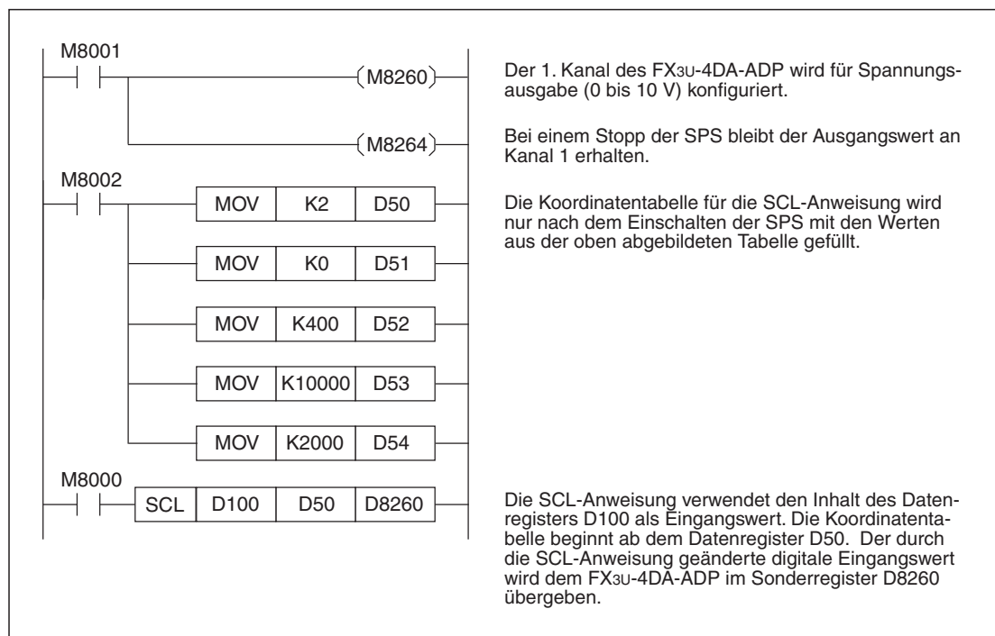
Abb. 7-24: Programmbeispiel zur Änderung der Charakteristik eines Spannungseingangs durch eine SCL-Anweisung
