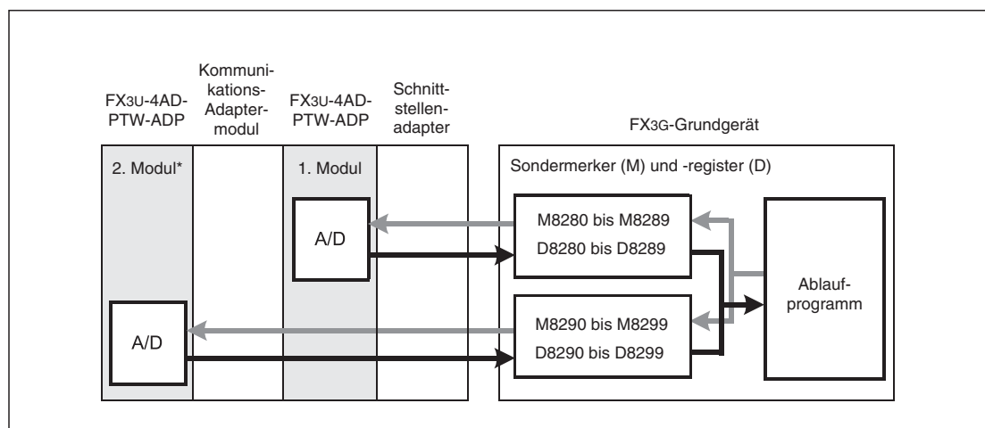
Abb. 11-11: Datenaustausch eines FX3G-Grundgeräts mit analogen Adaptermodulen
