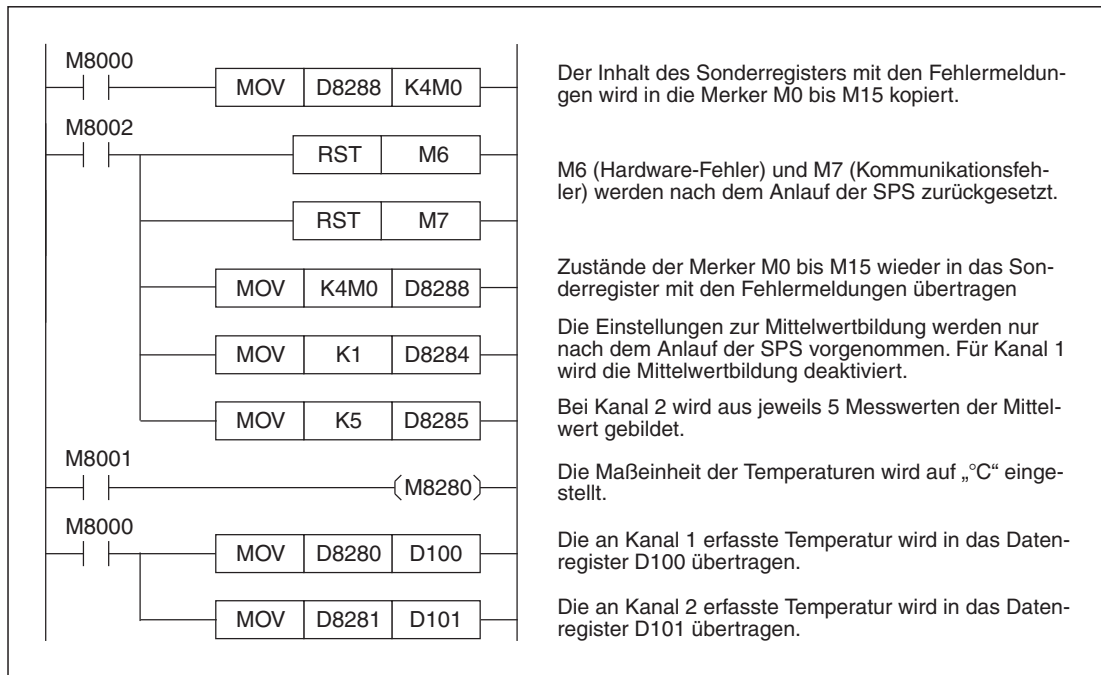
Abb. 10-22: Beispielprogramm zur Konfiguration von Kanal 1 und Kanal 2 eines FX3U-4AD-PT-ADP
