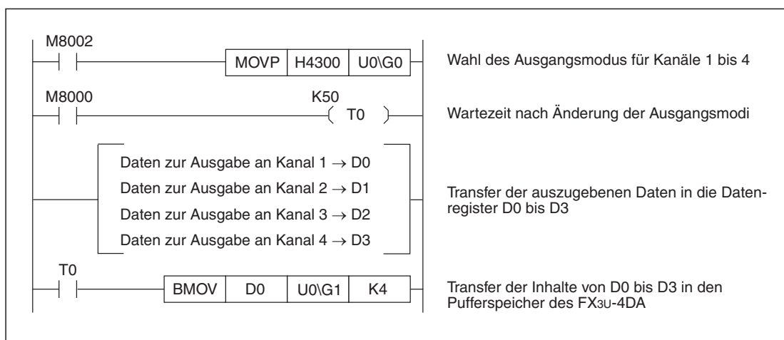
Abb. 8-37: Beispielprogramm mit direktem Speicherzugriff zur Einstellung der Ausgangsmodi und der Ausgabe von analogen Werten
