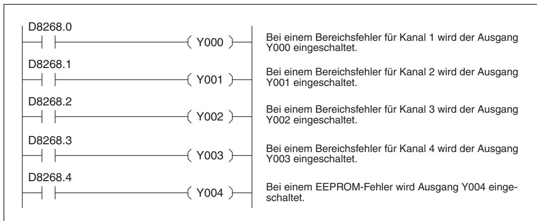
Abb. 7-20: Beispiel zur Auswertung der Fehlermeldungen eines FX3U-4DA-ADP, das als 1. analoges Adaptermodul installiert ist.
