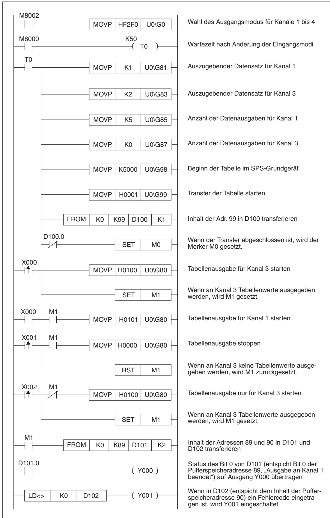
Abb. 8-41: Beispielprogramm mit direktem Speicherzugriff zur Ausgabe von Werten aus einer Tabelle
