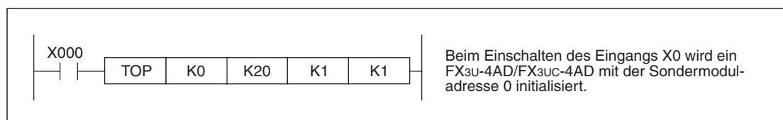
Abb. 5-24: Beispiel für FX3G-, FX3U- oder FX3UC-Grundgeräte zur Initialisierung eines FX3U-4AD oder FX3UC-4AD.
