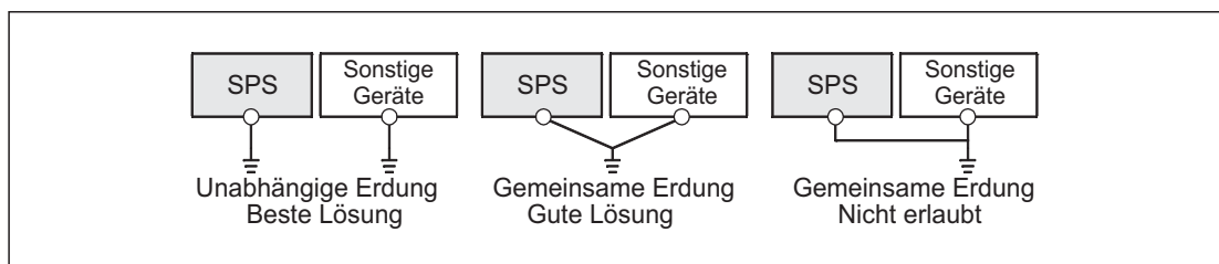
Abb. 13-8: Erdung der SPS
