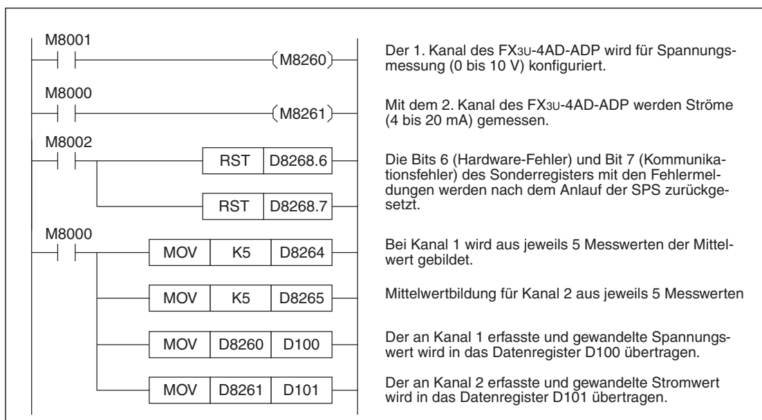
Abb. 4-23: Beispielprogramm zur Konfiguration von Kanal 1 und Kanal 2 eines FX3U-4AD-ADP, das als 1. analoges Adaptermodul installiert ist.
