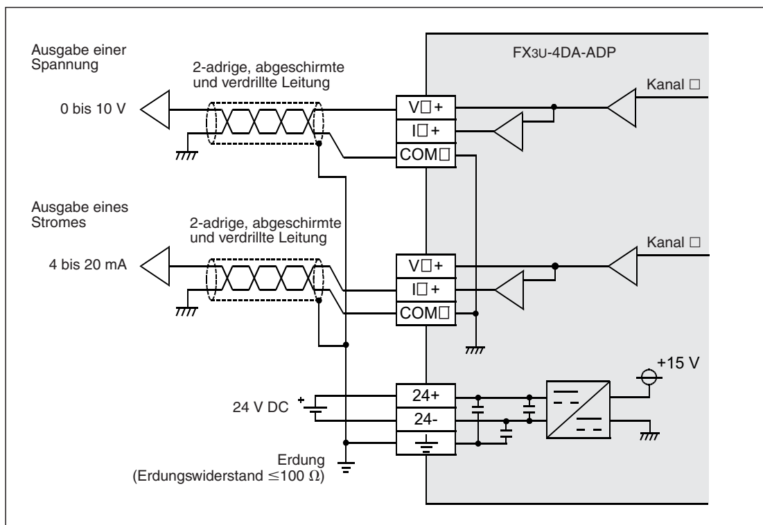
Abb. 7-10: Anschluss der analogen Signale an ein Analogausgangs-Adaptermodul FX3U-4DA-ADP
