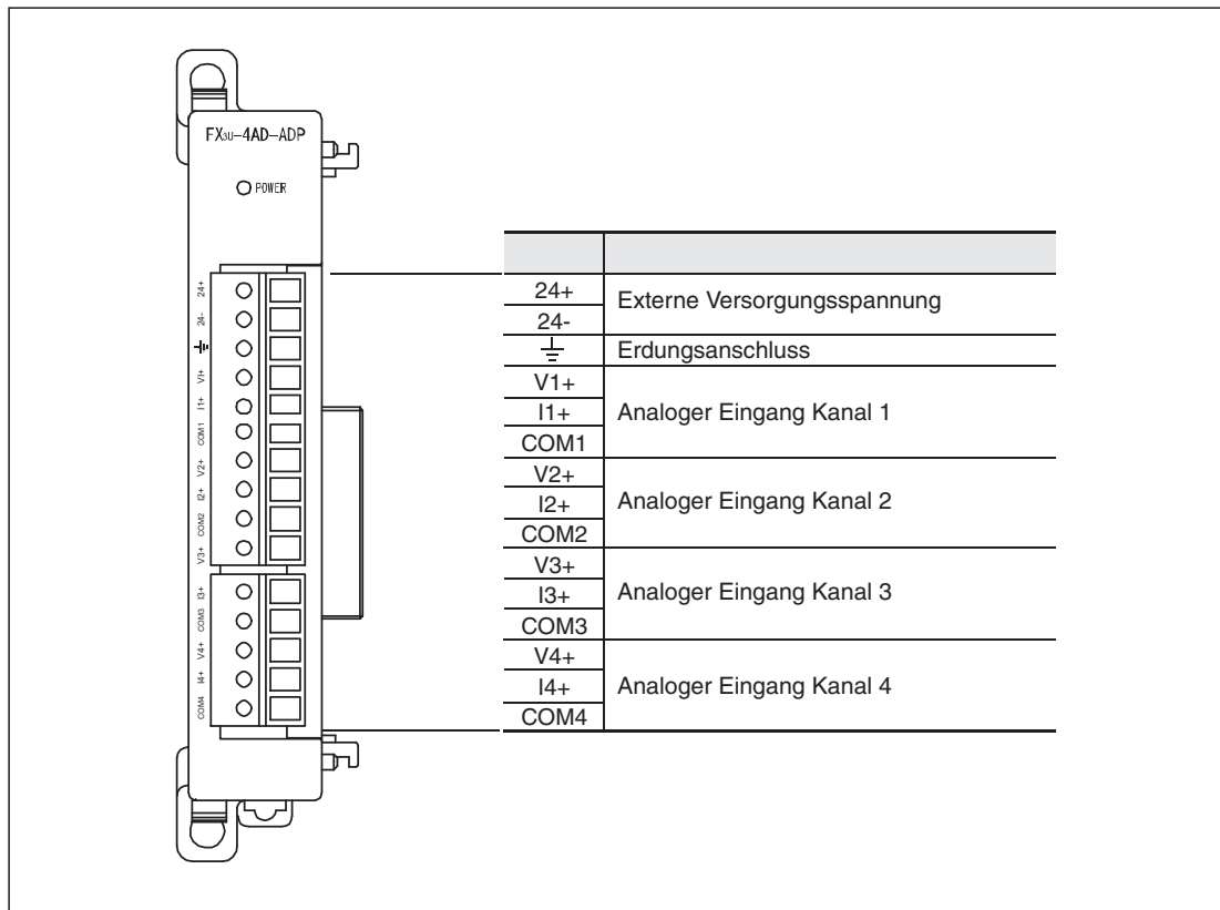
Abb. 4-6: Klemmenbelegung des FX3U-4AD-ADP
