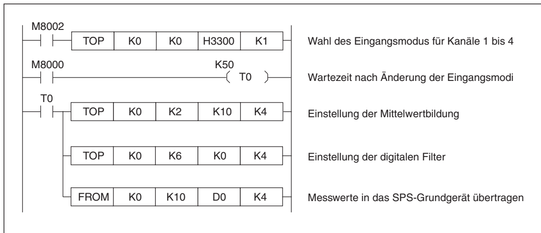
Abb. 5-30: Beispielprogramm zur Konfiguration der Mittelwertbildung und der digitalen Filter
