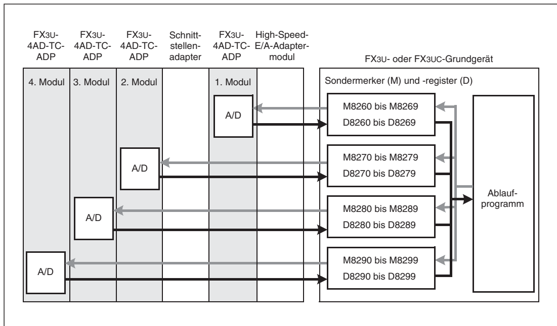
Abb. 13-13: Datenaustausch eines FX3U- oder FX3UC-Grundgeräts mit analogen Adaptermodulen
