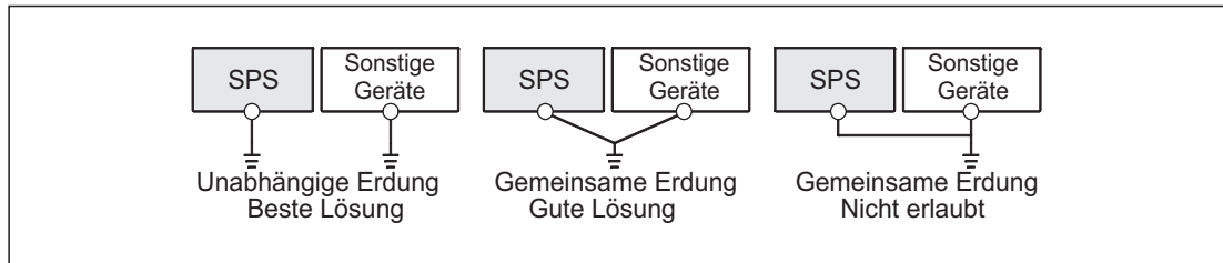
Abb. 4-9: Erdung der SPS
