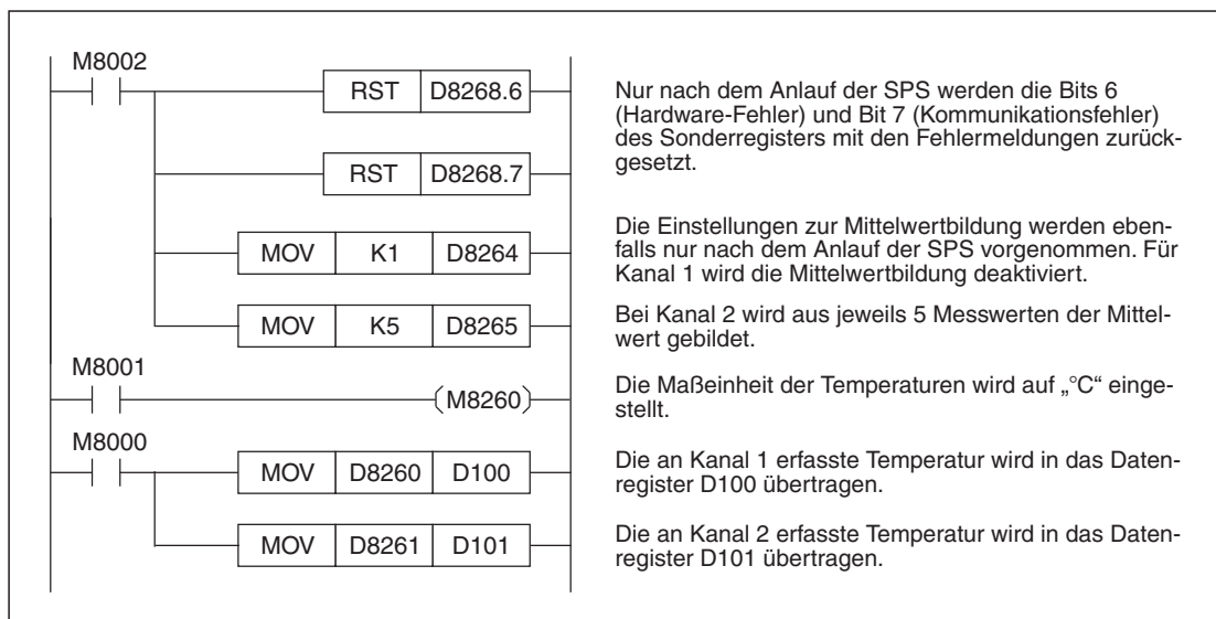
Abb. 11-23: Beispielprogramm zur Konfiguration von Kanal 1 und Kanal 2 eines FX3U-4AD-PTW-ADP, das als 1. analoges Adaptermodul installiert ist.
