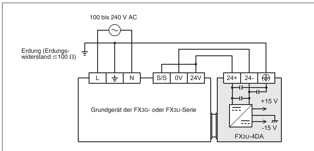
Abb. 8-8: Versorgung durch ein SPS-Grundgerät, das für minusschaltende Geber konfiguriert ist (Der Anschluss „S/S“ ist mit dem Anschluss „24V“ verbunden.)
