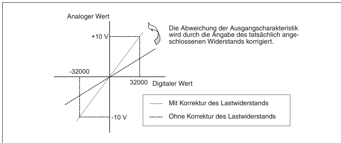
Abb. 8-22: Funktion der Korrektur des Lastwiderstands
