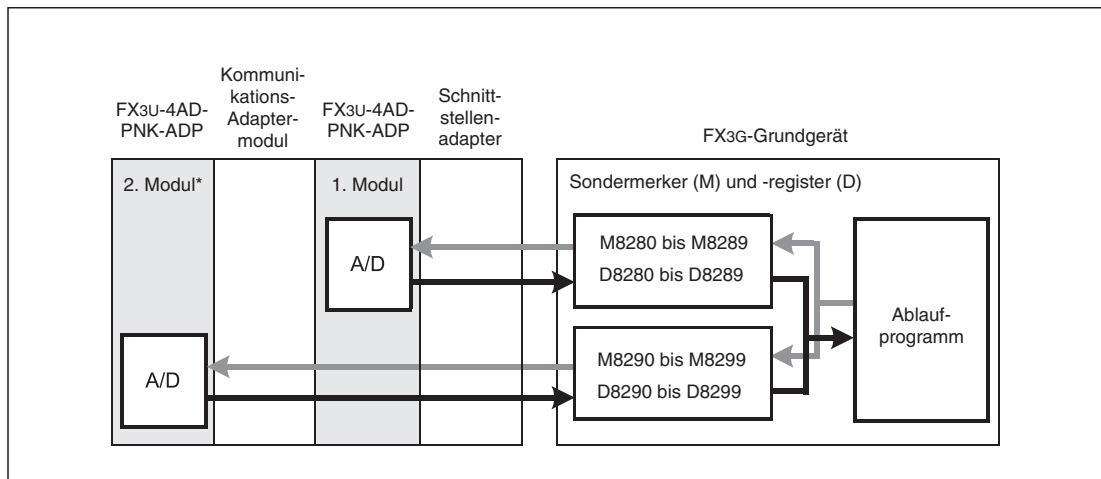
Abb. 12-11: Datenaustausch eines FX3G-Grundgeräts mit analogen Adaptermodulen
