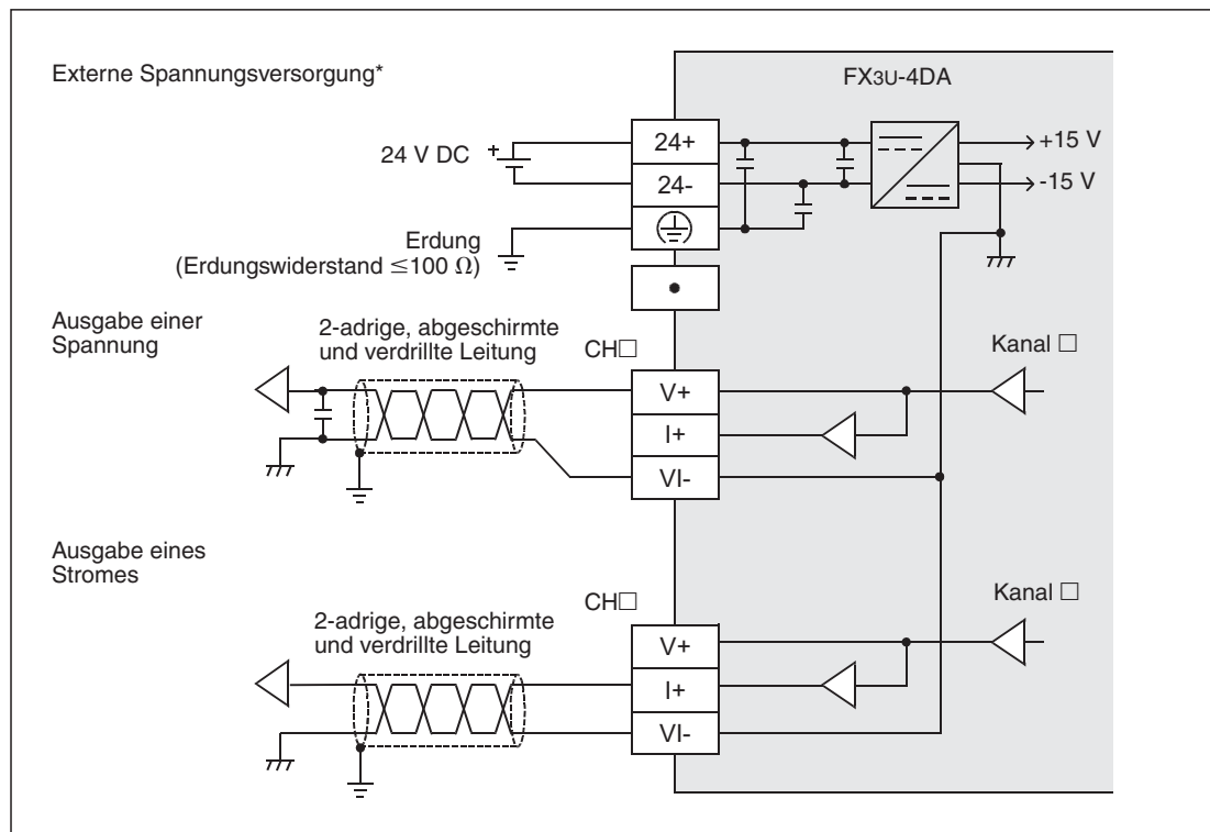
Abb. 8-11: Anschluss der analogen Signale an ein Analogausgangsmodule FX3U-4DA
