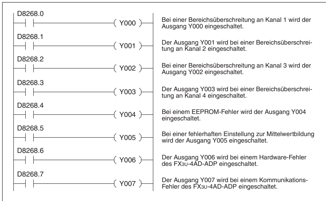
Abb. 4-20: Beispiel zur Auswertung von Fehlermeldungen eines FX3U-4AD-ADP, das als 1. analoges Adaptermodul installiert ist.
