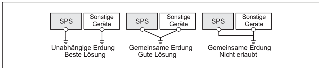
Abb. 7-9: Erdung der SPS
