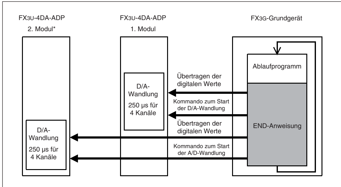
Abb. 7-1: Prinzip der Analogwertausgabe bei FX3G-Grundgeräten (Maximal können zwei FX3U-4AD-ADP angeschlossen werden).
