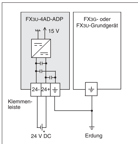
Abb. 4-5: Versorgung des FX3U-4AD-ADP aus einer separaten Spannungsquelle
