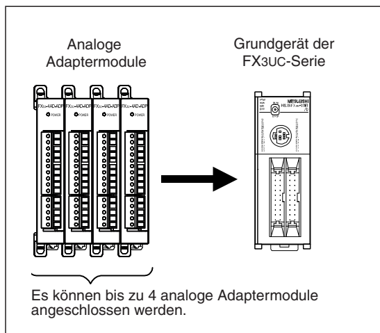
Abb. 1-7: Adaptermodule können direkt an ein Grundgerät der FX3UC-Serie angeschlossen werden.
