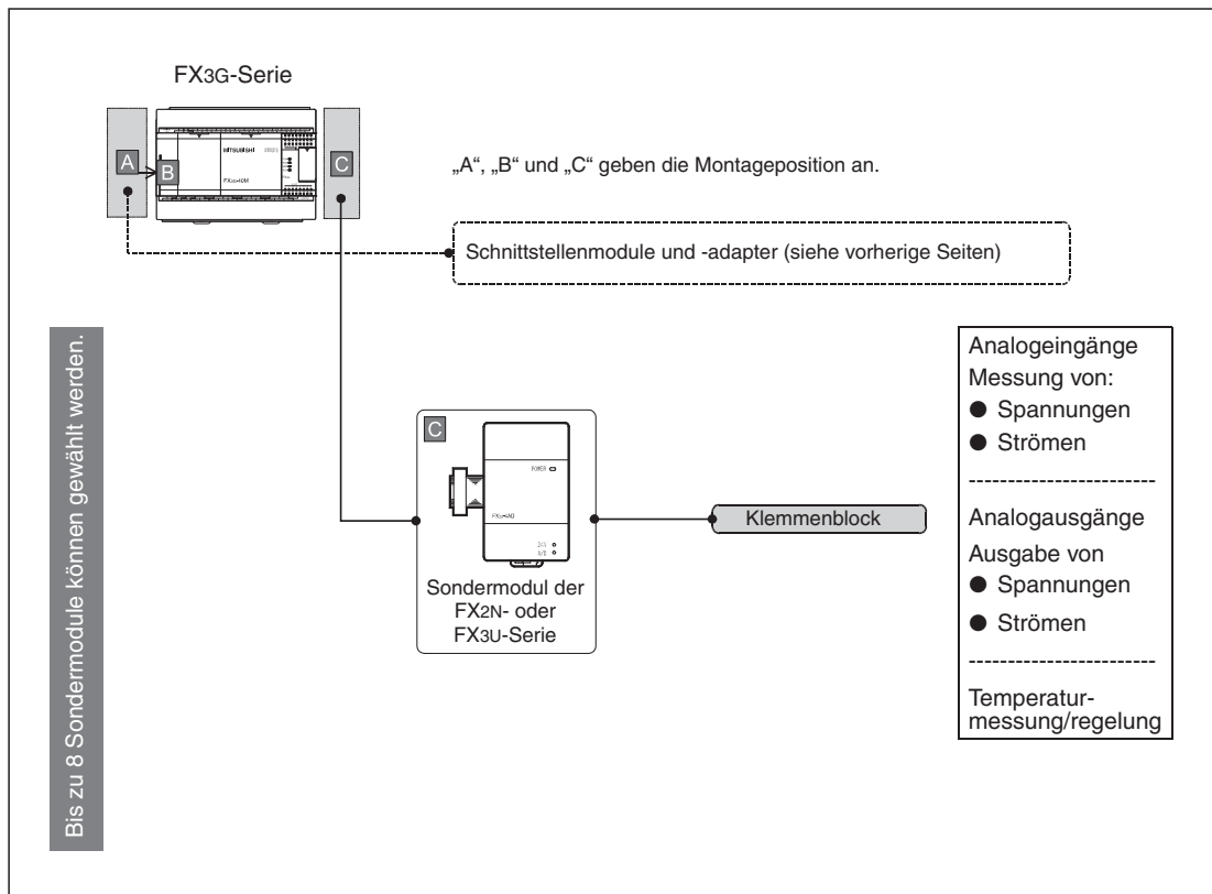
Abb. 1-13: Anschluss von Sondermodulen an ein Grundgerät der FX3G-Serie
