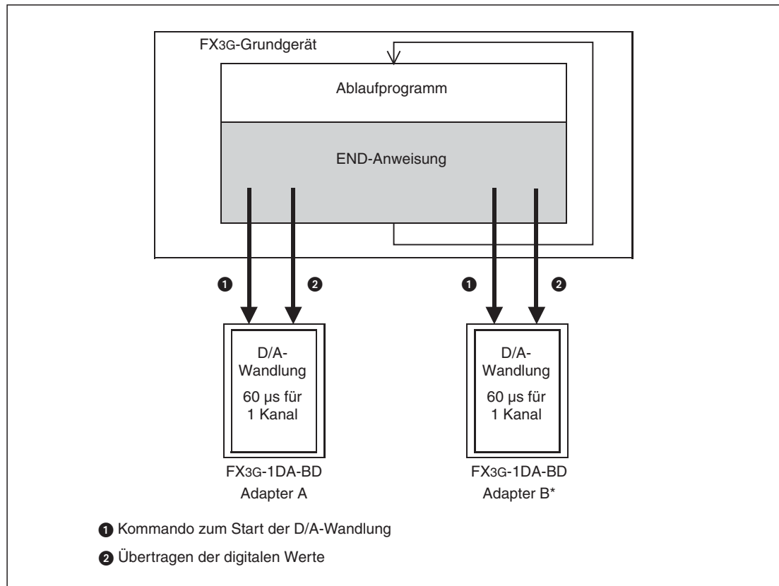
Abb. 6-1: Bei der Ausführung der END-Anweisung werden die digitalen Werte gewandelt und als analoge Signale ausgegeben.
