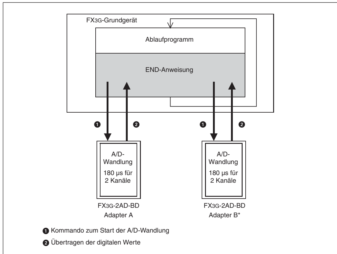
Abb. 3-1: Bei der Ausführung der END-Anweisung werden die analogen Werte gewandelt und in das Grundgerät übertragen.
