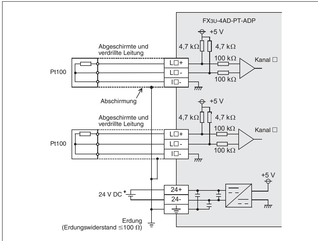
Abb. 10-10: Anschluss der Widerstandsthermometer an ein Temperaturerfassungs-Adaptermodul FX3U-4AD-PT-ADP
