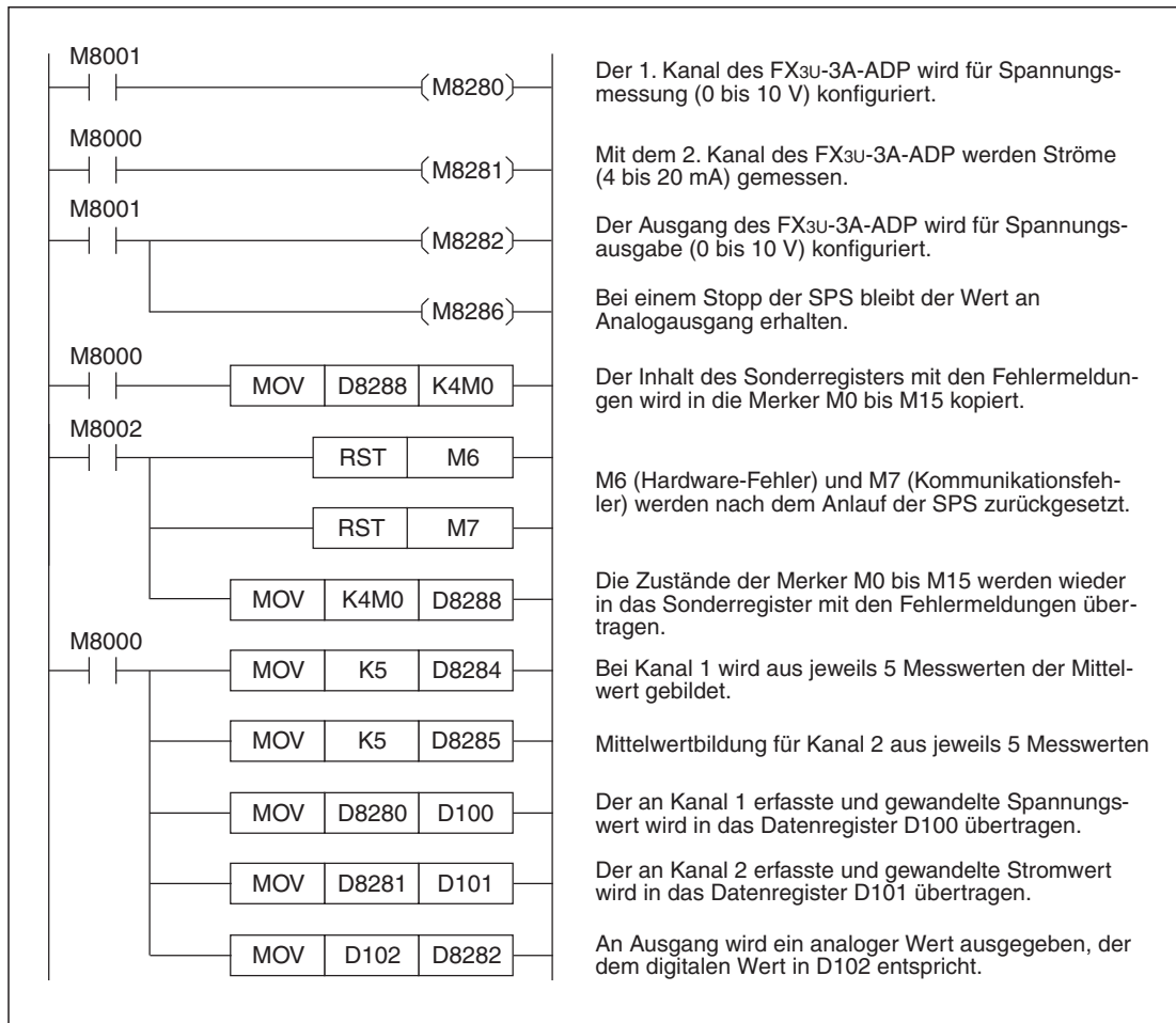
Abb. 9-27: Beispielprogramm zum Messen und zur Ausgabe von Analogwerten mit einem FX3U-3A-ADP
