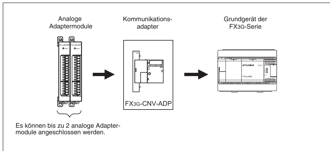
Abb. 1-5: Anschluss von Adaptermodulen an der linken Seite eines FX3G-Grundgeräts
