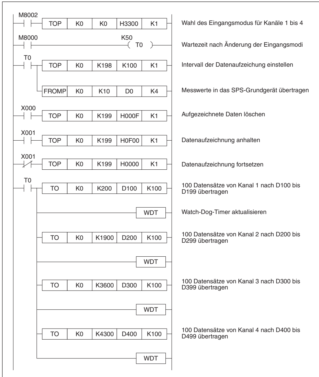
Abb. 5-34: Beispielprogramm zur Konfiguration der Datenaufzeichnung und zum Auslesen von aufgezeichneten Daten
