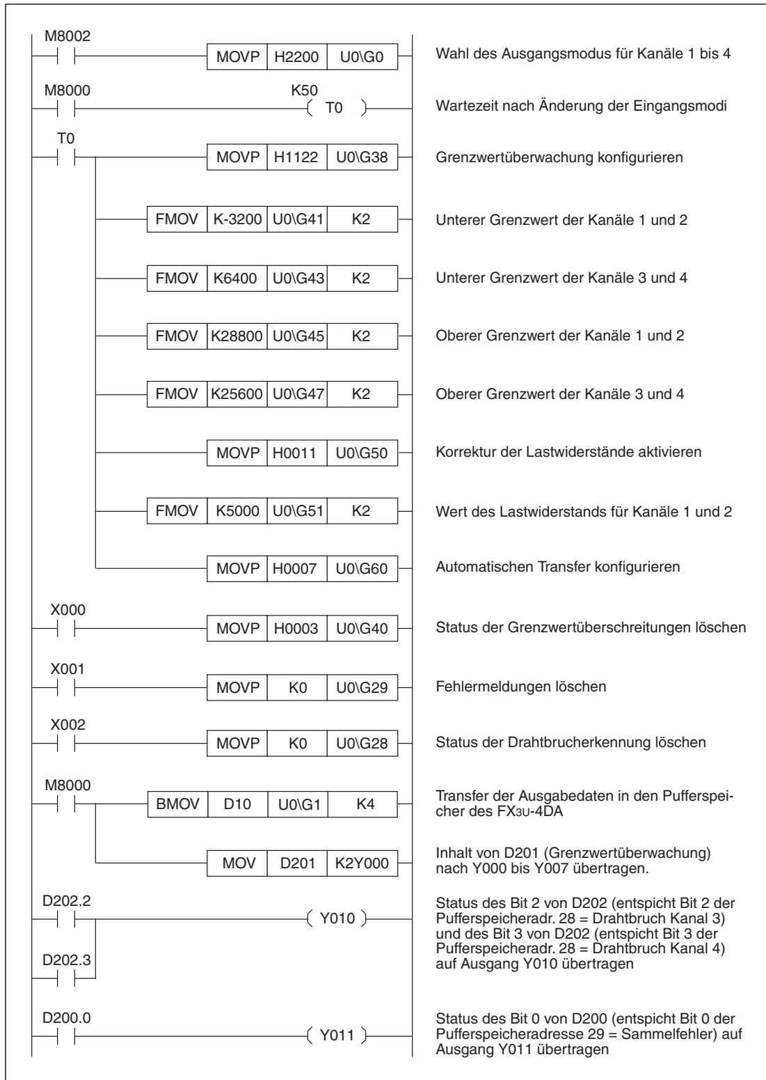
Abb. 8-39: Beispielprogramm mit direktem Speicherzugriff zur Konfiguration erweiterter Funktionen des FX3U-4DA
