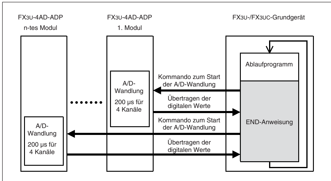
Abb. 4-2: Prinzip der Messwerterfassung bei FX3U- und FX3UC-Grundgeräten.
