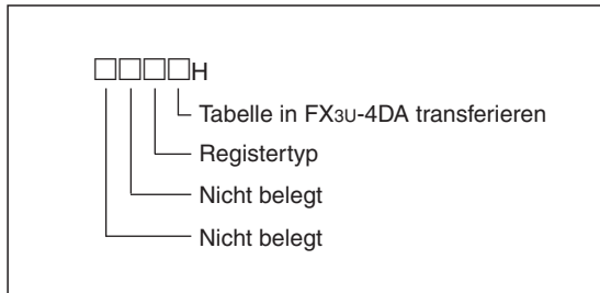
Abb. 8-30: Belegung der Pufferspeicheradresse 99
