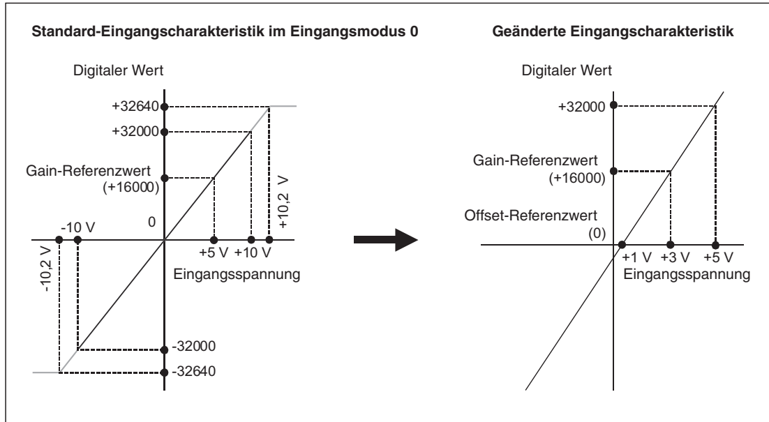
Abb. 5-25: Die Standard-Eingangscharakteristik für den Eingangsmodus 0 wird verändert.
