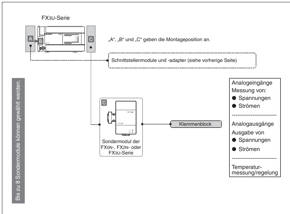
Abb. 1-15: Anschluss von Sondermodulen an ein Grundgerät der FX3U-Serie
