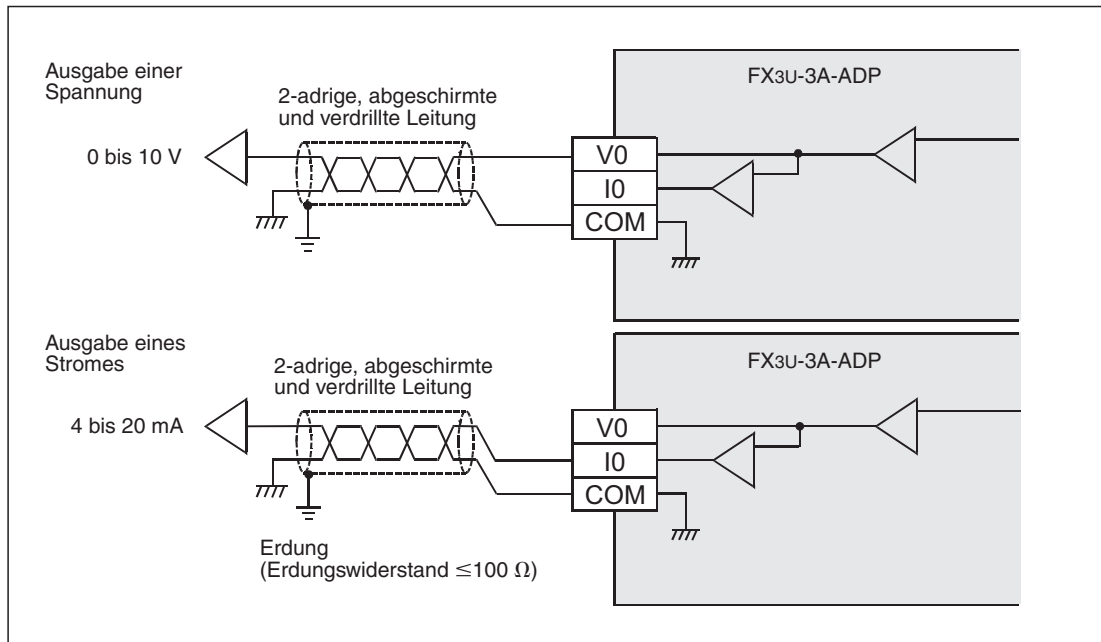
Abb. 9-11: Anschluss des analogen Ausgangssignals an ein Adaptermodul FX3U-3A-ADP
