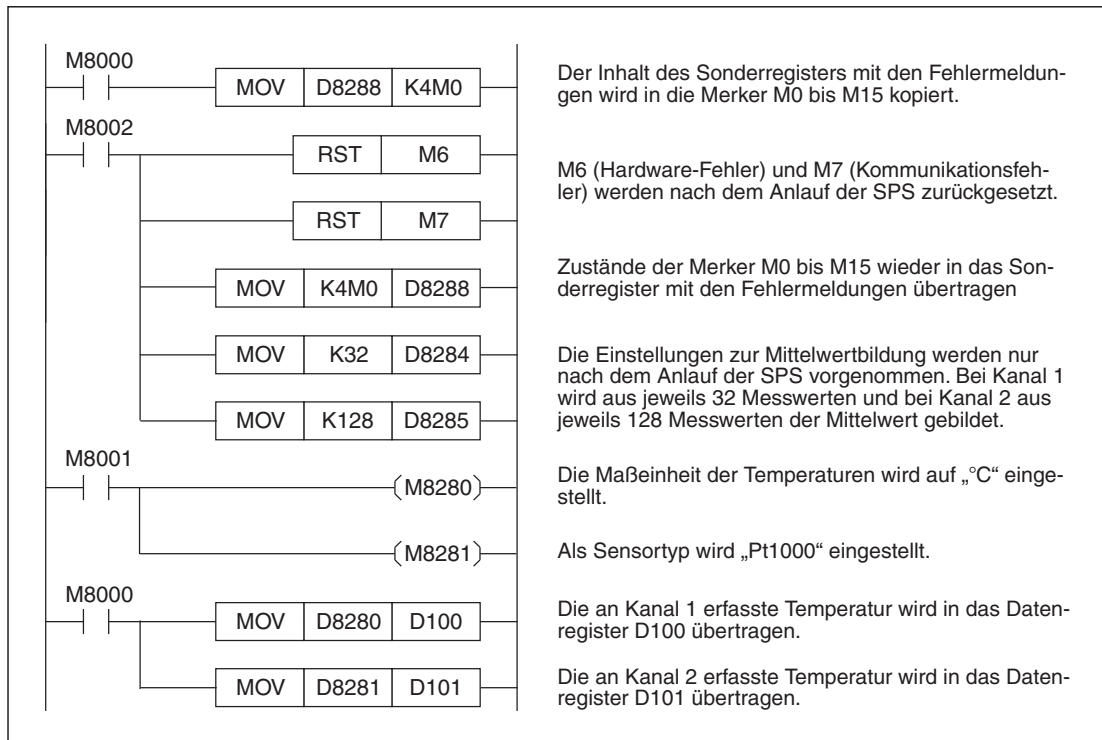
Abb. 12-24: Beispielprogramm zur Konfiguration von Kanal 1 und Kanal 2 eines FX3U-4AD-PNK-ADP
