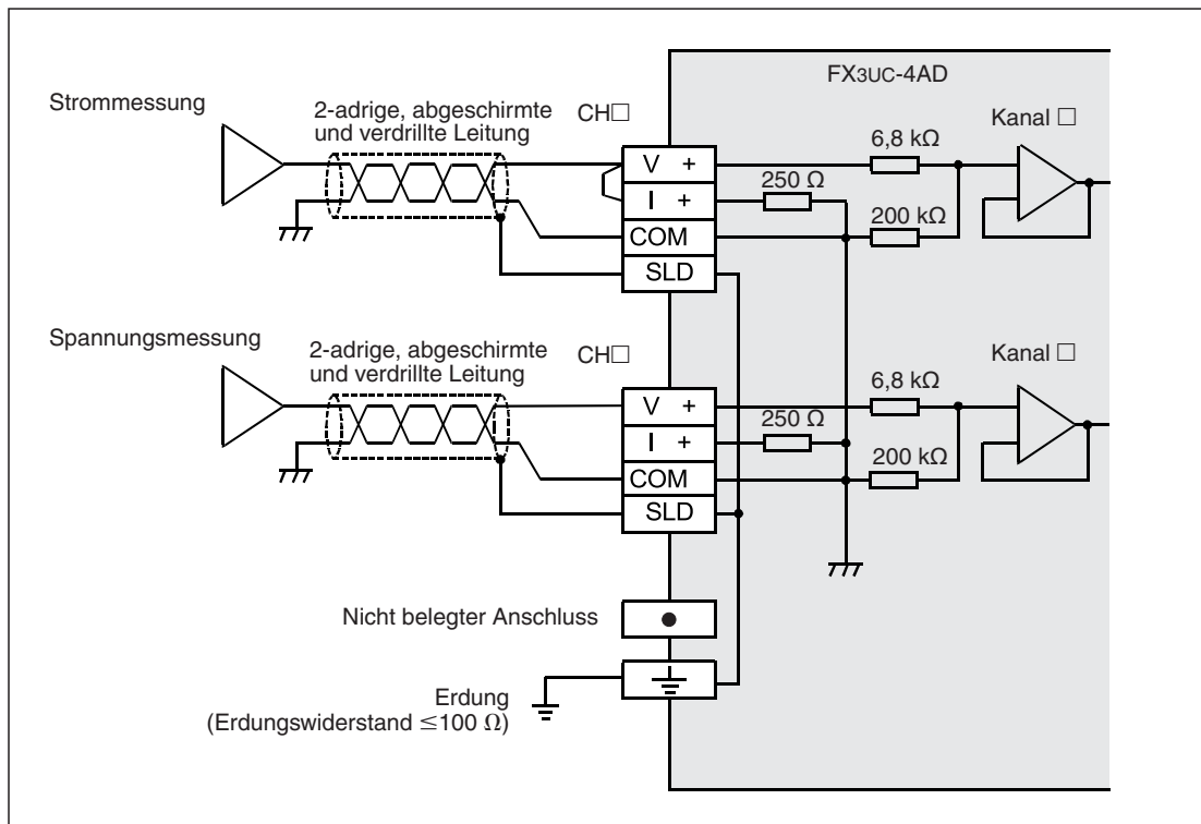
Abb. 5-18: Anschluss der analogen Signale an ein Analogeingangsmodul FX3UC-4AD
