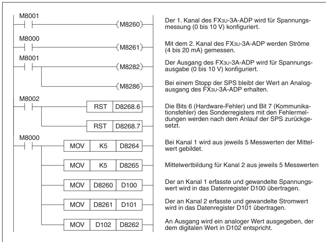
Abb. 9-28: Beispielprogramm zum Messen und zur Ausgabe von Analogwerten mit einem FX3U-3A-ADP, das als 1. analoges Adaptermodul installiert ist.
