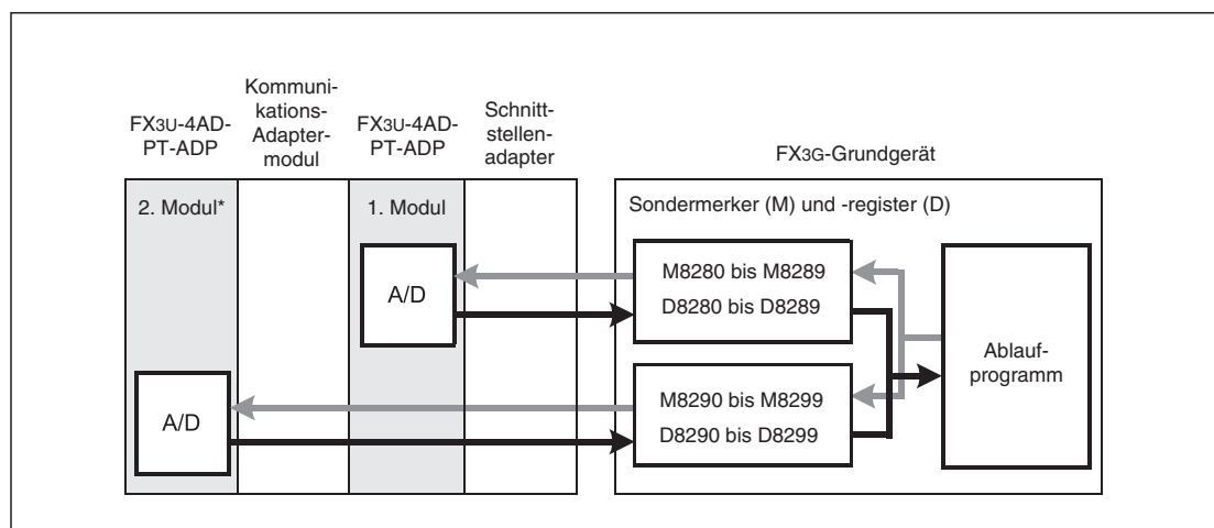
Abb. 10-11: Datenaustausch eines FX3G-Grundgeräts mit analogen Adaptermodulen
