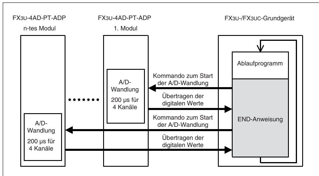
Abb. 10-2: Prinzip der Messwerterfassung bei FX3U- und FX3UC-Grundgeräten
