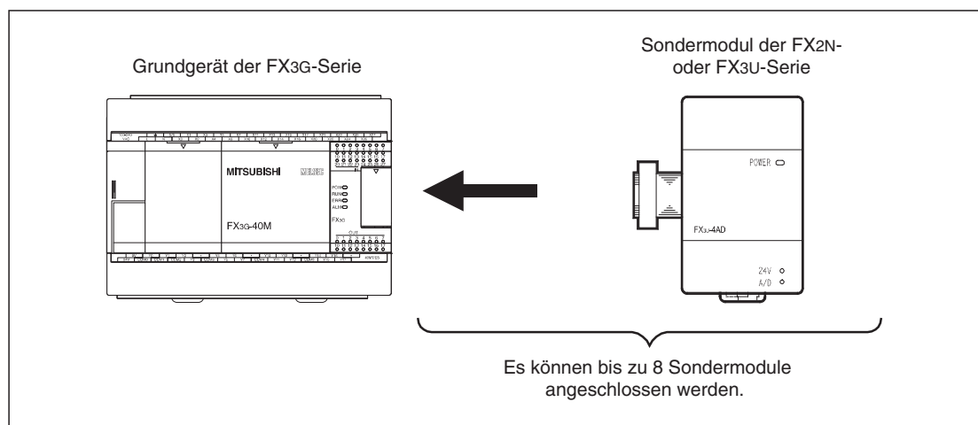
Abb. 1-8: Sondermodule werden an ein FX3G-Grundgerät direkt angeschlossen
