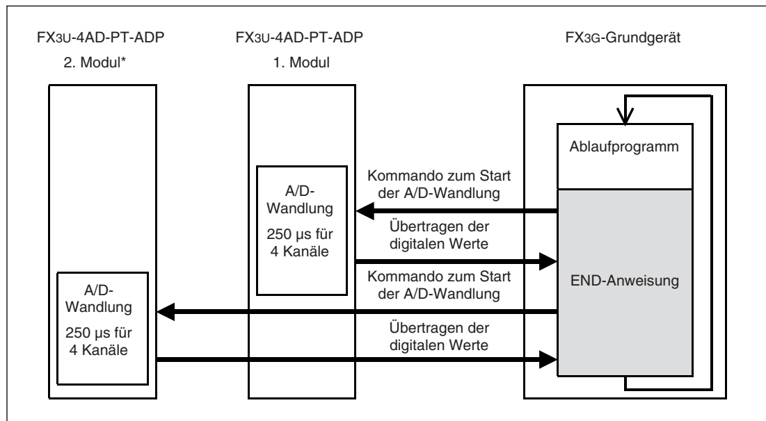
Abb. 10-1: Prinzip der Messwertverarbeitung bei FX3G-Grundgeräten (Maximal können zwei FX3U-4AD-PT-ADP angeschlossen werden).
