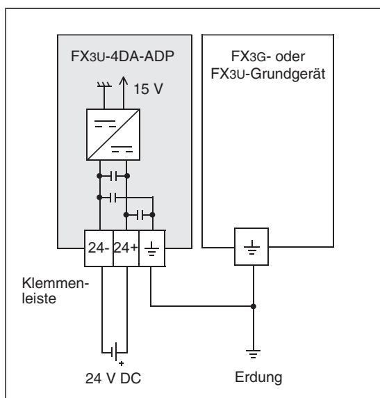
Abb. 7-6: Versorgung des FX3U-4DA-ADP aus einer separaten Spannungsquelle
