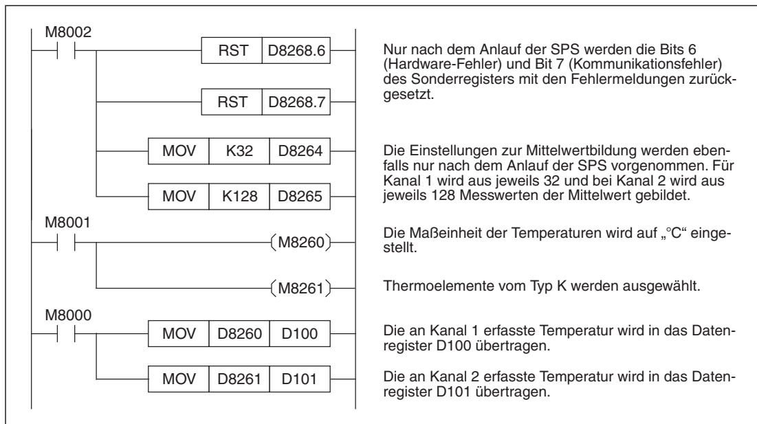
Abb. 13-25: Beispielprogramm zur Konfiguration von Kanal 1 und Kanal 2 eines FX3U-4AD-TC-ADP, das als 1. analoges Adaptermodul installiert ist.
