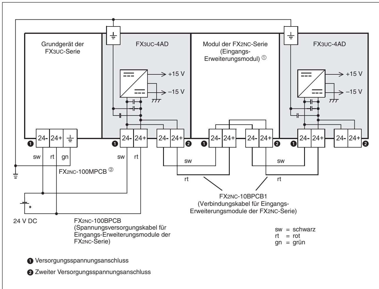
Abb. 5-15: Anschluss der Versorgungsspannung eines FX3UC-4AD
