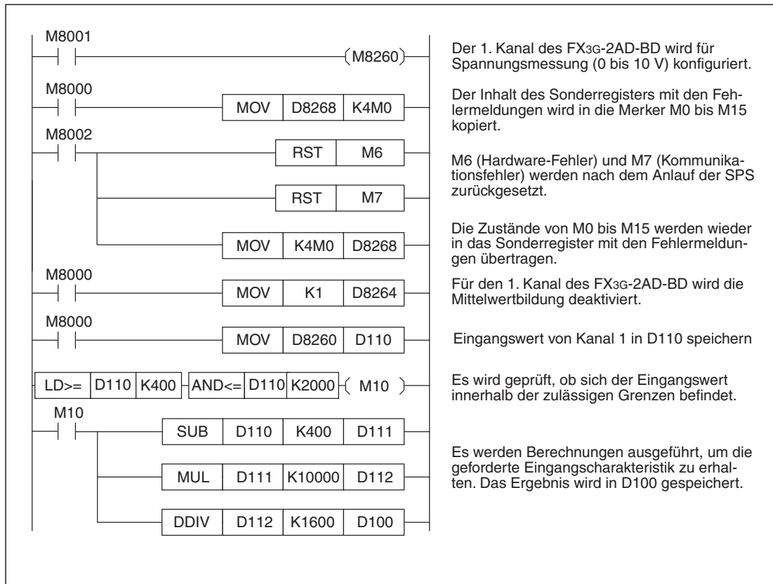
Abb. 3-16: Programmbeispiel zur Änderung der Charakteristik eines Spannungseingangs
