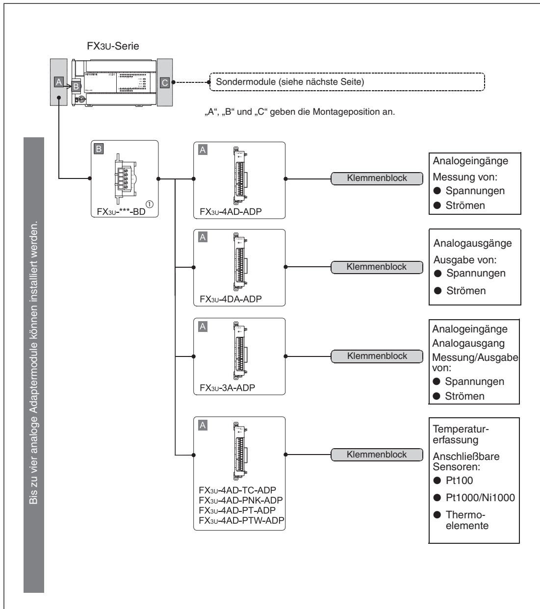
Abb. 1-14: Anschluss von analogen Adaptermodulen an ein Grundgerät der FX3U-Serie
