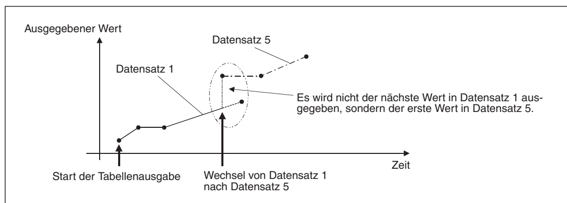
Abb. 8-31: Beispiel für den Wechsel von Datensätzen während der Tabellenausgabe
