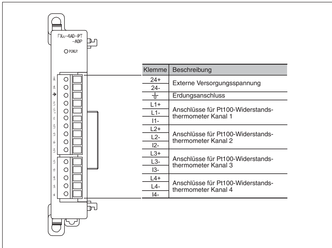
Abb. 10-5: Klemmenbelegung des FX3U-4AD-PT-ADP
