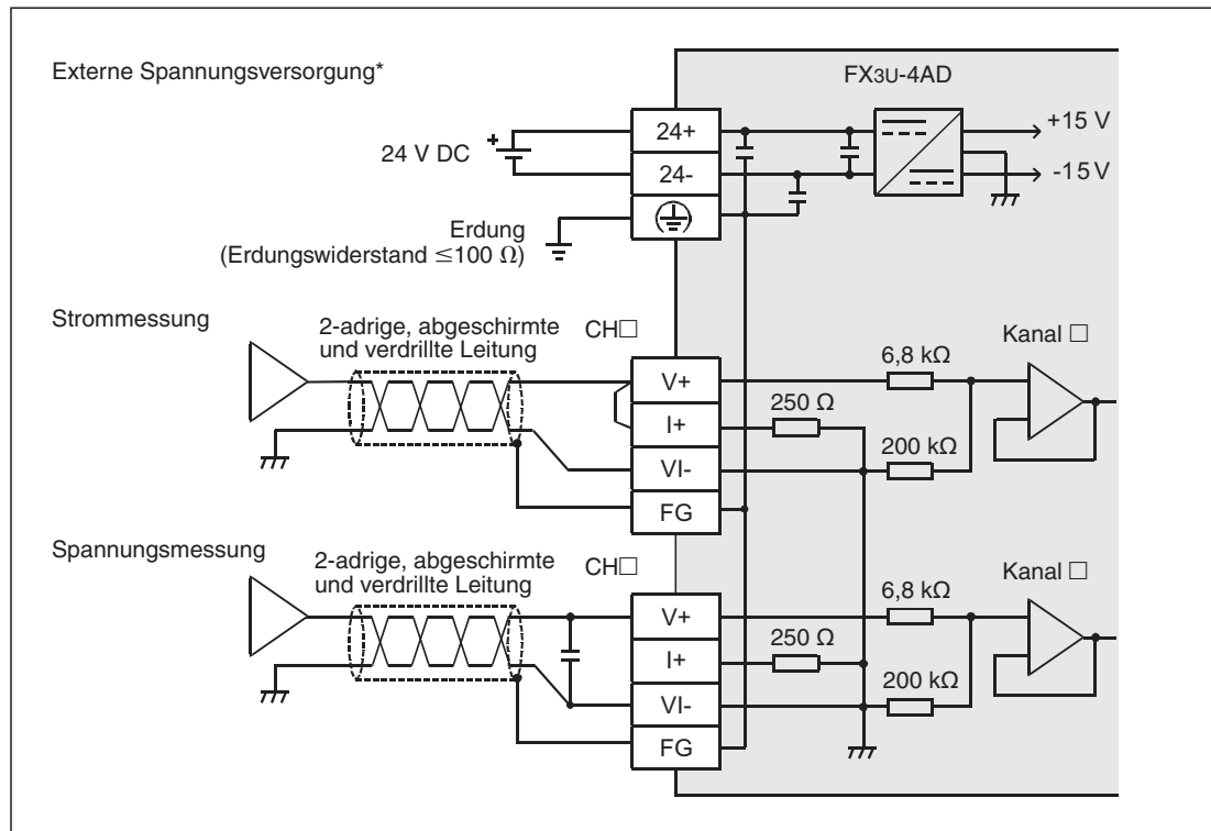
Abb. 5-17: Anschluss der analogen Signale an ein Analogeingangsmodul FX3U-4AD
