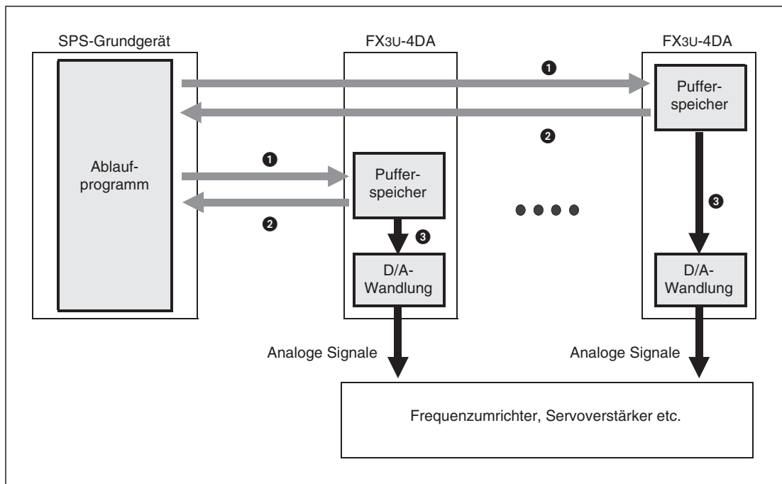
Abb. 8-13: Prinzip des Datenaustausches zwischen SPS-Grundgerät und Sondermodulen
