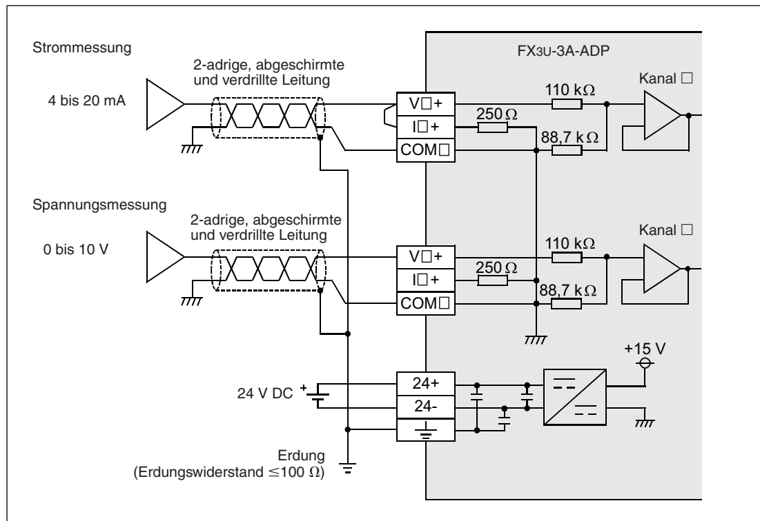
Abb. 9-10: Anschluss der analogen Eingangssignale an ein Adaptermodul FX3U-3A-ADP
