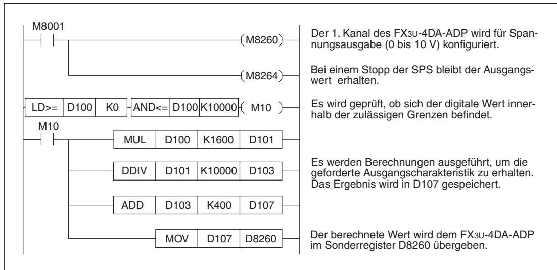
Abb. 7-23: Programmbeispiel zur Änderung der Charakteristik eines Spannungsausgangs
