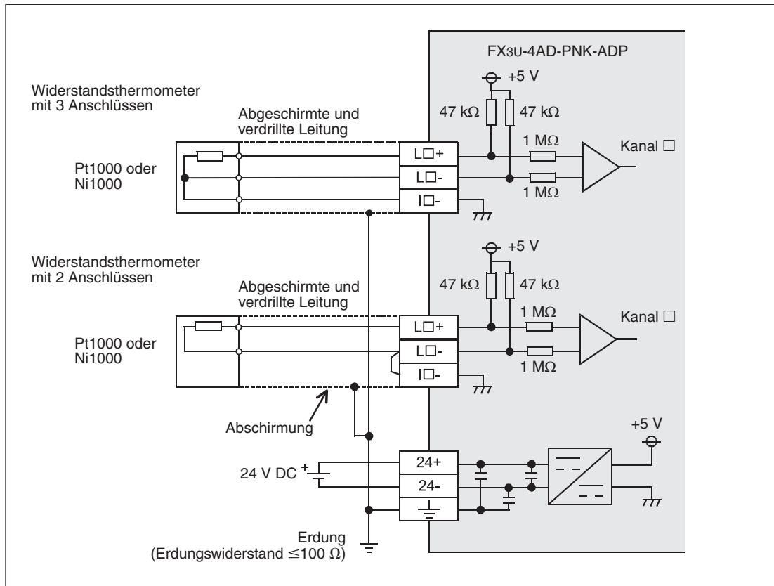
Abb. 12-10: Anschluss der Widerstandsthermometer an ein Temperaturerfassungs-Adaptermodul FX3U-4AD-PNK-ADP
