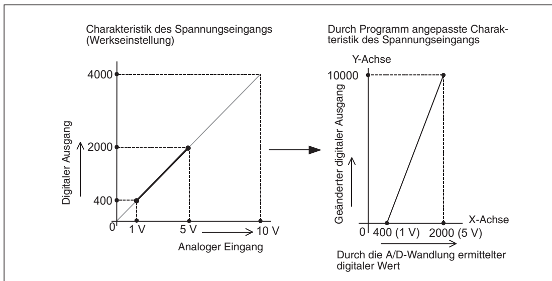
Abb. 3-15: In diesem Beispiel wird durch Anweisungen im Ablaufprogramm der Anfangspunkt und die Steigung einer Geraden verändert.
