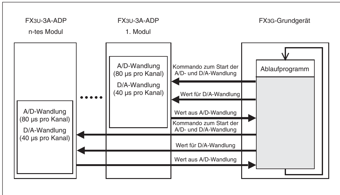
Abb. 9-2: Prinzip der Messwerterfassung und Analogwertausgabe bei FX3U- und FX3UC-Grundgeräten.
