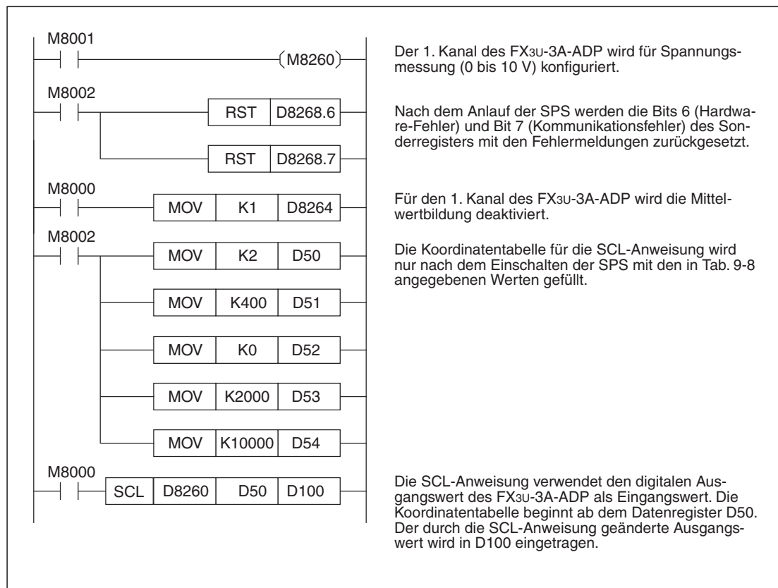
Abb. 9-31: Programmbeispiel zur Änderung der Charakteristik eines Spannungseingangs durch eine SCL-Anweisung
