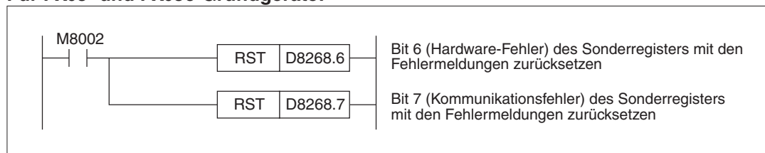
Abb. 13-21: Beispiel zum Zurücksetzen der Fehlermeldungen des FX3U-4AD-TC-ADP, das als 1. analoges Adaptermodul installiert ist.
