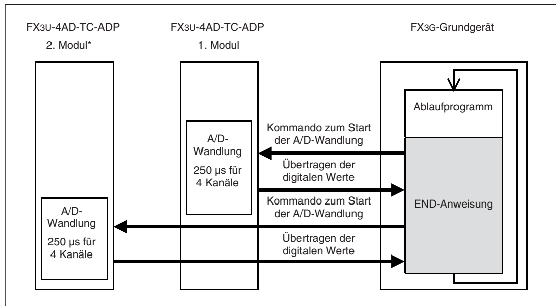
Abb. 13-1: Prinzip der Messwerterfassung bei FX3G-Grundgeräten (Maximal können zwei FX3U-4AD-TC-ADP angeschlossen werden).
