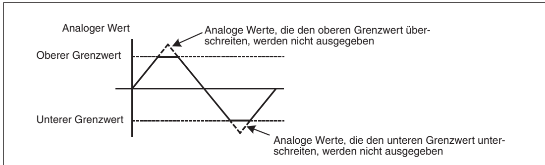
Abb. 8-21: Die Ausgabe des Analogwerts wird bei einer Grenzwertüberschreitung begrenzt
