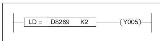
Abb. 7-18: Wenn als 1. analoges Adaptermodul ein FX3U-4DA-ADP installiert ist, wird der Ausgang Y005 eingeschaltet.
