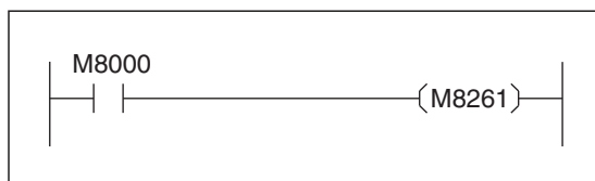
Abb. 3-8: Der 2. Kanal des FX3G-2AD-BD, das auf dem 1. Erweiterungssteckplatz installiert ist, wird für Strommessung konfiguriert. Der Merker M8000 ist immer „1“.
