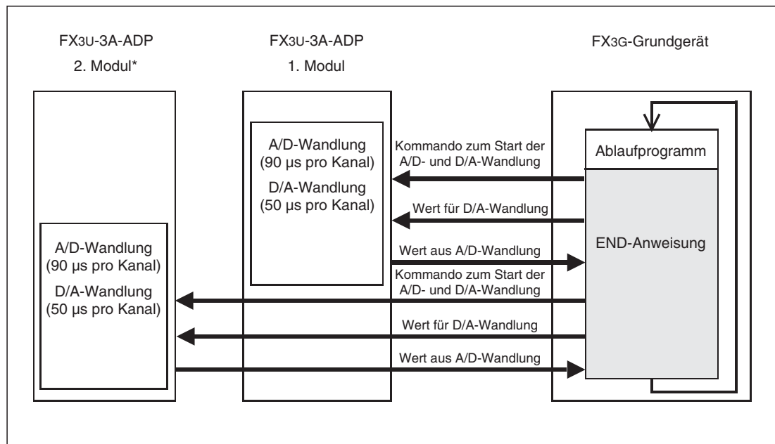
Abb. 9-1: Prinzip der Messwerterfassung und Analogwertausgabe bei FX3G-Grundgeräten (Maximal können zwei FX3U-3A-ADP angeschlossen werden).
