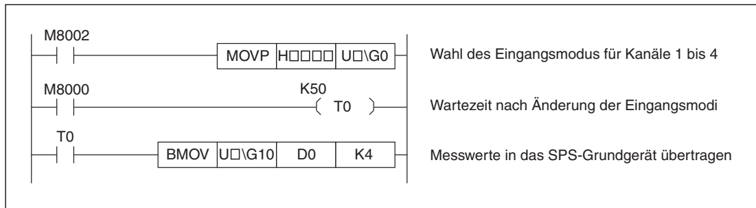
Abb. 5-29: Zur Einstellung der Eingangsmodi und zum Lesen der Messwerte genügen drei Anweisungen.
