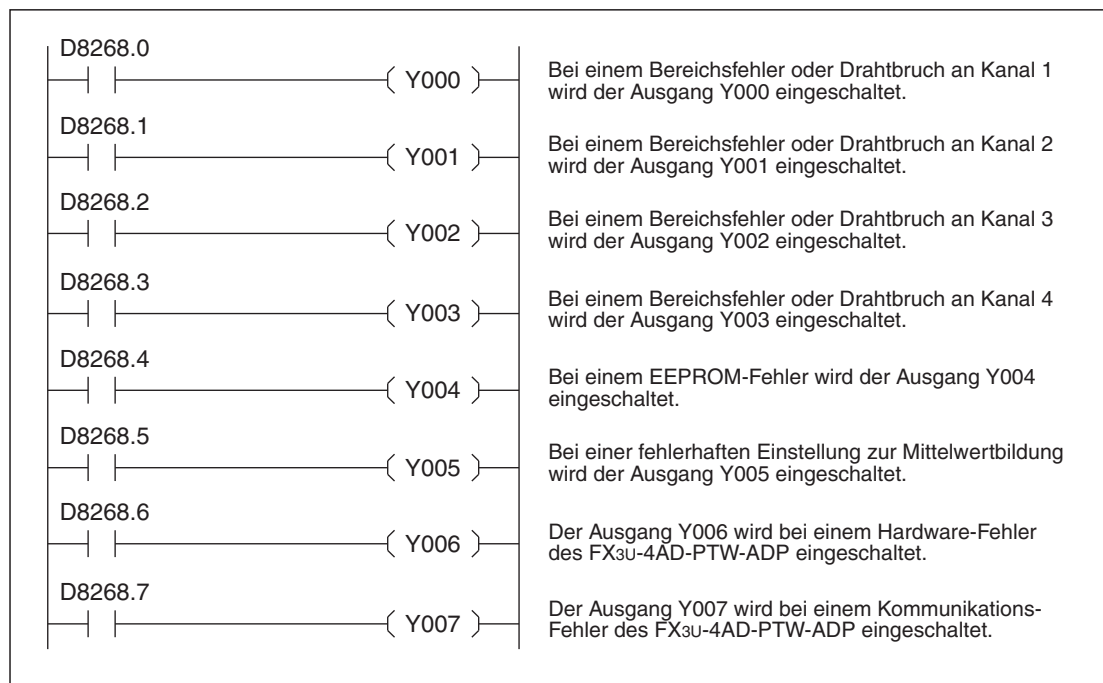
Abb. 11-20: Beispiel zur Auswertung von Fehlermeldungen eines FX3U-4AD-PTW-ADP, das als 1. analoges Adaptermodul installiert ist.
