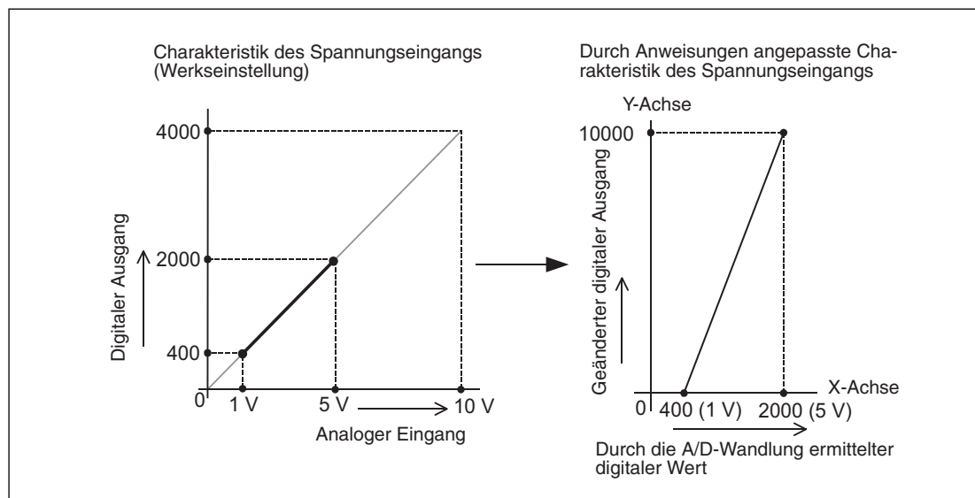
Abb. 9-29: In diesem Beispiel wird durch Anweisungen im Programm der Anfangspunkt und die Steigung einer Geraden verändert.
