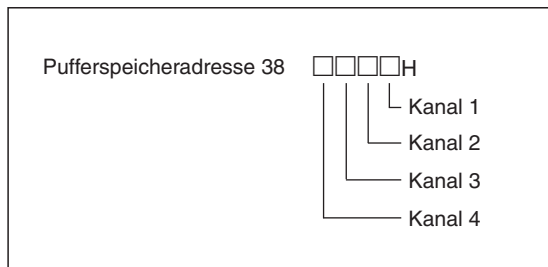
Abb. 8-19: Zuordnung der 4-Bit-Gruppen zu den einzelnen Kanälen
