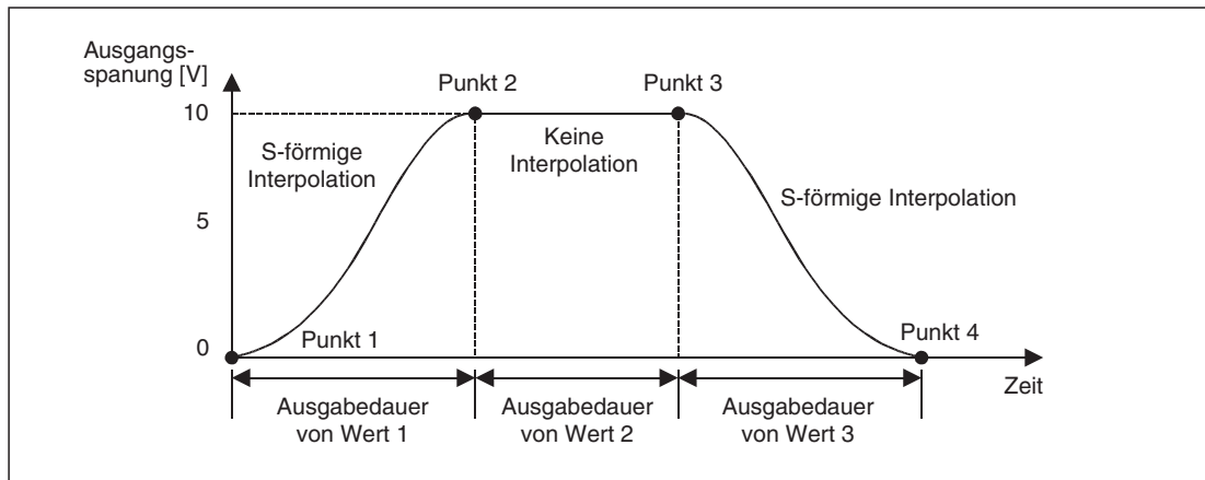
Abb. 8-26: Realisierung der Funktion durch eine Tabelle mit 4 Werten im Analogausgangsmodul FX3U-4DA, mit denen die Ausgangsspannung des Moduls gesteuert wird.
