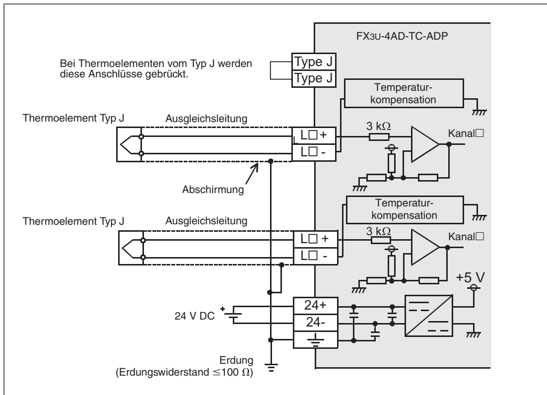
Abb. 13-11: Anschluss von Thermoelementen des Typs J an ein Temperaturerfassungs-Adaptermodul FX3U-4AD-TC-ADP; Die Klemmen „Type J“ werden gebrückt.
