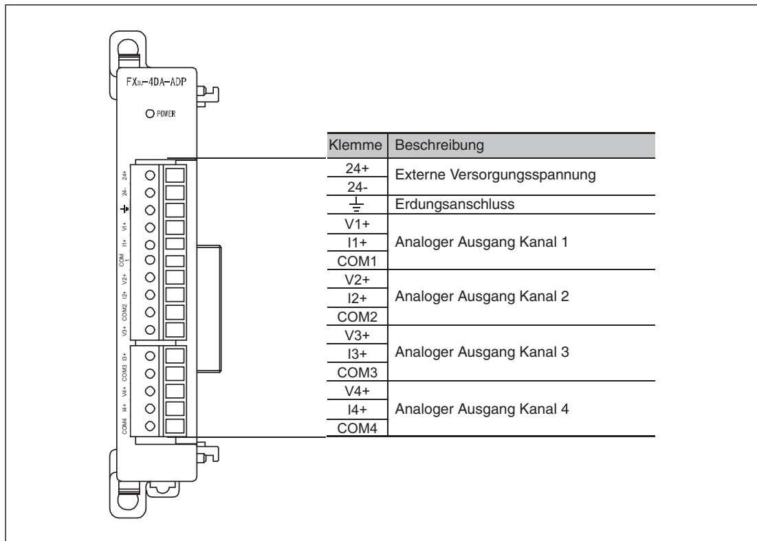
Abb. 7-5: Klemmenbelegung des FX3U-4DA-ADP
