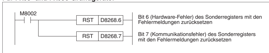
Abb. 4-18: Beispiel zum Zurücksetzen der Fehlermeldungen des FX3U-4AD-ADP, das als 1. analoges Adaptermodul installiert ist.
