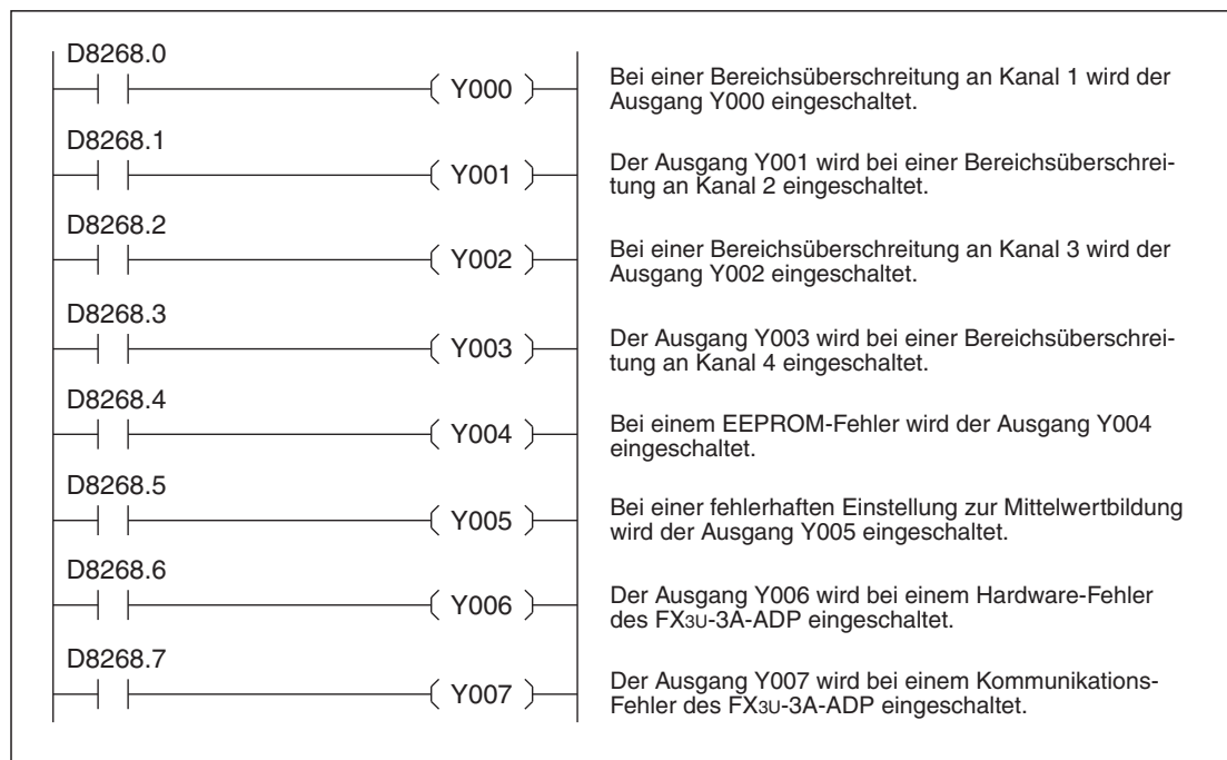
Abb. 9-25: Beispiel zur Auswertung von Fehlermeldungen eines FX3U-3A-ADP, das als 1. analoges Adaptermodul installiert ist.
