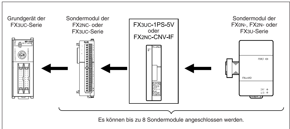
Abb. 1-10: Anschluss von Sondermodulen an ein FX3UC-Grundgerät
