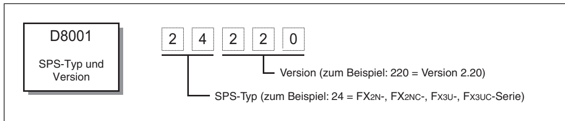
Abb. 1-19: Angabe der Version des Grundgeräts im Sonderregister D8001
