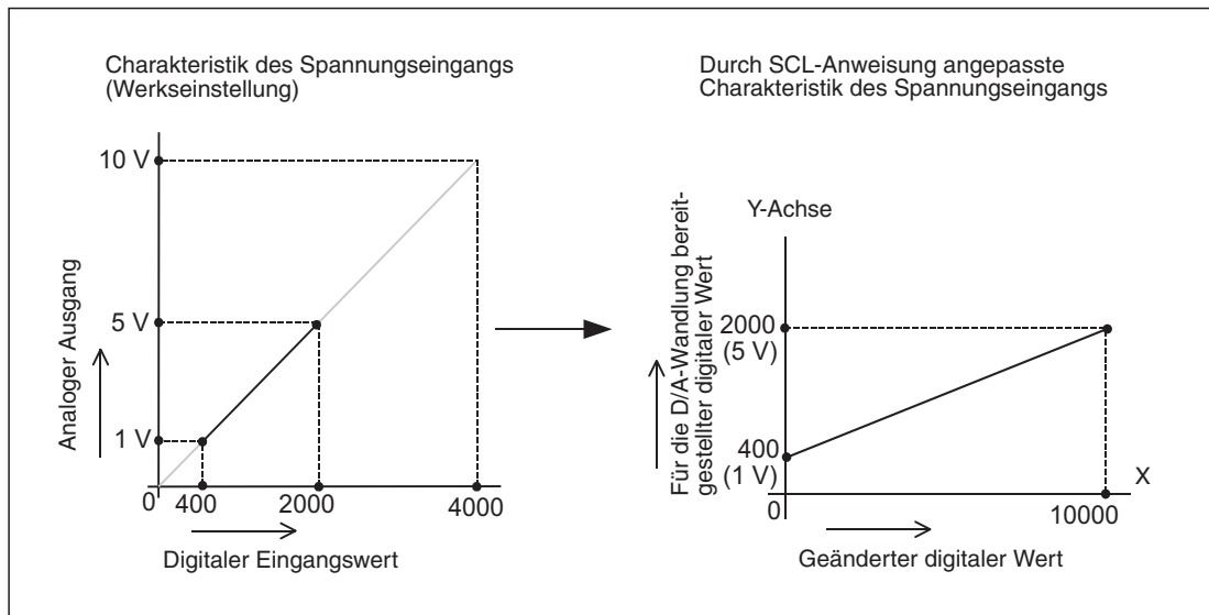
Abb. 6-13: In diesem Beispiel wird durch Anweisungen im Ablaufprogramm der Anfangspunkt und die Steigung einer Geraden verändert.
