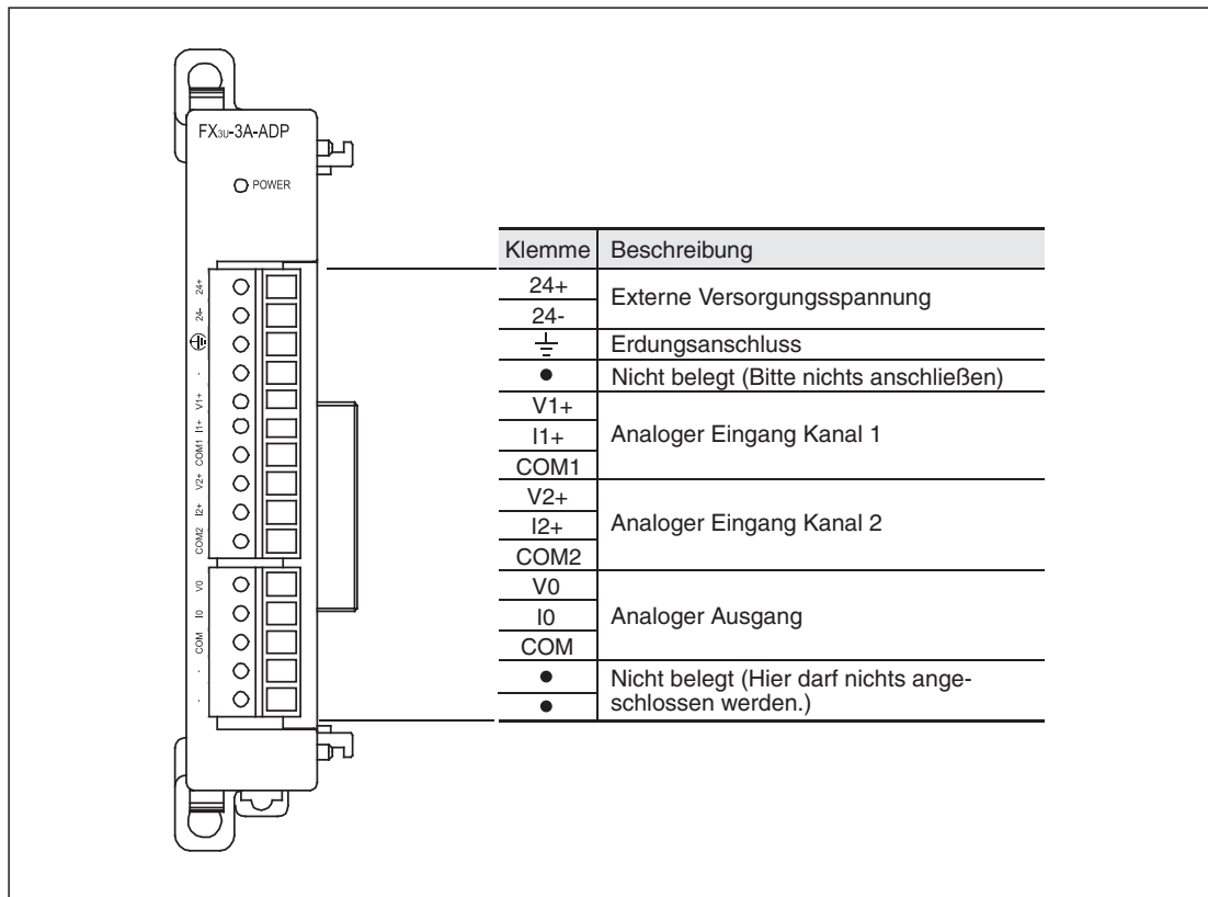
Abb. 9-5: Klemmenbelegung des FX3U-3A-ADP
