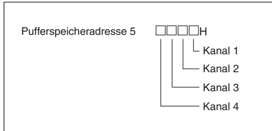
Abb. 8-15: Zuordnung der 4-Bit-Gruppen zu den einzelnen Kanälen
