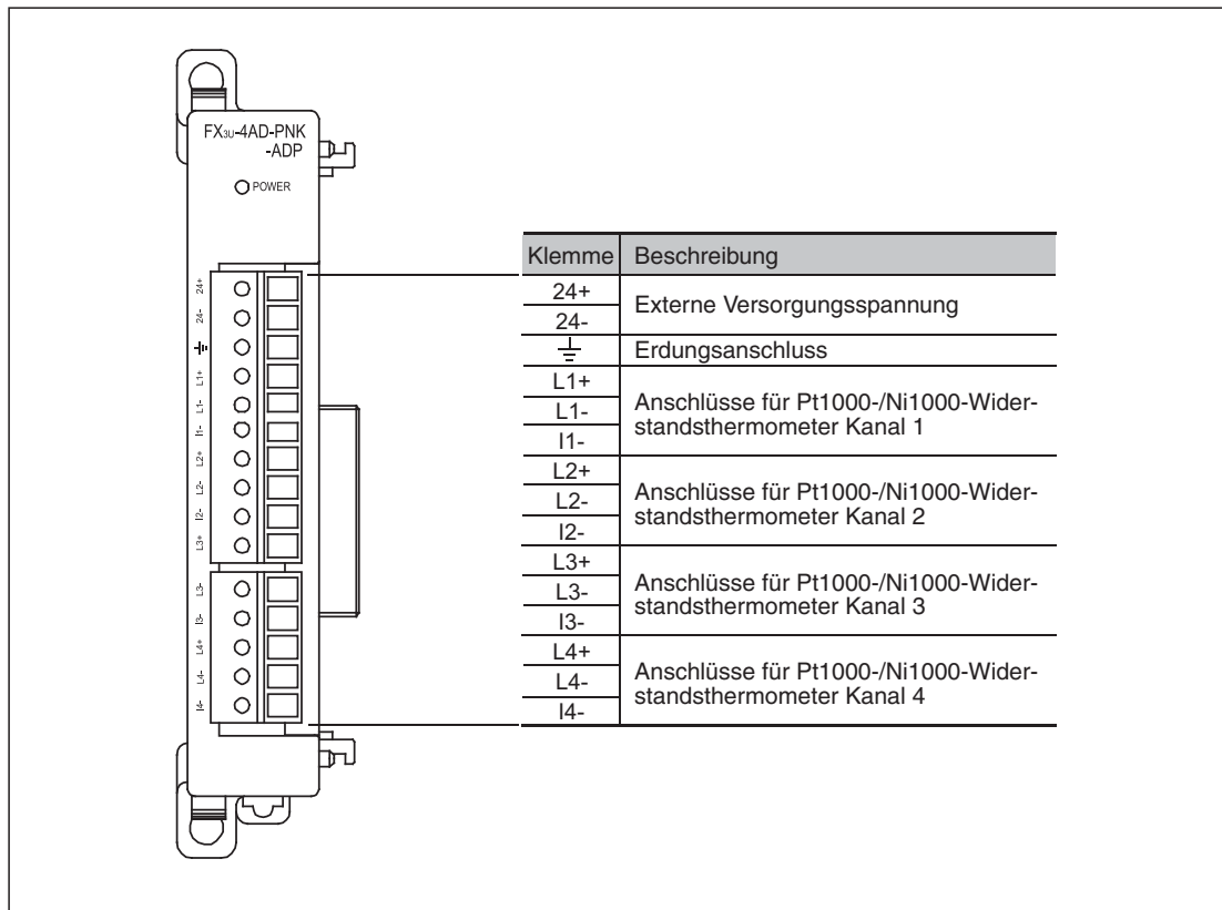
Abb. 12-5: Klemmenbelegung des FX3U-4AD-PNK-ADP
