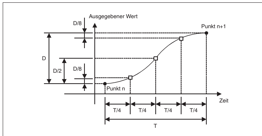
Abb. 8-28: S-förmige Interpolation
