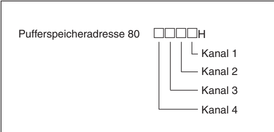
Abb. 8-32: Zuordnung der 4-Bit-Gruppen zu den einzelnen Kanälen
