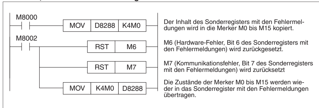
Abb. 12-19: Beispiel zum Zurücksetzen der Fehlermeldungen des FX3U-4AD-PNK-ADP, das als 3. analoges Adaptermodul (1. Modul bei FX3G) installiert ist.
