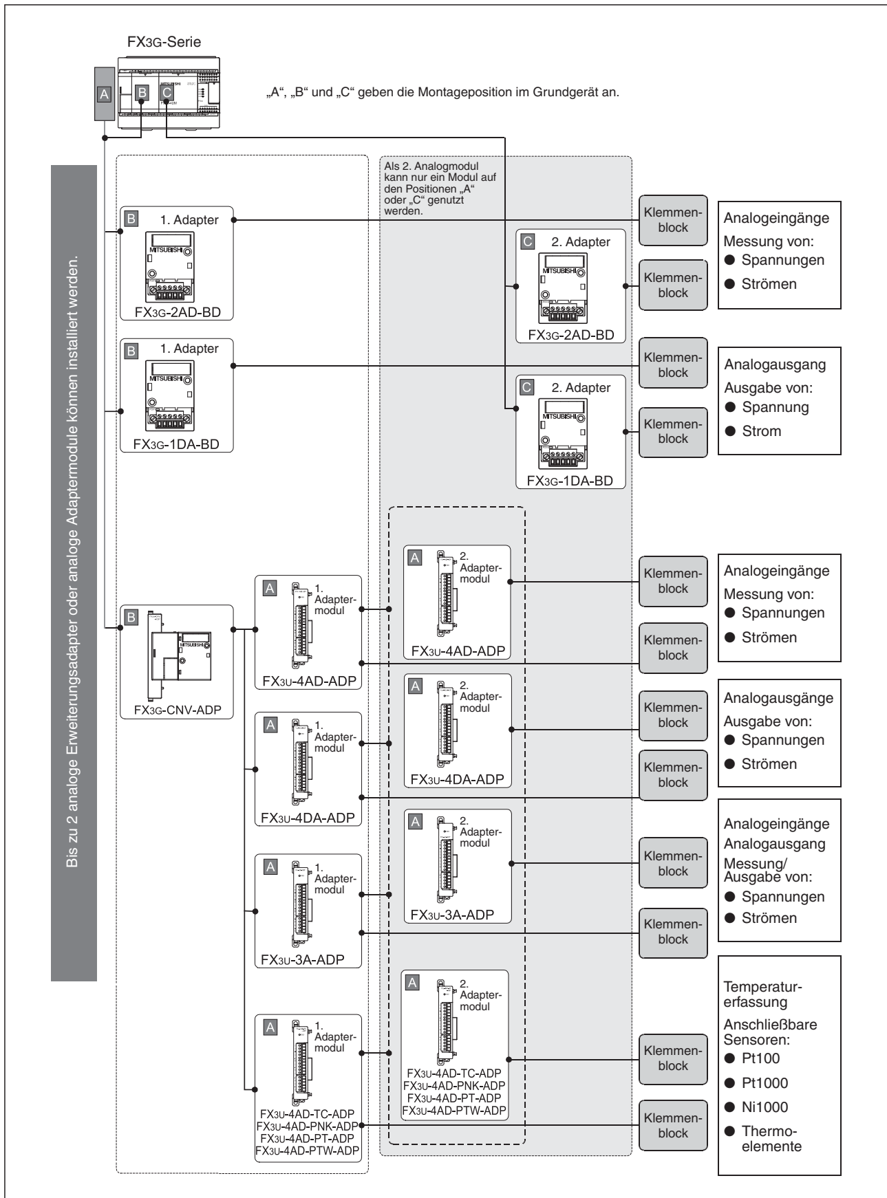
Abb. 1-12: Verwendbare Analogmodule für ein FX3G-Grundgerät mit 40 oder 60 Ein- und Ausgängen
