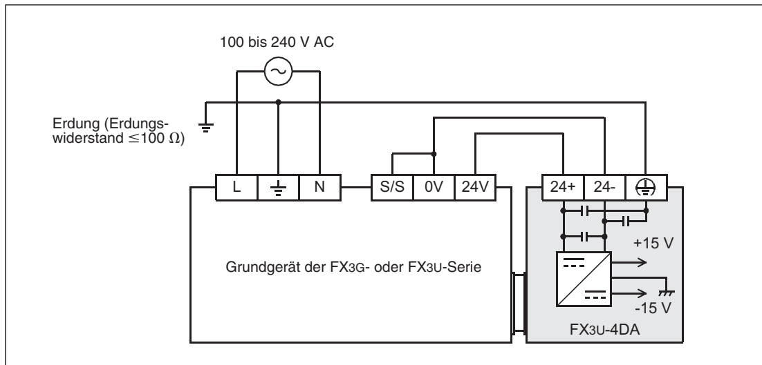
Abb. 8-9: Versorgung durch ein SPS-Grundgerät, das für plusschaltende Geber konfiguriert ist (Der Anschluss „S/S“ ist mit dem Anschluss „0V“ verbunden.)
