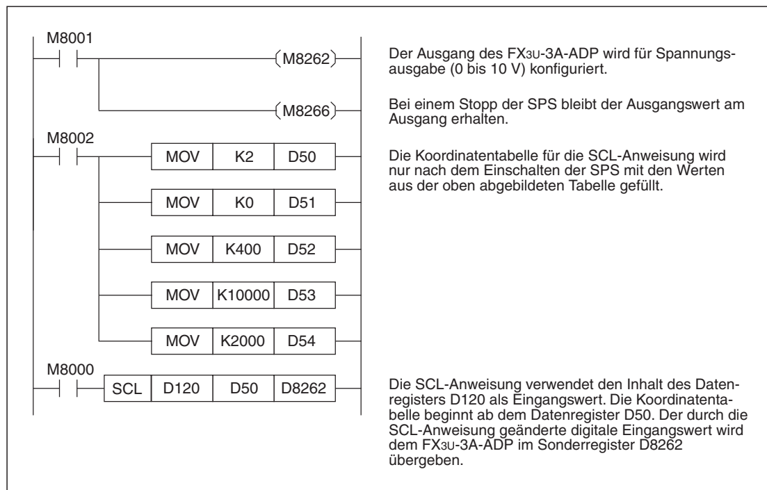
Abb. 9-34: Programmbeispiel zur Änderung der Charakteristik eines Spannungseingangs durch eine SCL-Anweisung
