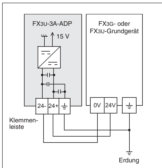
Abb. 9-6: Bei FX3G- und FX3U-Grundgeräten, die mit Wechselspannung versorgt werden, kann das FX3U-3A-ADP an die Servicespannungsquelle der SPS angeschlossen werden.
