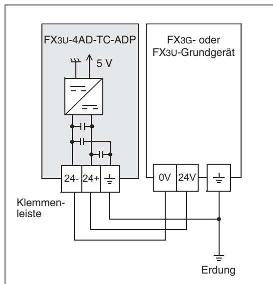
Abb. 13-6: Bei FX3G- und FX3U-Grundgeräten, die mit Wechselspannung versorgt werden, kann ein FX3U-4AD-TC-ADP auch an die Servicespannungsquelle der SPS angeschlossen werden.
