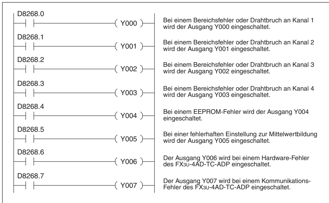
Abb. 13-: Beispiel zur Auswertung von Fehlermeldungen eines FX3U-4AD-TC-ADP
