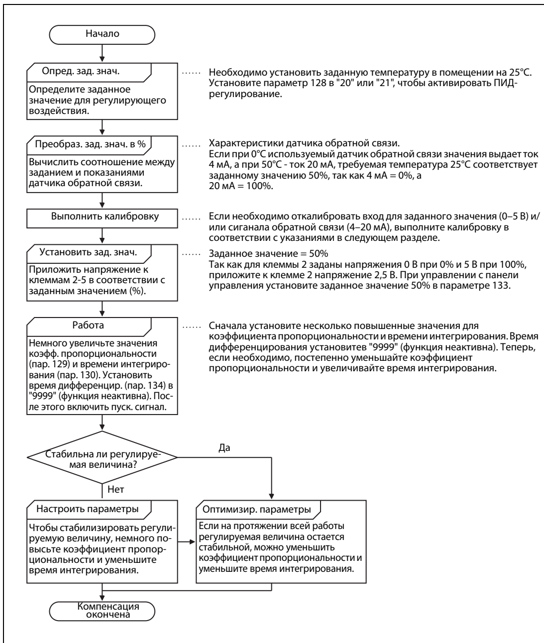
Рис. 6-141: Пример калибровки
