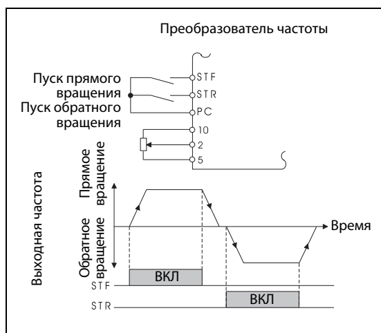
Рис. 6-55: Управление по 2-жильному проводу цепи управления (парам. 250 = 9999)
