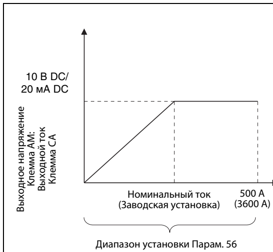
Рис. 6-73: Опорная величина для внешней индикации тока
