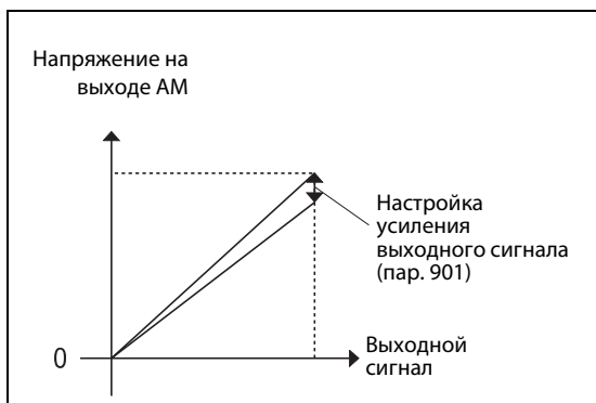
Рис. 6-76: Настройка усиления на выходе АМ
