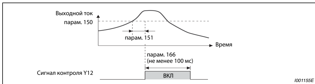
Рис. 6-63: Контроль выходного тока (Y12, парам. 166 ≠9999, парам. 167 = 0)
