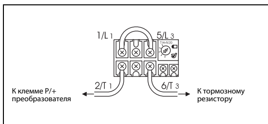
Рис. 3-21: Подключение Термореле
