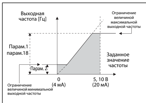
Рис. 6-10: Минимальная и максимальная выходная частота
