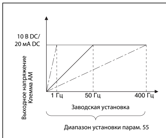
Рис. 6-72: Опорная величина для внешней индикации частоты
