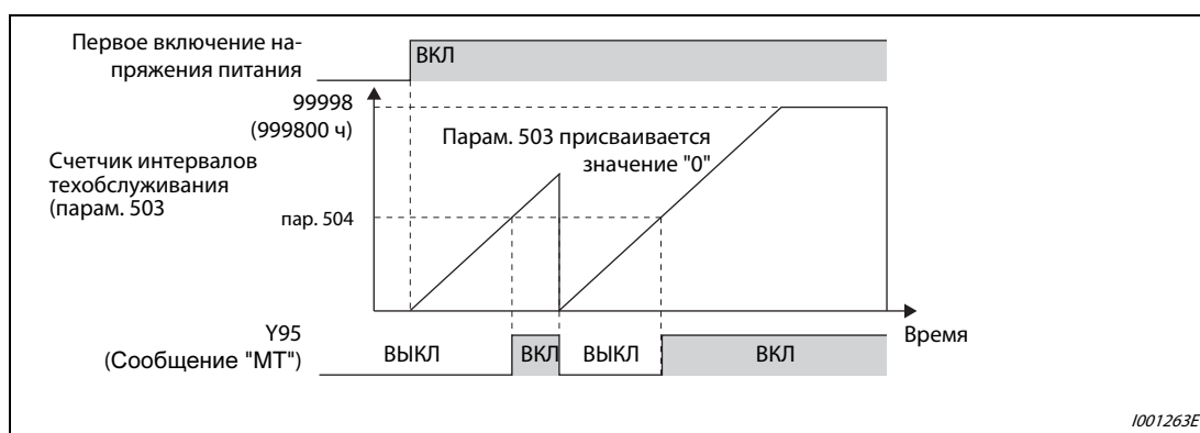
Рис. 6-153: Счетчик интервалов технического обслуживания
