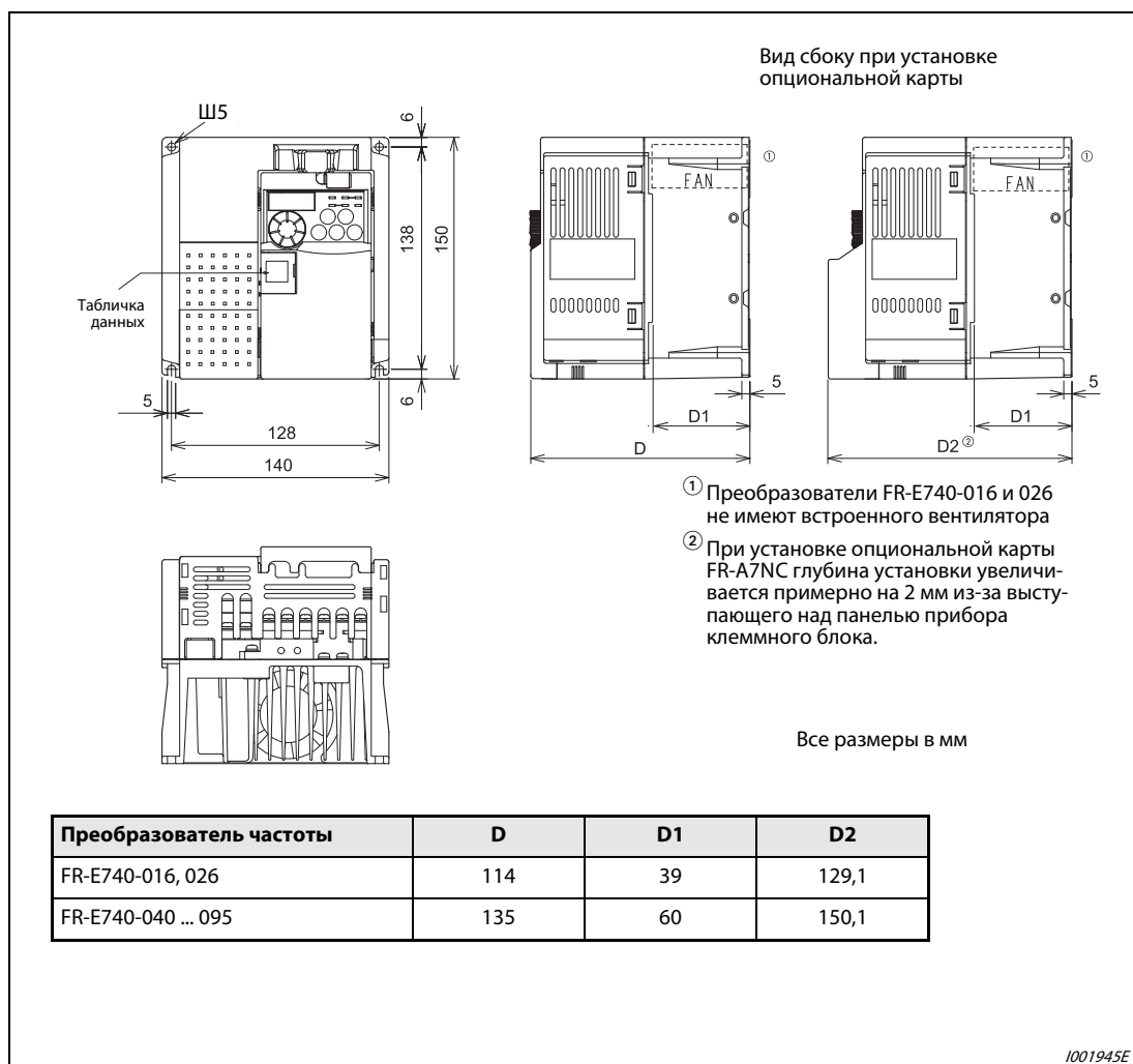
Рис. А-1: Размеры преобразователей частоты FR-E740-016...095
