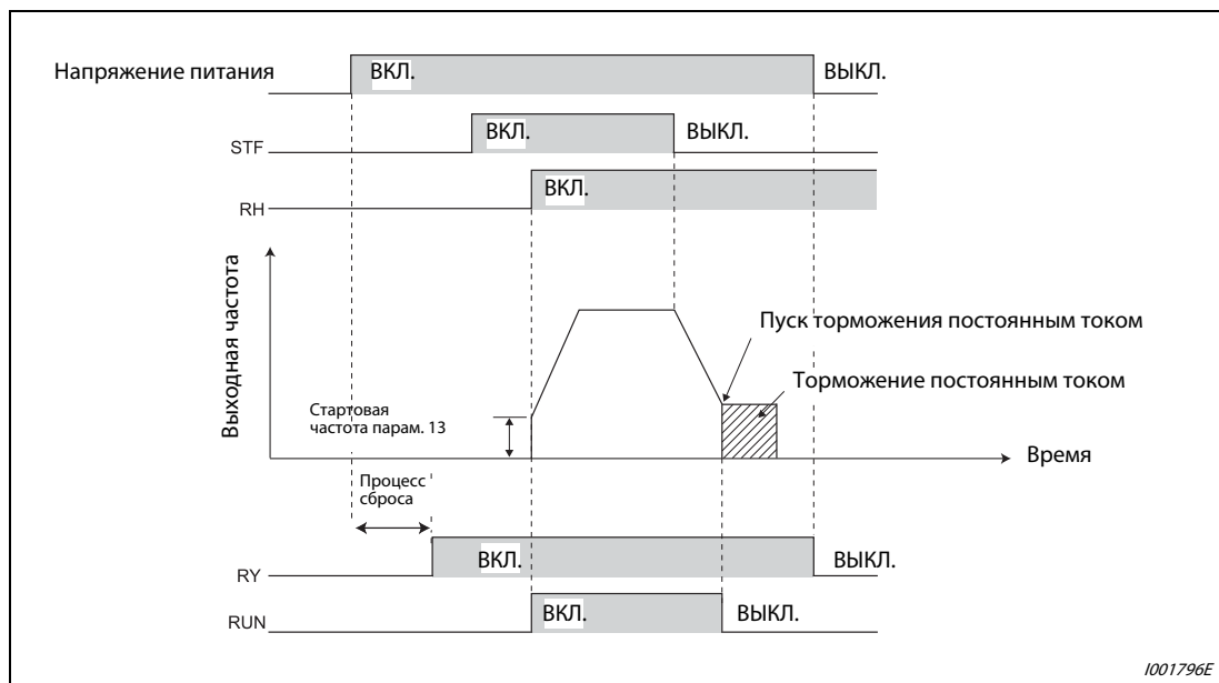
Рис. 6-59: Готовность к работе и работа двигателя
