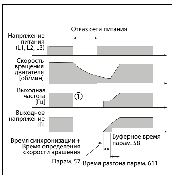
Рис. 6-79: Автоматический перезапуск с определением выходной частоты (парам. 162 = 0/10)
