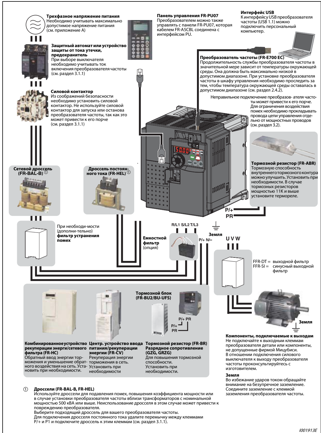
Рис. 3-1: Описание конфигурации системы
