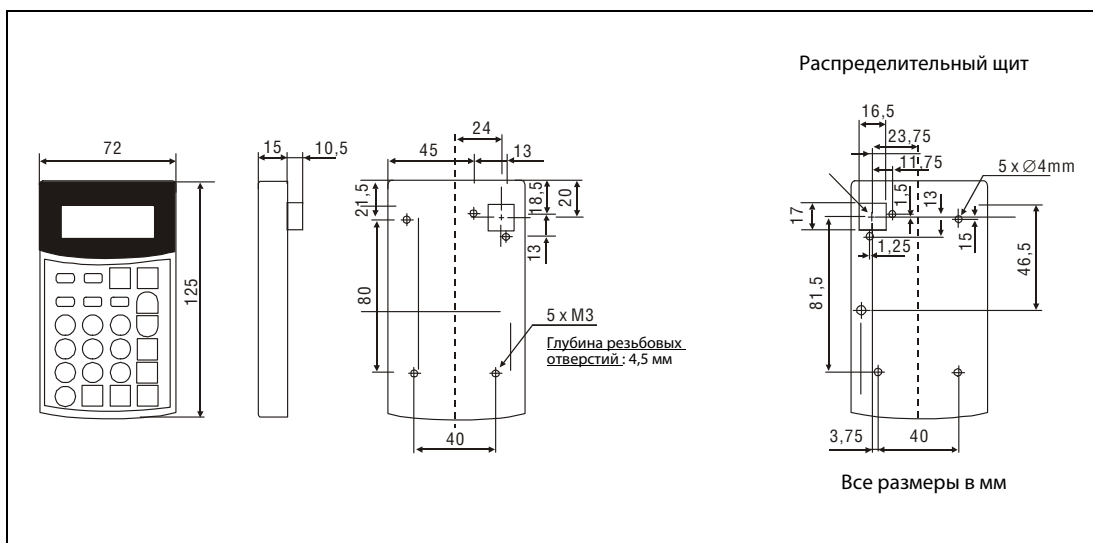
Рис. А-5: Пульт управления FR-PU04
