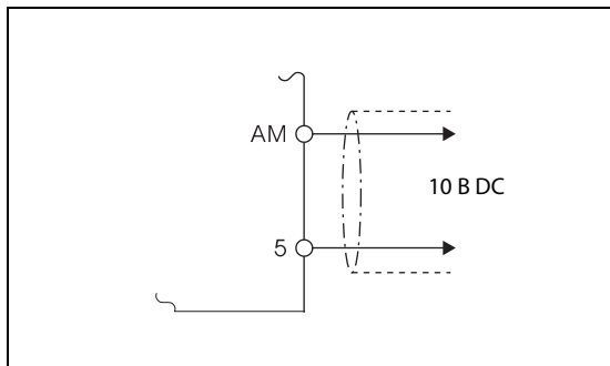
Рис. 6-75: Подключение аналогового индикатора к выходу АМ
