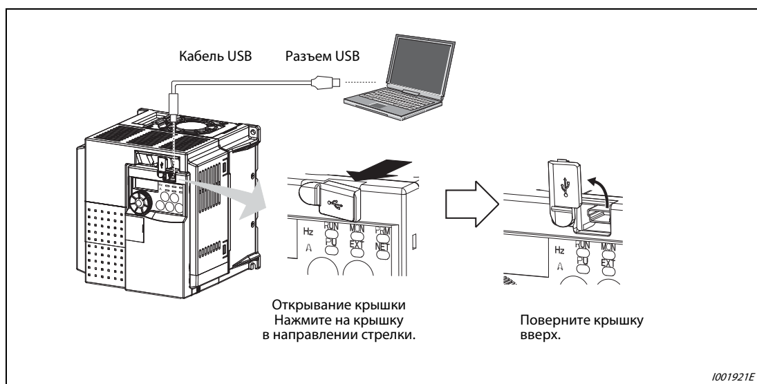
Рис. 6-131: Подключение к интерфейсу USB
