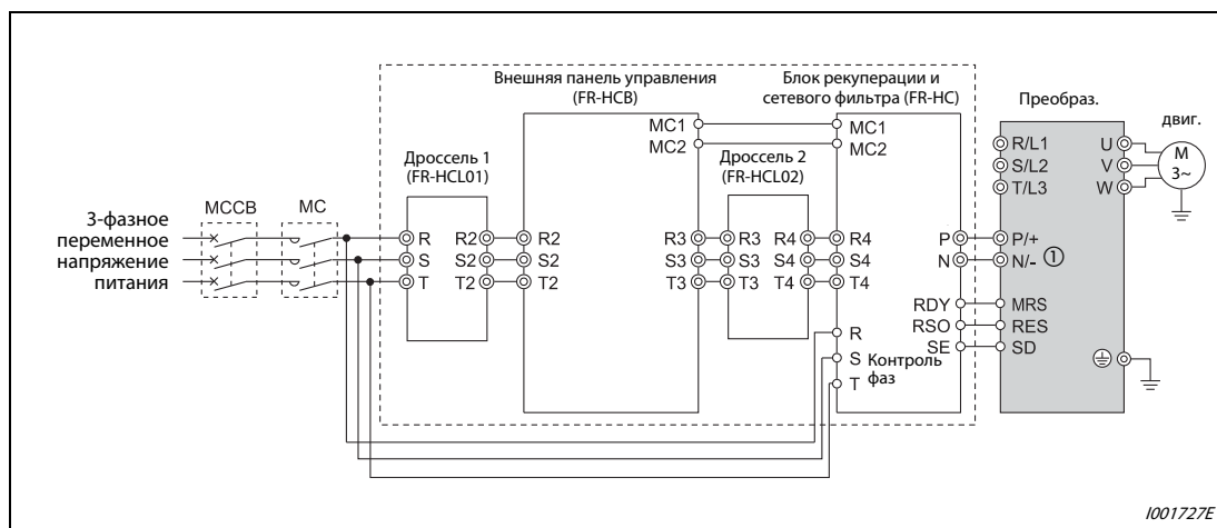
Рис. 3-24: Подключение комбинированного устройства рекуперации энергии/сетевого фильтра FR-NC
