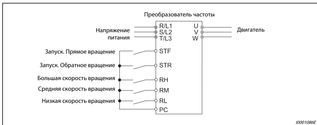
Рис. 5-23: Предустановка скорости вращения и ввод команды запуска при помощи переключателя
