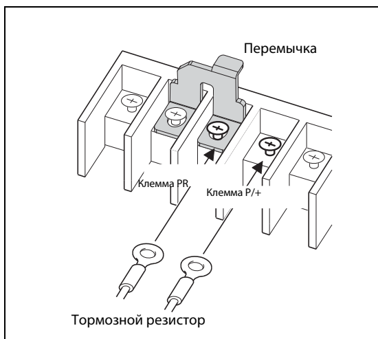
Рис. 3-19: Подключение тормозного резистора к клеммам P/+ и PR преобразователей частоты типов FR-E740-120 и FR-E740-300
