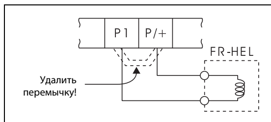
Рис. 3-26: Подключение дросселя постоянного тока
