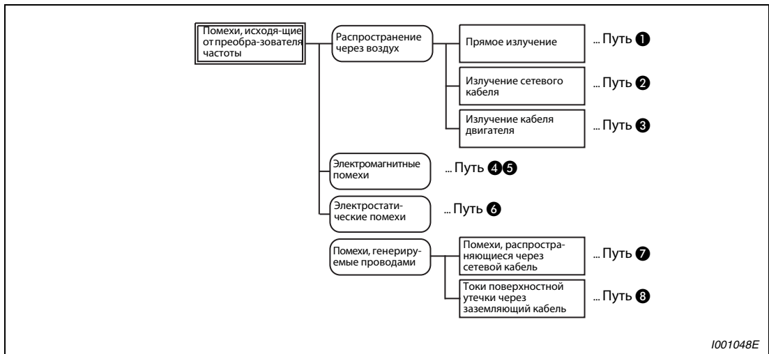
Рис. 3-30: Распространение помех
