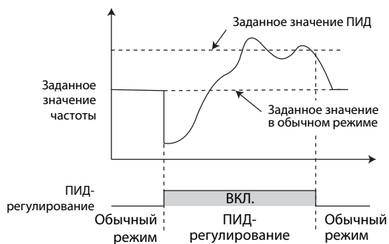
Работа при переключении с обычного режима на ПИД-регулирование
