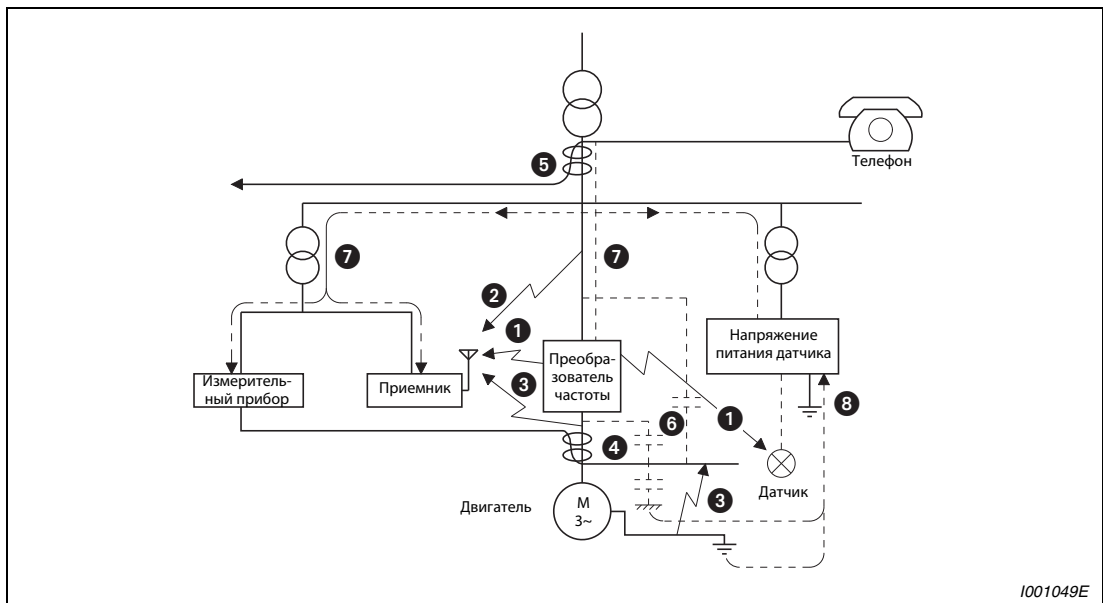
Рис. 3-31: Пути распространения помех
