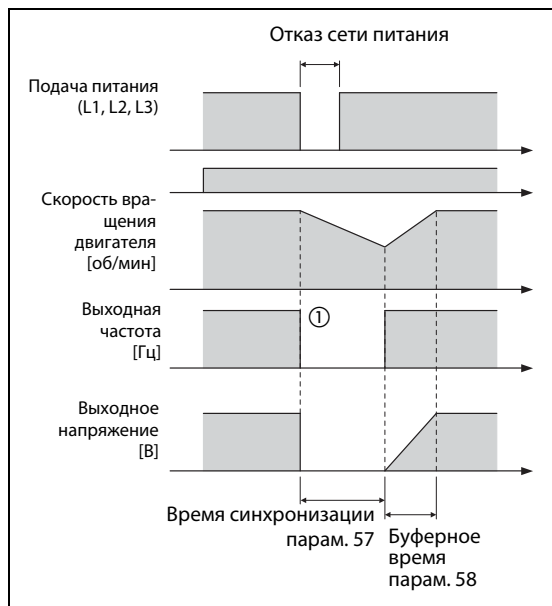
Рис. 6-78: Автоматический перезапуск без определения выходной частоты (парам. 162 = 1/11)
