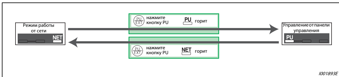
Рис. 6-103: Переключение режима работы при параметре 340 = 10 или 12
