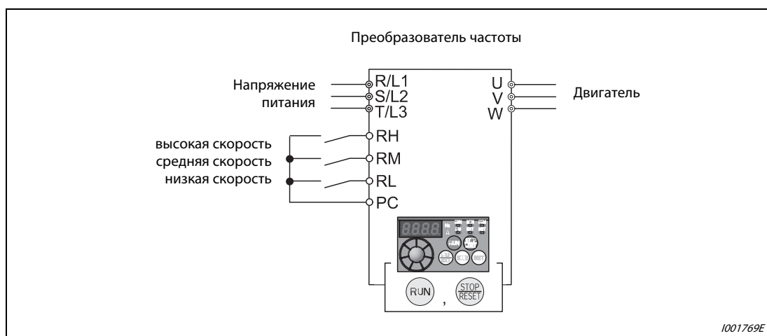
Рис. 5-14: Пример установки переключателей на клеммах RH, RM и RL
