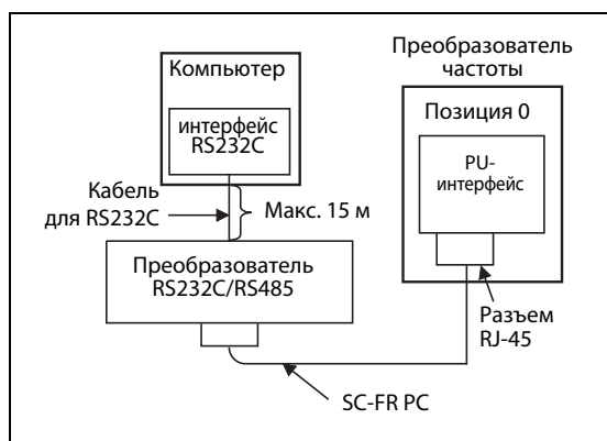
Рис. 6-111: Подключение компьютера с интерфейсом RS232 к интерфейсу PU
