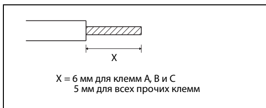
Рис. 3-7: Подготовка кабеля
