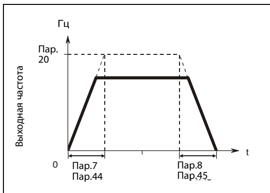
Рис. 6-29: Время разгона/замедления
