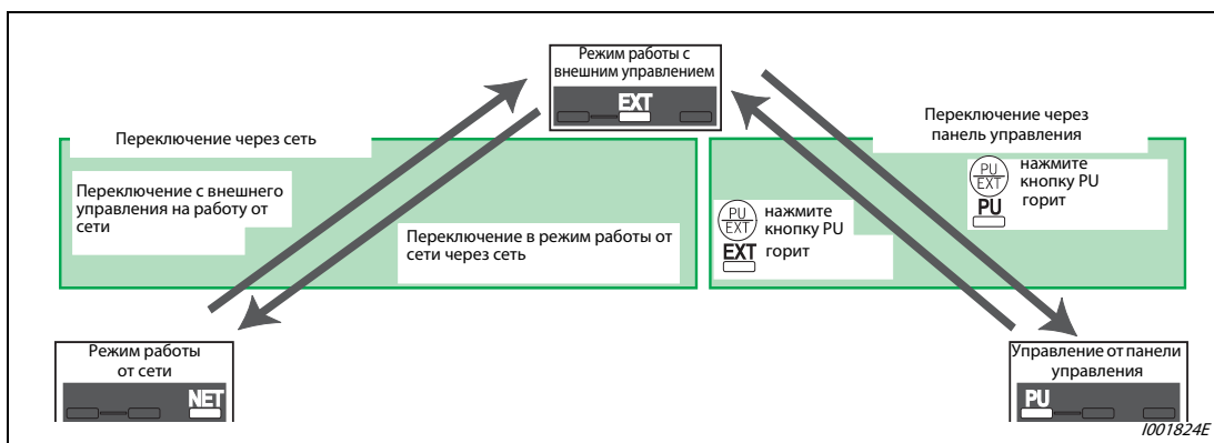
Рис. 6-102: Переключение режима работы при параметре 340 = 0, 1 или 2
