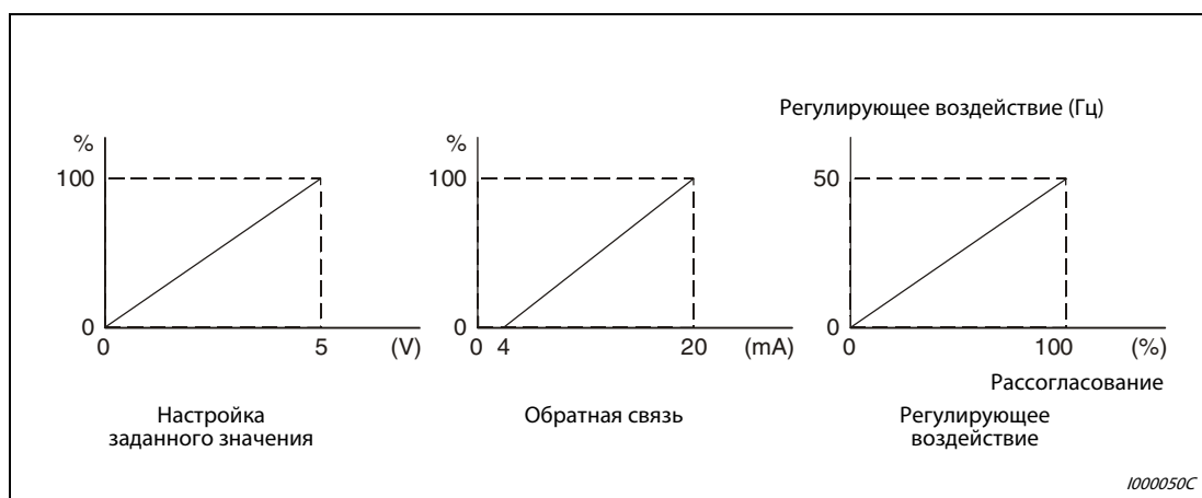
Рис. 6-142: Калибровка входов
