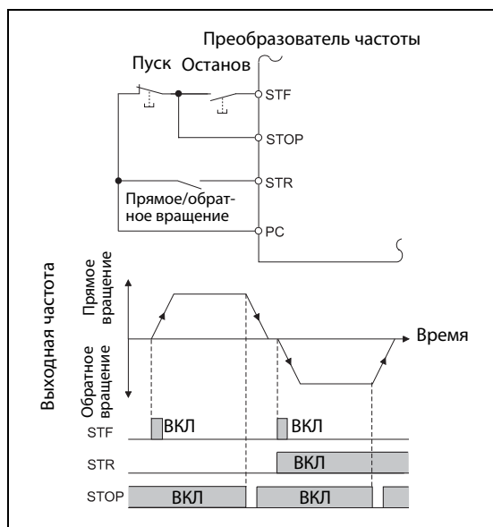
Рис. 6-58: Управление по 3-жильному проводу цепи управления (парам. 250=8888)
