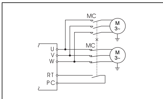
Рис. 6-37: Питание двух двигателей от одного преобразователя частоты
