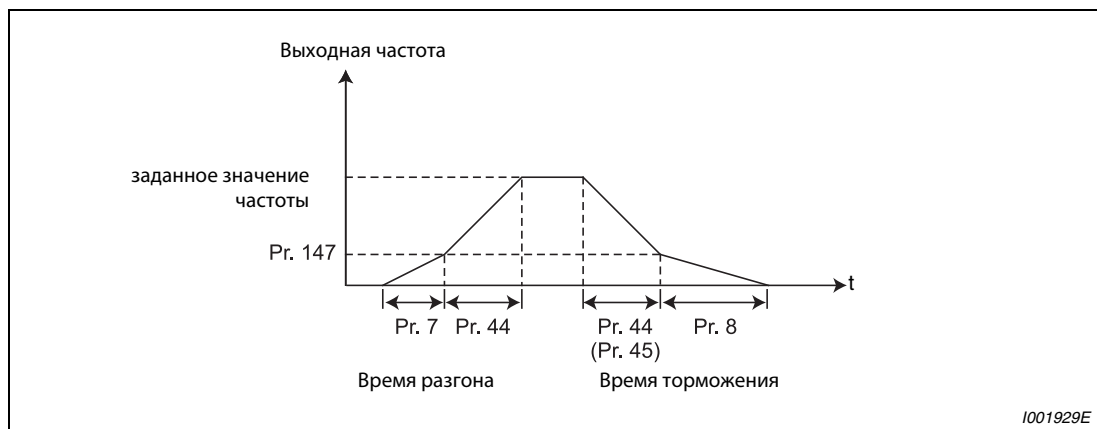
Рис. 6-30: Автоматическое переключение времени разгона/торможения
