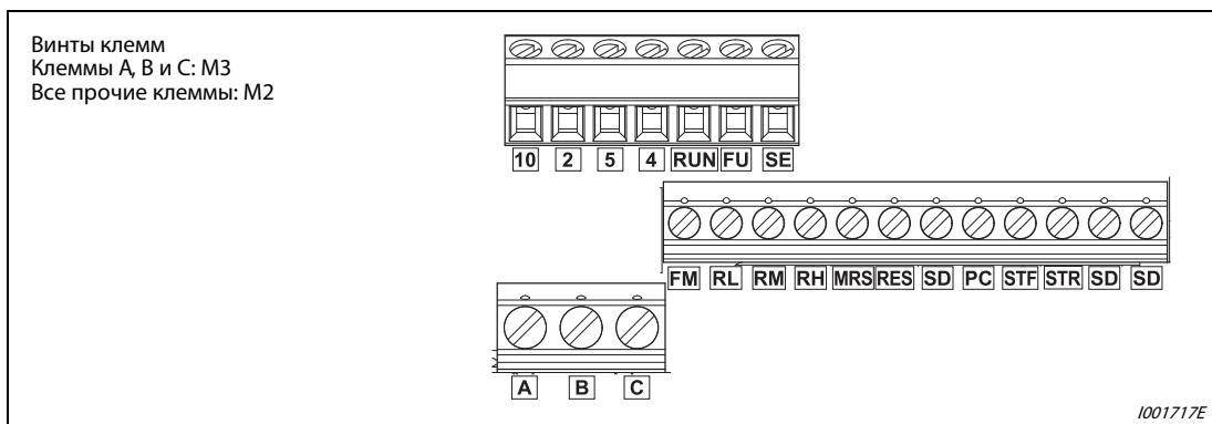
Рис. 3-6: Расположение клемм
