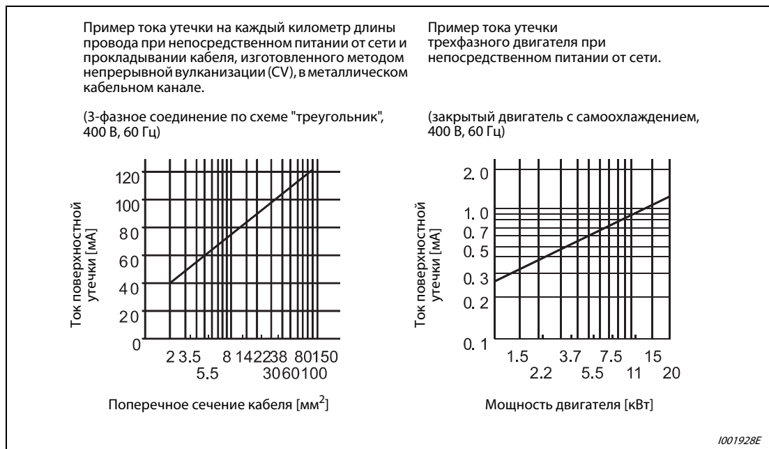
Рис. 3-29: Токи утечки
