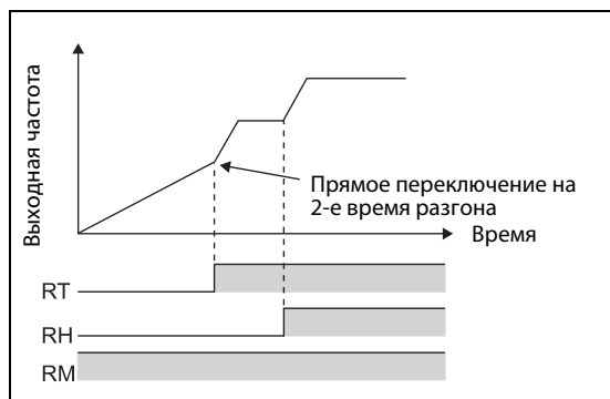
Рис. 6-54: Пример переключения времени разгона/торможения
