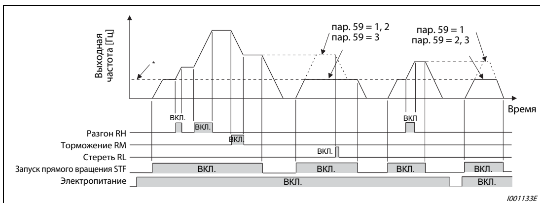
Рис. 6-26: Пример работы цифрового потенциометра
