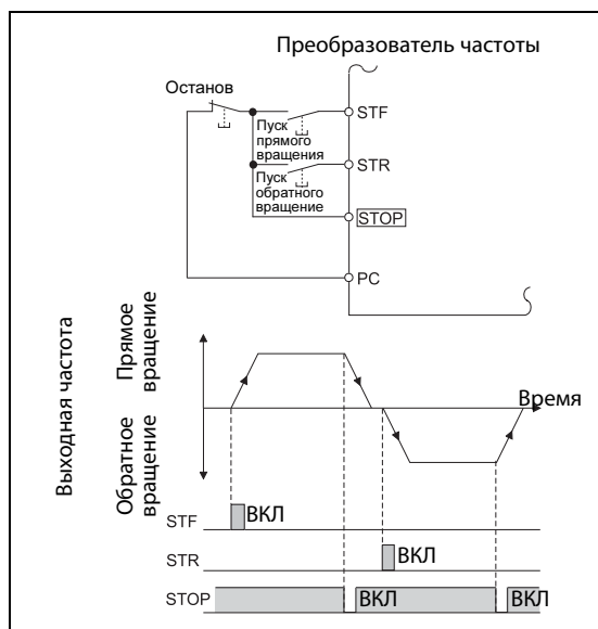
Рис. 6-57: Управление по 3-жильному проводу цепи управления (парам. 250 = 9999)
