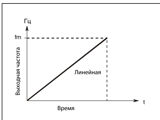
Рис. 6-33: Характеристика при парам. 29 = "0"
