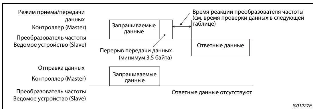
Рис. 6-128: Формат сообщений
