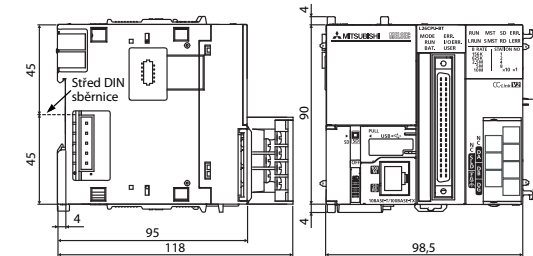
Rozměry: mm
