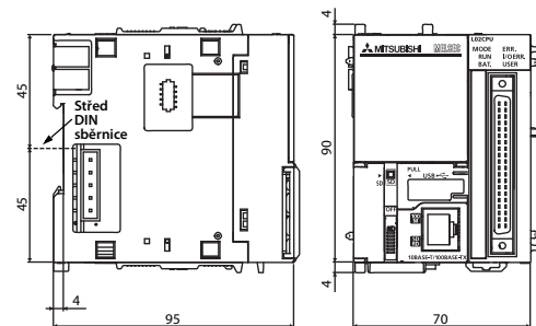
Rozměry: mm
