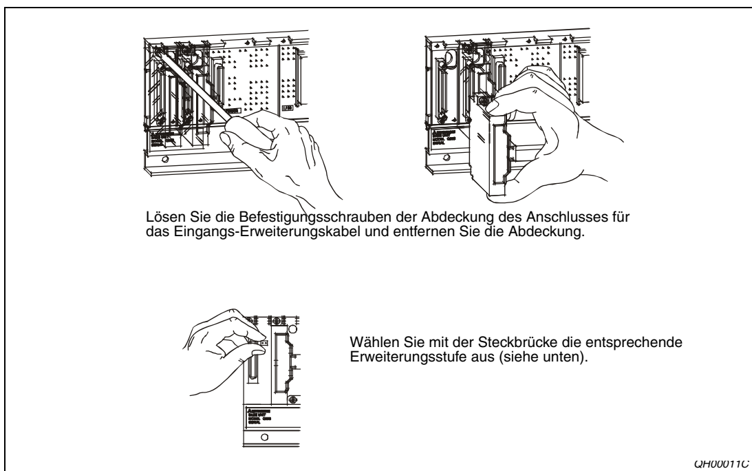
Abb. 8-6: Einstellung der Erweiterungsstufe
