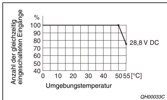
Abb. 12-13: Gleichzeitig schaltbare Eingänge beim Ein-/Ausgangsmodul QH42P
