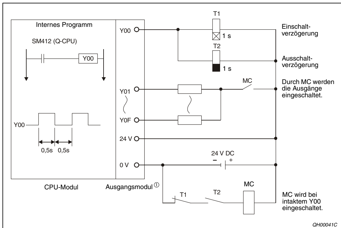
Abb. 9-3: Sicherheitsschaltung
