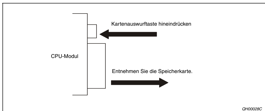
Abb. 5-3: Ausbau der Speicherkarte
