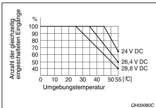
Abb. 12-9: Gleichzeitig schaltbare Eingänge beim Digital-Eingangsmodul QX82
