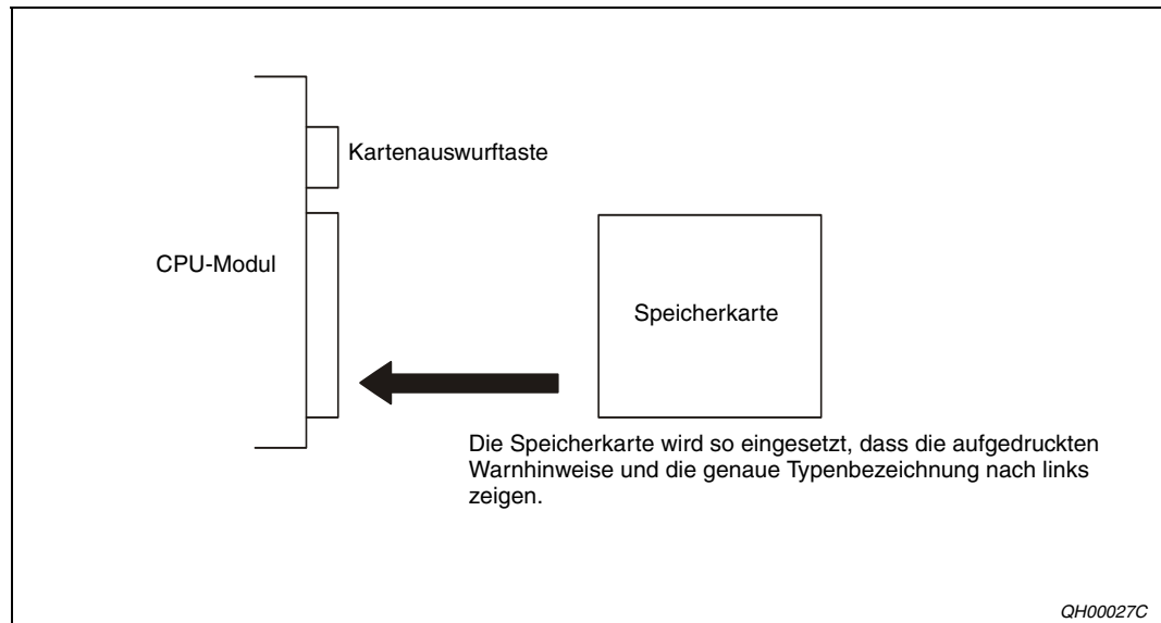
Abb. 5-2: Einbau der Speicherkarte
