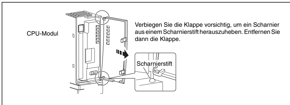
Abb. 5-4: Entfernen der Klappe
