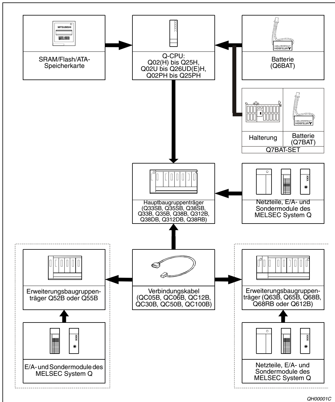
Abb. 3-3: Systemkonfiguration für die CPUs Q02(H) bis Q25H, die Universal-CPU's Q02U bis Q26UD(E)H und die Prozess-CPU's Q02PH bis Q25PH
