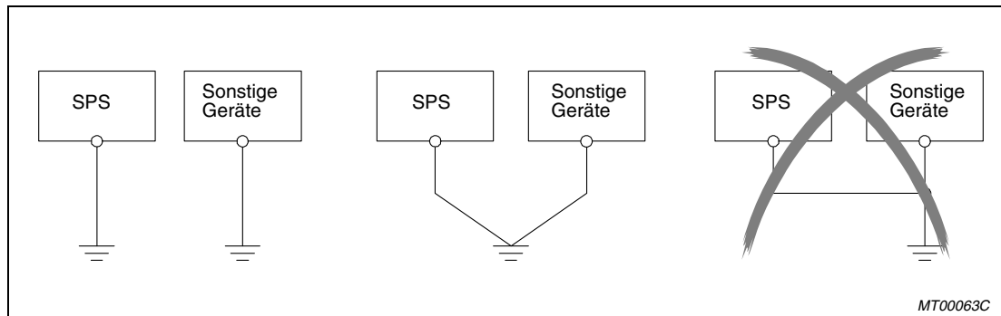
Abb. 9-21: Erdungsanschluss
