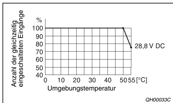
Abb. 12-8: Gleichzeitig schaltbare Eingänge beim Digital-Eingangsmodul QX81
