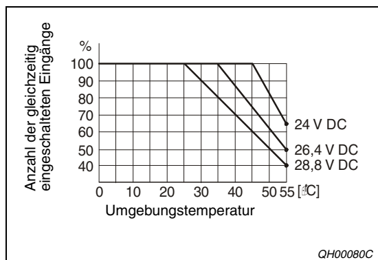
Abb. 12-6: Gleichzeitig schaltbare Eingänge beim Digital-Eingangsmodul QX42
