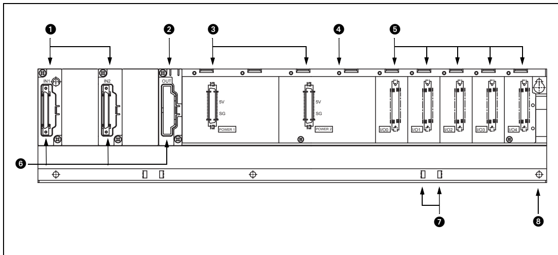
Abb. 8-5: Erweiterungsbaugruppenträger Q65WRB
