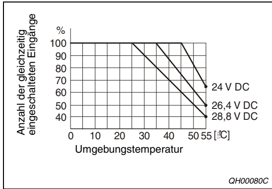
Abb. 12-7: Gleichzeitig schaltbare Eingänge beim Digital-Eingangsmodul QX42-S1
