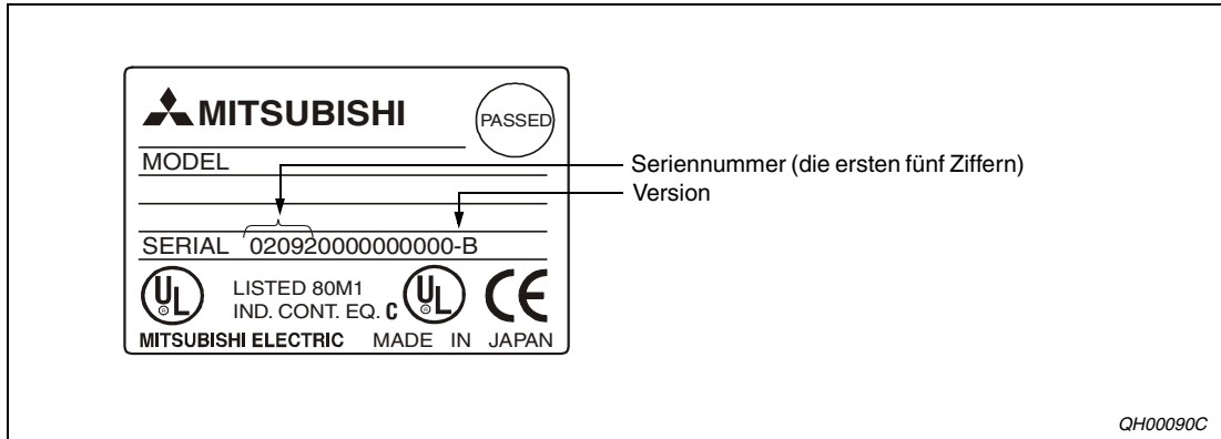
Abb. 4-11: Typenschild einer CPU des System Q
