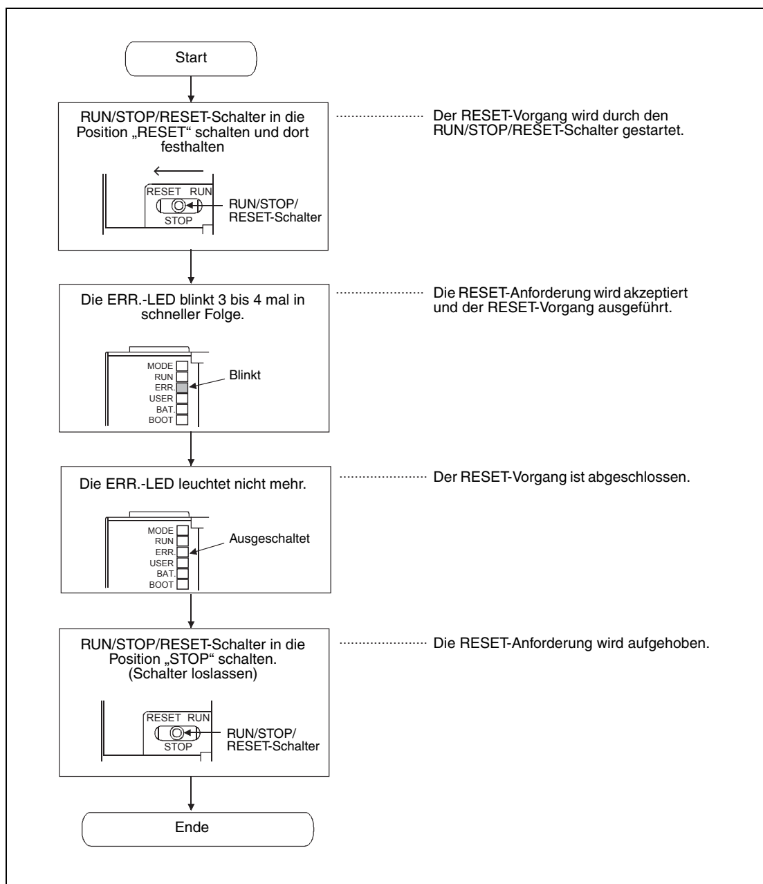
Abb. 4-10: RESET an einer Universal-SPS-CPU
