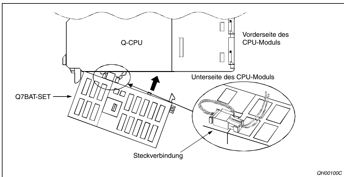
Abb. 5-12: Montage der Batterie Q7BAT
