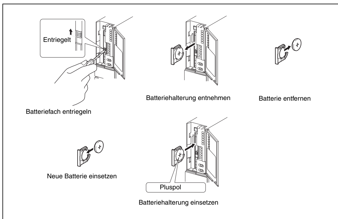
Abb. 10-6: Wechsel der Batterie der Speicherkarten Q2MEM-1MBS und Q2MEM-2MBS
