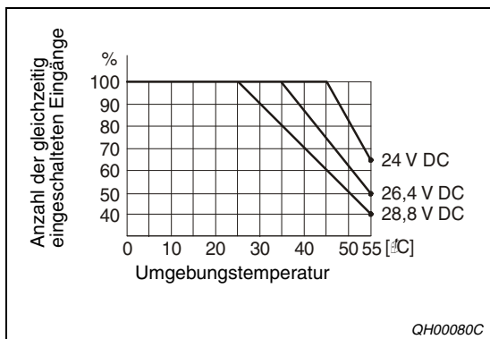
Abb. 12-10: Gleichzeitig schaltbare Eingänge beim Digital-Eingangsmodul QX82-S1
