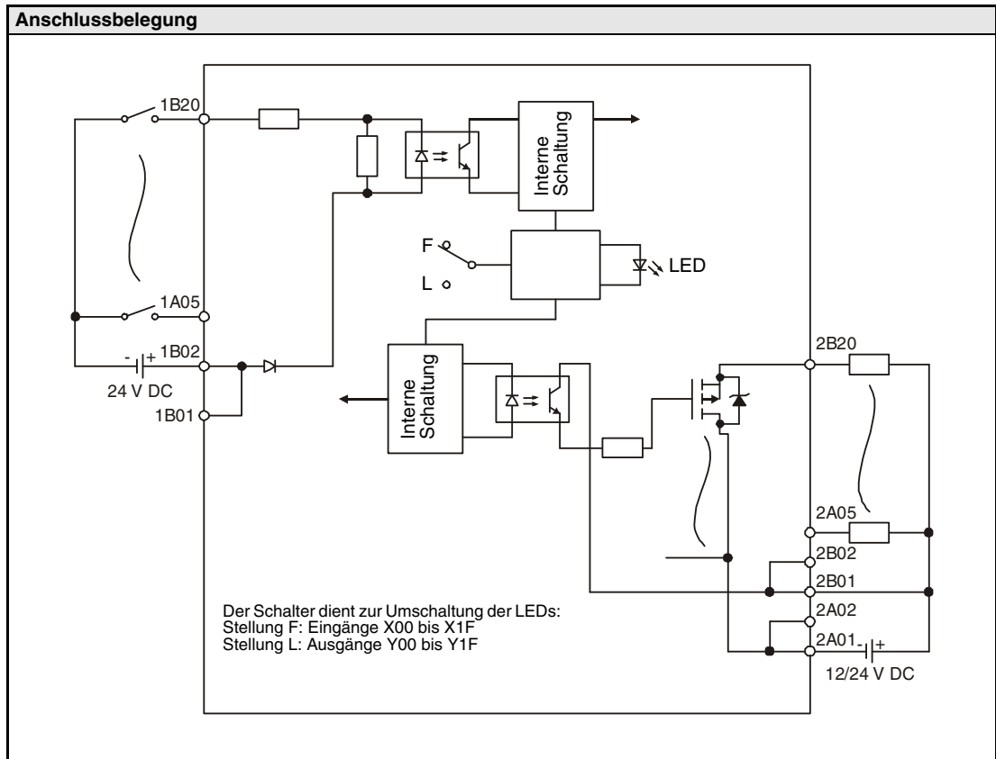
Abb. 12-12: Anschlussbelegung und interne Schaltung des Ein-/Ausgangsmoduls QH42P
