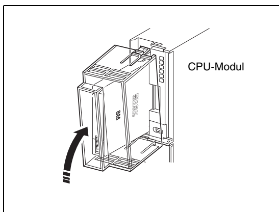
Abb. 5-6: Die Abdeckung schützt die aus dem CPU-Gehäuse herausstehende ATA-Speicherkarte.
