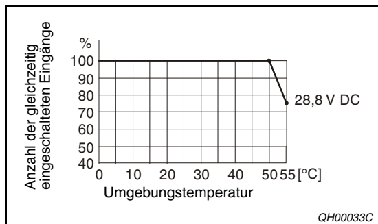
Abb. 12-4: Gleichzeitig schaltbare Eingänge beim Digital-Eingangsmodul QX41
