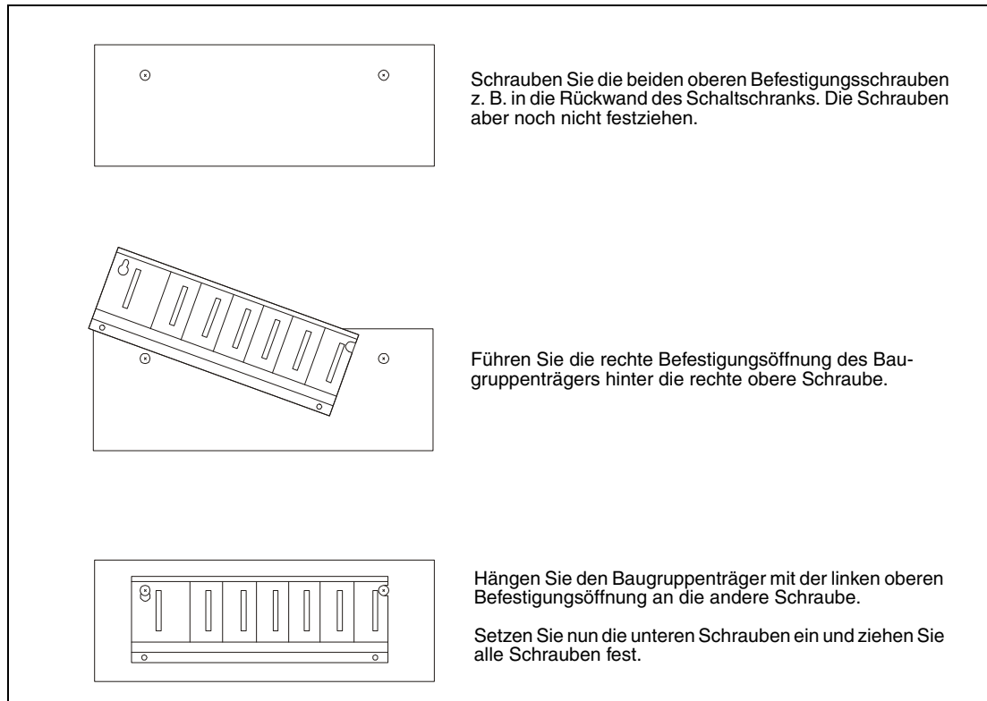
Abb. 9-9: Schritte bei der direkten Montage eines Baugruppenträgers oder einer Q00U(J)CPU
