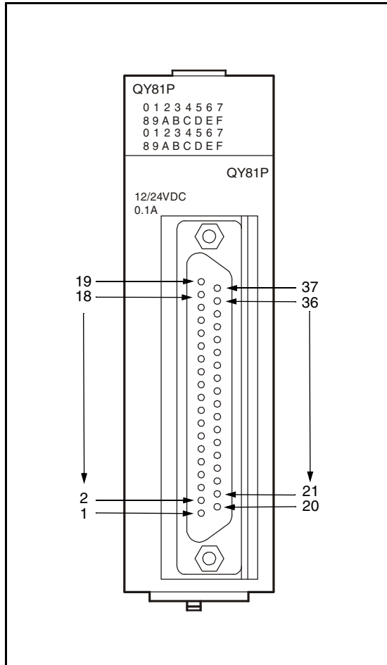
Abb. 12-11: PIN-Anordnung des 37-poligen D-Sub-Steckers des Ausgangsmoduls QY81P
