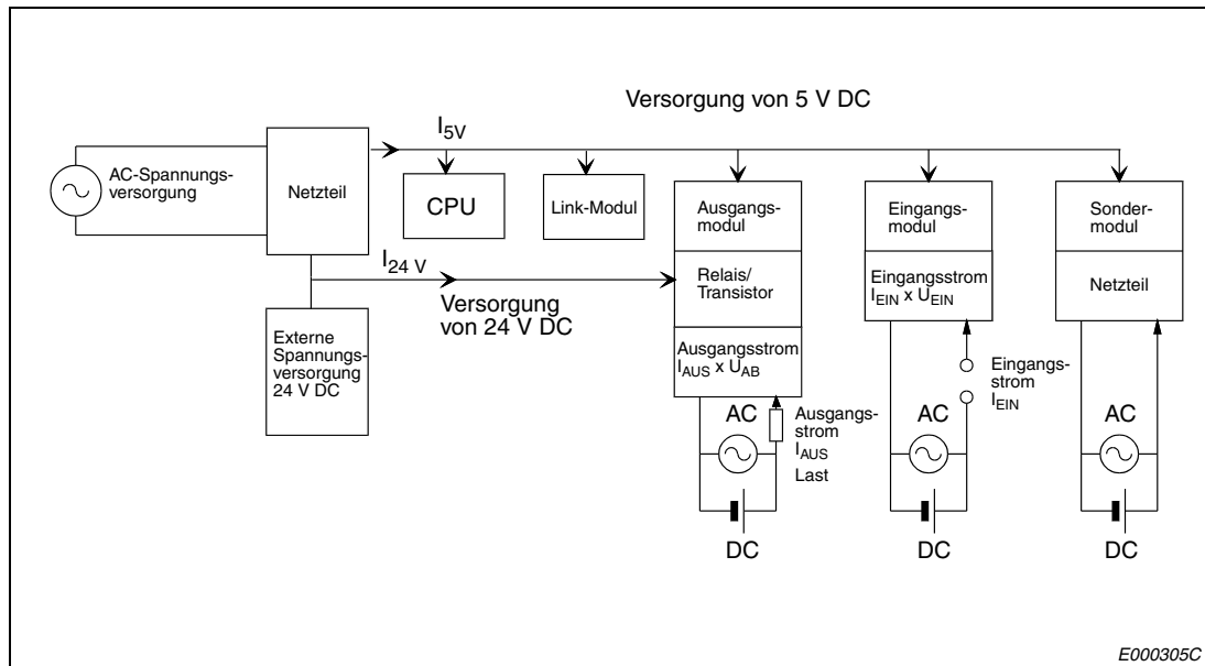
Abb. 9-4: Ermittlung der Stromaufnahme
