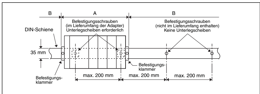
Abb. 9-11: Befestigung der DIN-Schiene bei einer Q00JCPU oder Q00UJCPU sowie den Baugruppenträgern Q33B, Q35B, Q65B, Q52B, Q55B, Q63B, Q32SB, Q33SB und Q35SB
