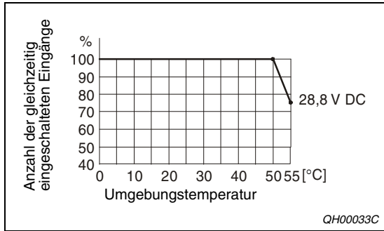
Abb. 12-5: Gleichzeitig schaltbare Eingänge beim Digital-Eingangsmodul QX41-S1
