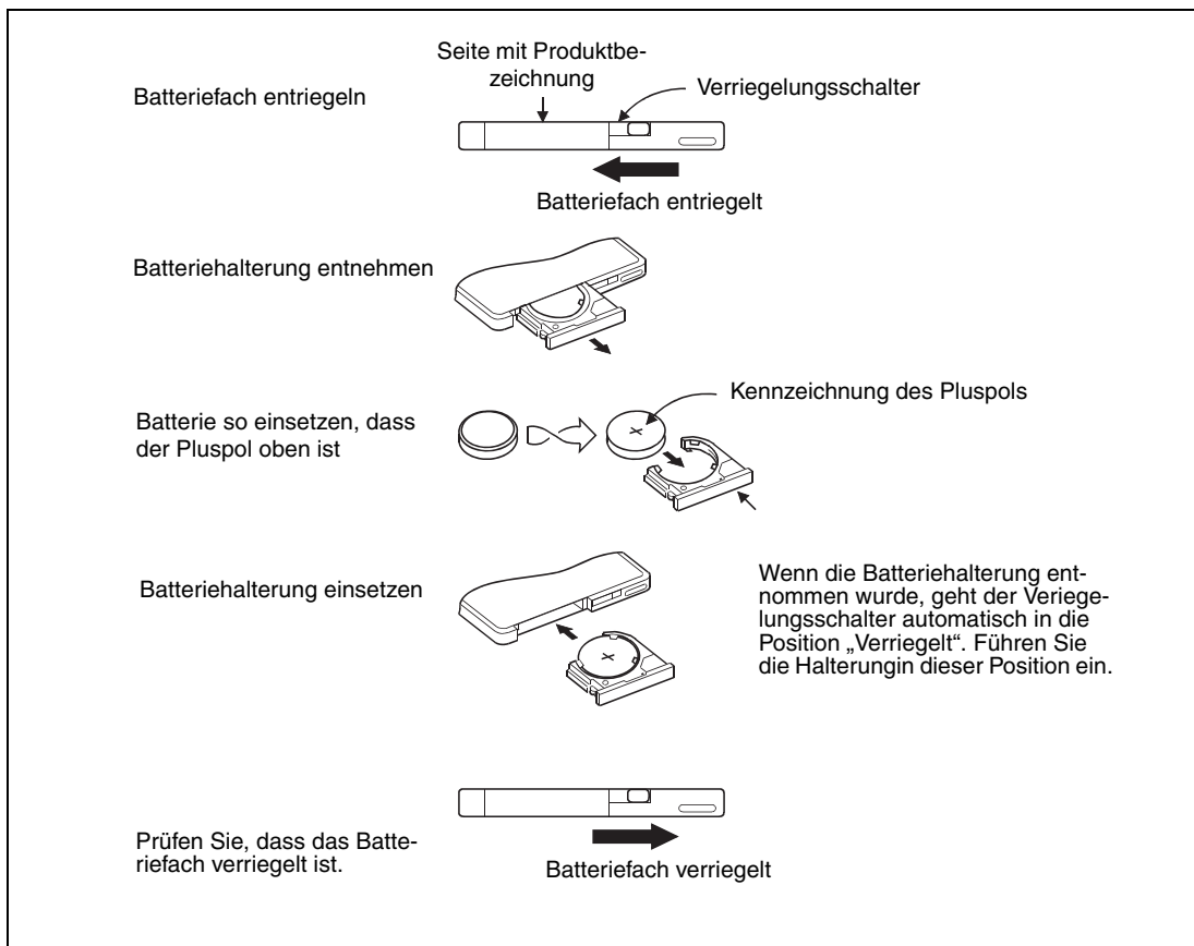
Abb. 5-13: Einbau der Batterie in die Speicherkarten Q2MEM-□□□
