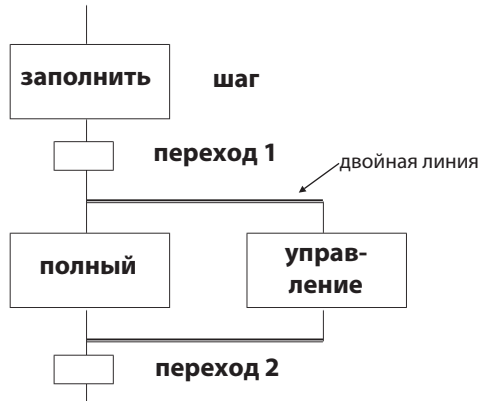
Параллельное ветвление
