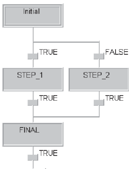
Пример последовательной функциональной схемы
