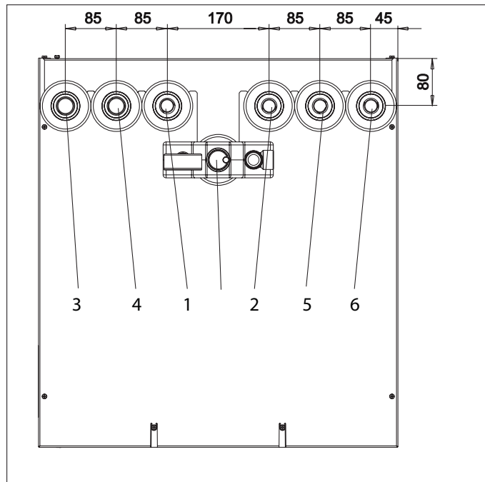
Подключение гидро модуля (вид сверху)
